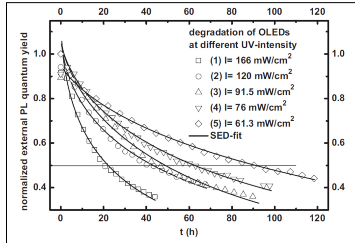
Figure 3.6 Dégradation des OLED bleus à différentes intensités d'UV
