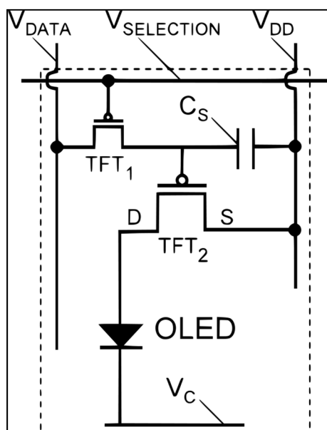
Figure 1.3 Exemple d'un circuit TFT pour une OLED Tirée d'Armael (2010)
