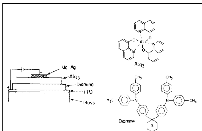
Figure 1.1 Configuration d'une OLED et structures moléculaires Tirée de Tang et VanSlyke (1987, p. 913) 1
