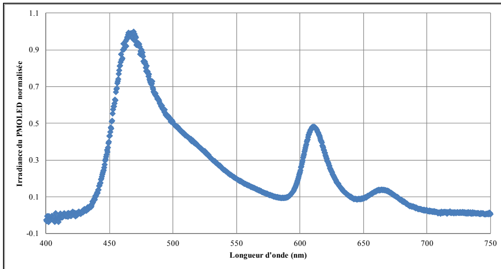
Figure 4.11 Spectre optique normalisé de l'écran PMOLED
