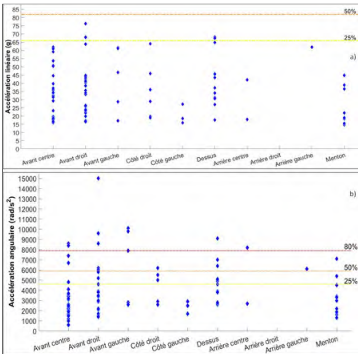
Figure 4.10 Accélérations des techniques de tête en fonction du mouvement de la tête des joueurs : a) linéaires (g) et b) angulaires ( \text{rad/s}^2 )
