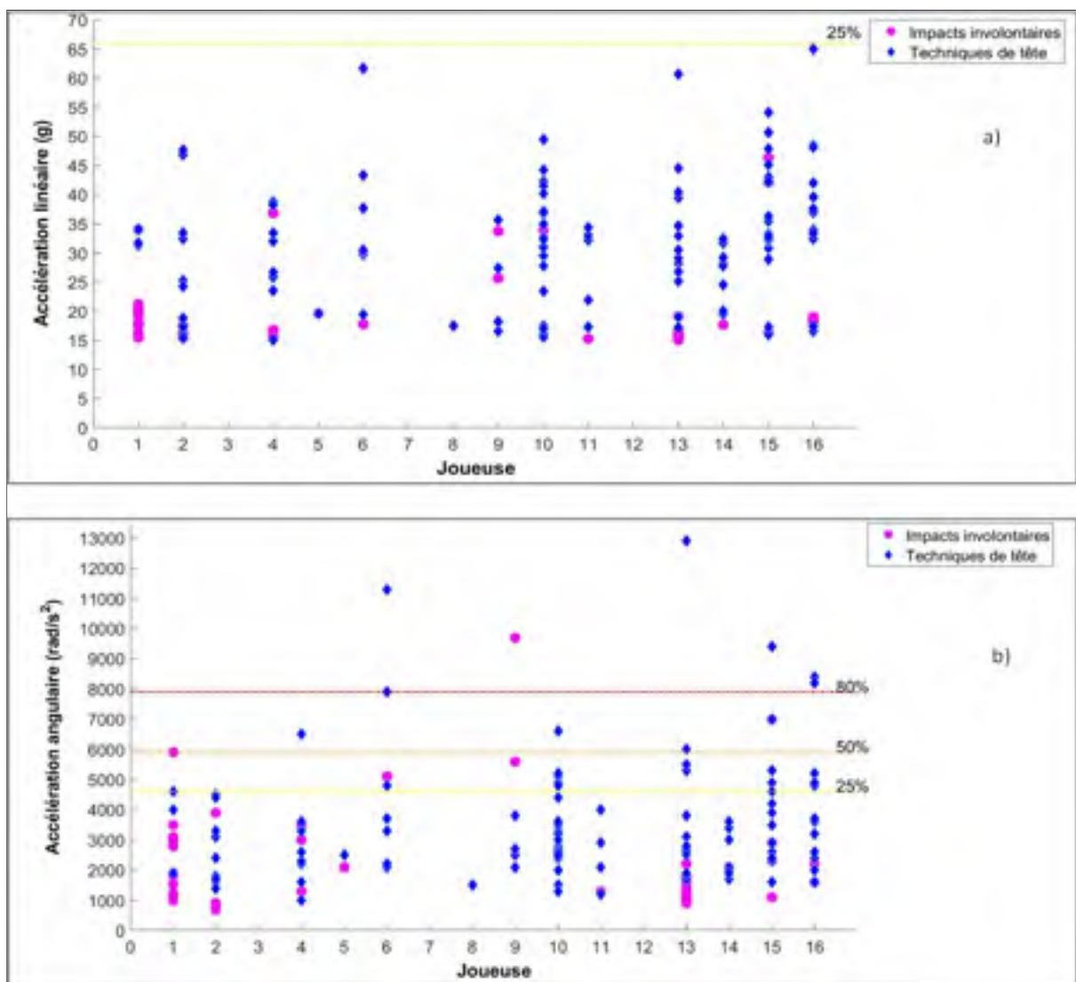
Figure 4.13 Accélérations des techniques de tête et des impacts involontaires des joueuses lors des matches de compétition de la saison d'automne : a) linéaires (g) et b) angulaires ( \text{rad/s}^2 )
