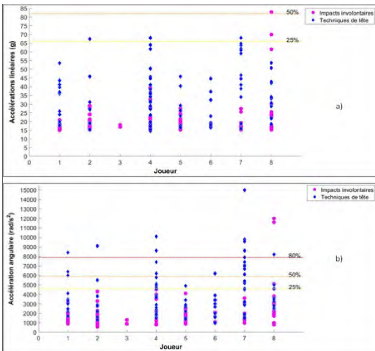
Figure 4.2 Accélérations des techniques de tête et des impacts involontaires de la tête des joueurs lors des matchs de compétition : a) linéaires (g) et b) angulaires ( \text{rad/s}^2 )
