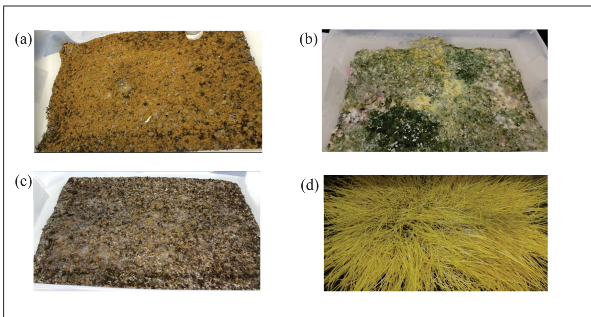
Figure 3.7 Croissance observée après 21 jours de traitement pour (a) seigle stérilisé, (b) tourteau de soja stérilisé, (c) seigle non stérilisé et (d) tourteau de soja non stérilisé
