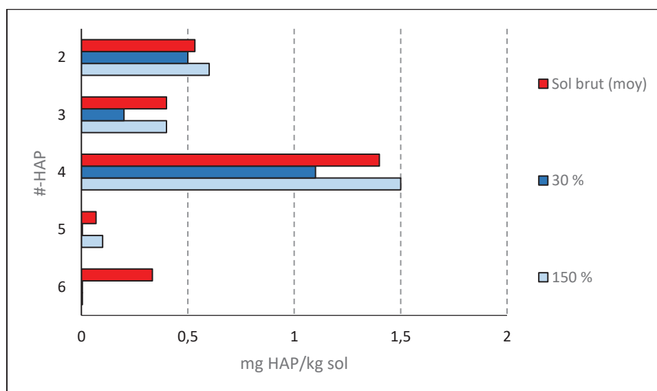
Figure 3.10 Comparaison du taux de contamination de sol traité par P. ostreatus avec différents teneurs en humidité
