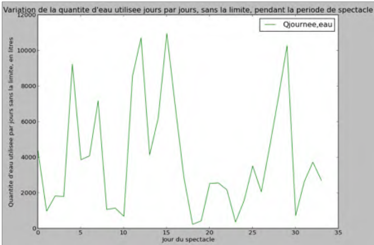
Figure 4.4 Tracé de V_{\text{day,eau}} pour chacun des jours de spectacles sans limite d'eau
