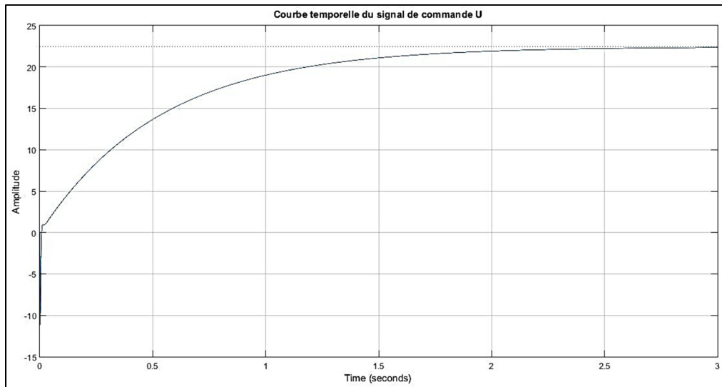
Figure 5-30 Courbe temporelle du signal de commande pour \varepsilon=0.2 , M=1.01 , \gamma=1.01
