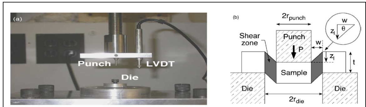
Figure 2.5 (a) dispositif expérimental du shear punch test et (b) schéma de principe du shear punch test (Guduru et al. 2005)
