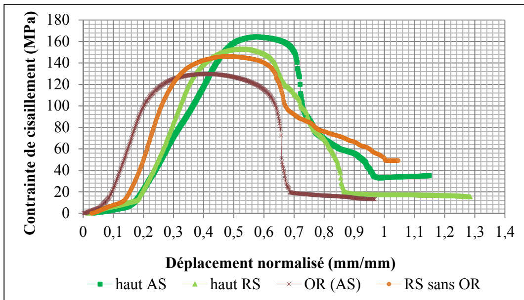
Figure 3.38 Courbes de la contrainte de cisaillement en fonction du déplacement normalisé de l'échantillon 823SS1
