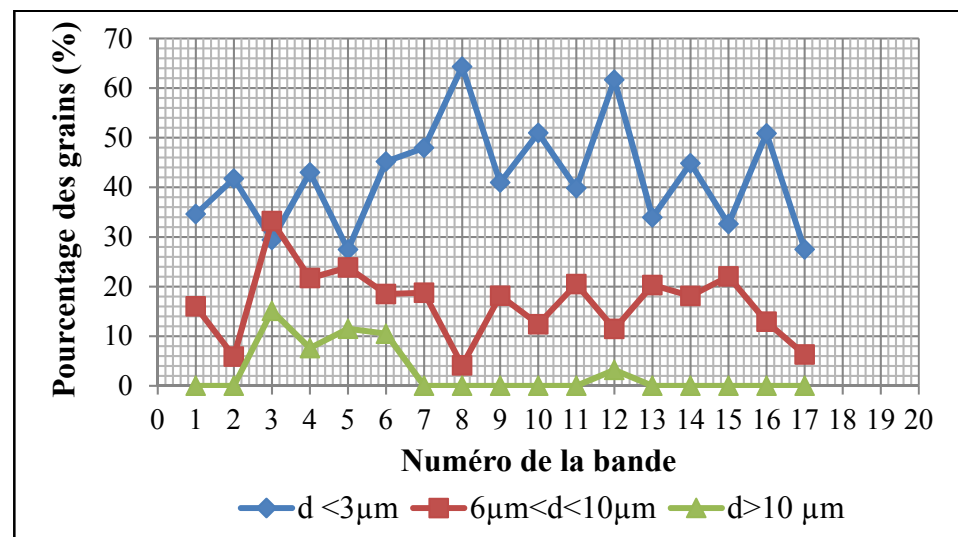
Figure 3.6 Pourcentage des grains dont le diamètre est <3 \mu m , entre 6 et 10 \mu m et >10 \mu m
