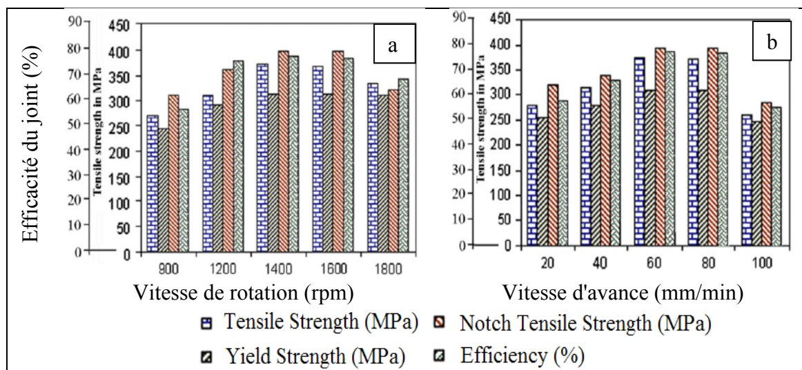
Figure 1.14 Résistance à la traction, limite d'écoulement et l'efficacité du joint correspondante pour l'alliage 7075-T6 en variant en (a) la vitesse de rotation et en (b) la vitesse d'avance (Rajakumar, Muralidharan, and Balasubramanian 2011)
