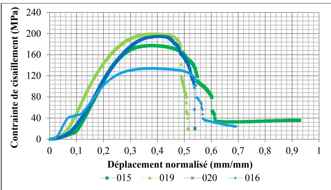
Figure 3.31 Courbes de la contraite de cisaillement en fonction du déplacement normalisé dans le haut de la soudure côté RS des quatre échantillons
