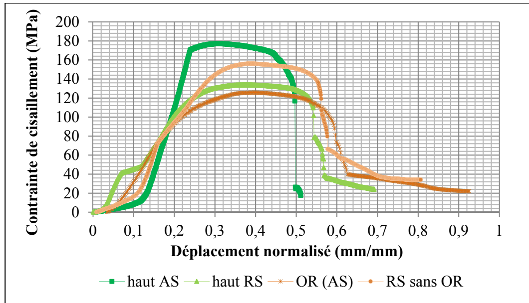
Figure 3.37 Courbes de la contrainte de cisaillement en fonction du déplacement normalisé de l'échantillon 016
