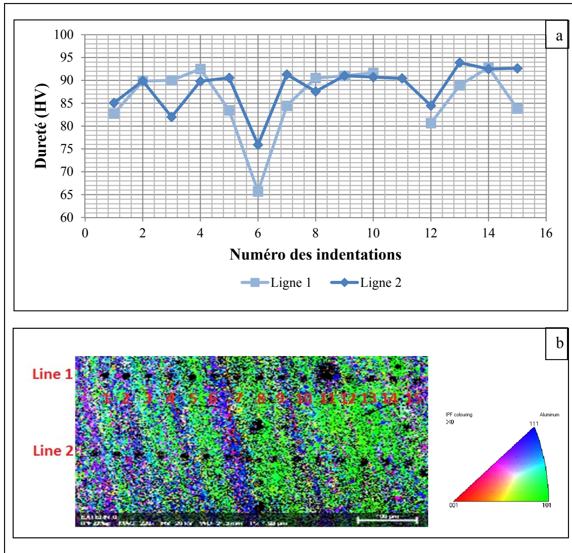
Figure 3.9 (a) Profil de dureté mesurée par des nano-indenteurs correspondant aux deux lignes de mesure sur la carte EBSD en (b)
