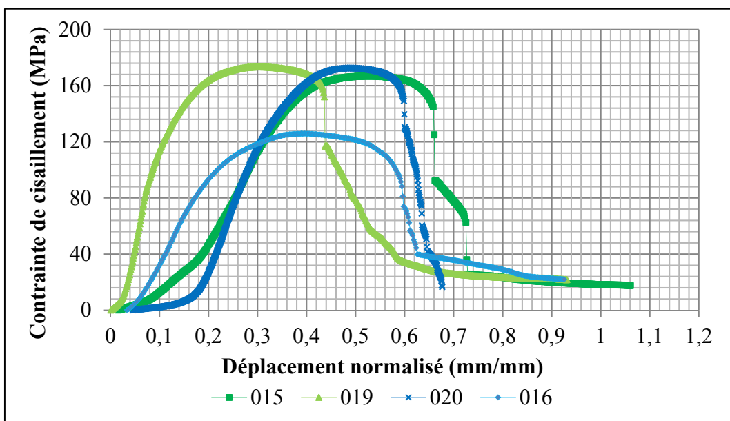
Figure 3.32 Courbes de la contraite de cisaillement en fonction du déplacement normalisé dans le bas de la soudure du côté AS avec présence des bandes alternées des quatre échantillons
