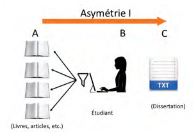
Figure 1.2 Diagramme de couverture pour plusieurs références et une seule projection.
