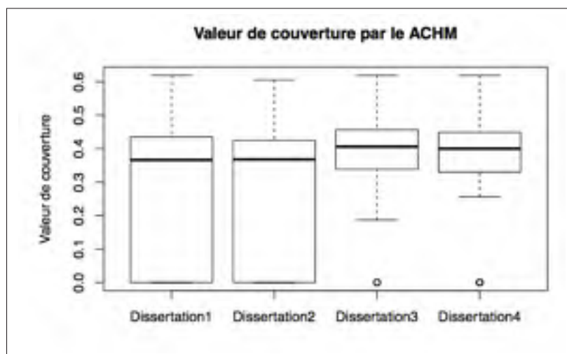
Figure 4.6 Distribution des valeurs de couverture des dissertations avec le ACHM.
