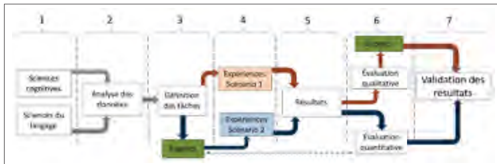
Figure 3.1 Étape présidant à notre choix méthodologique.
