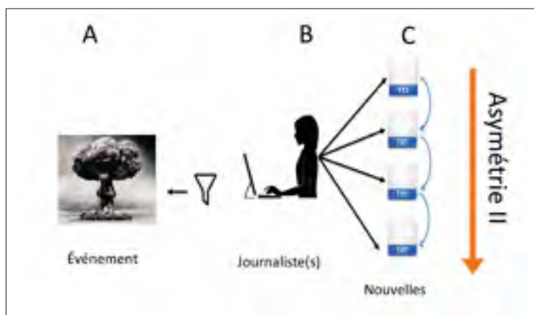
Figure 2.3 Diagramme de couverture scénario 2 (reprise de la fig. 1.3).
