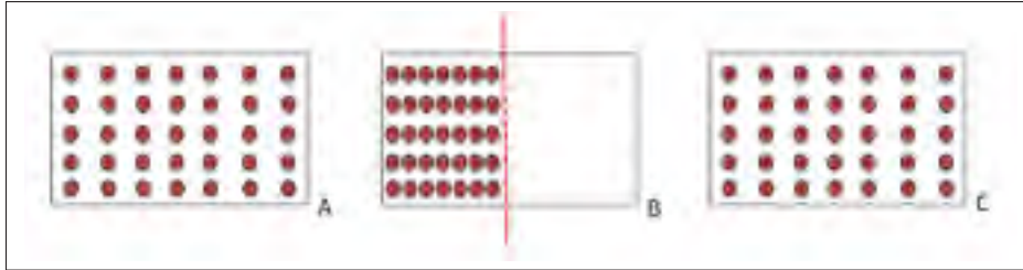
Figure 1.5 Reproduction du diagramme d'un réservoir de gaz en trois temps, A, B, et C. Exemple tiré de Leyton (1992, p. 8).
