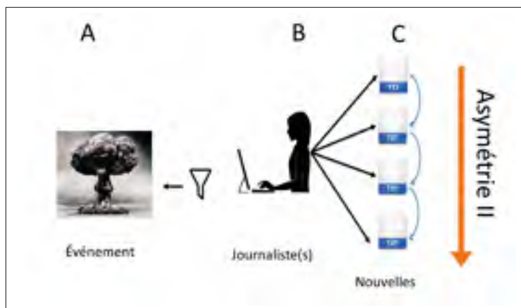
Figure 1.3 Diagramme de couverture pour une référence et plusieurs projections.
