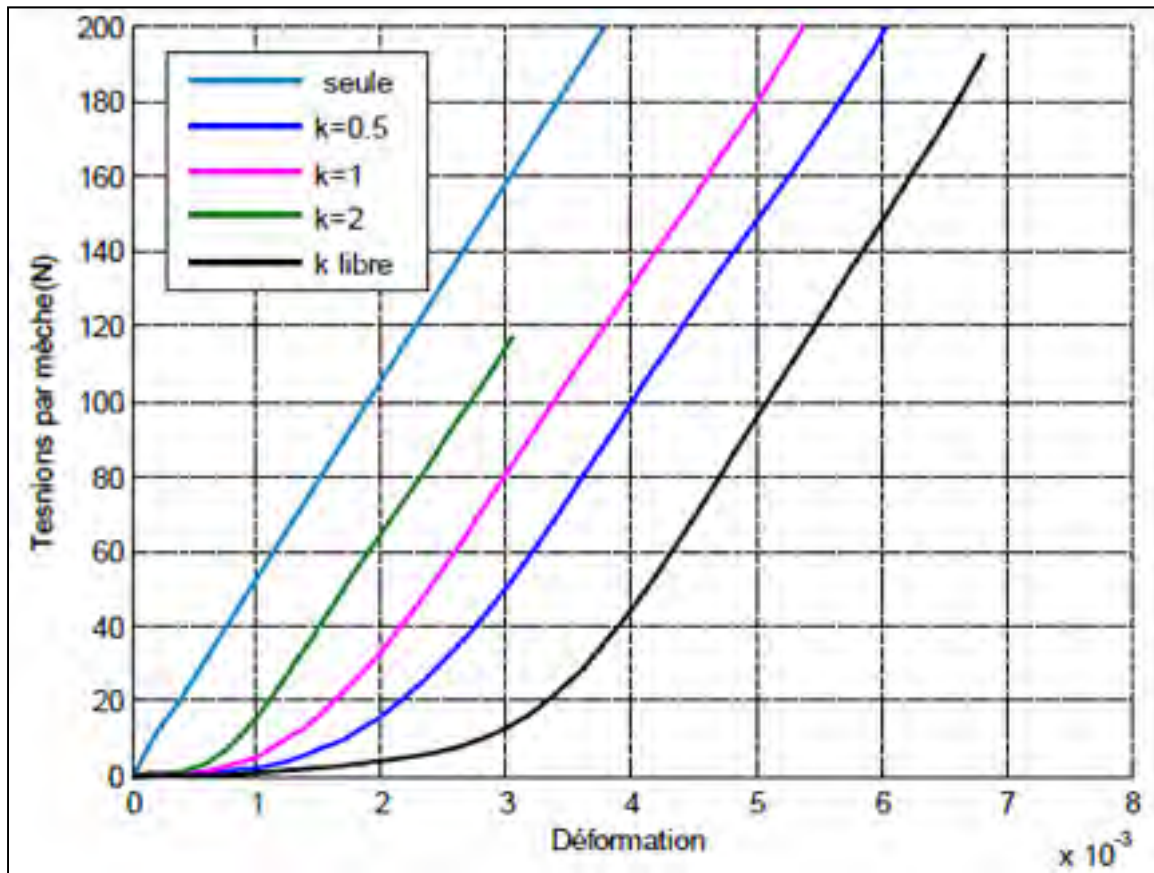
Figure 2.7 Comportement en tension bi-axiale d'un sergé 2 X 2 de carbone (Boisse, 2004).
