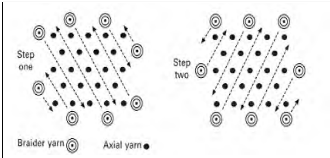
Figure 1.17 Schéma de fonctionnement du tissage 2-steps (Lomov, Verpoest et Robitaille, 2005)
