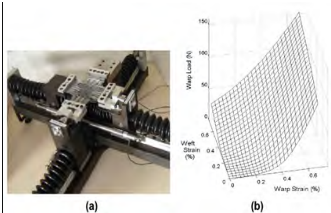
Figure 2.8 a) Montages de traction bi-axiale, b) surface caractéristique des résultats (Boisse et al., 2011 ; Quaglioni, Corazza et Poggi, 2008)
