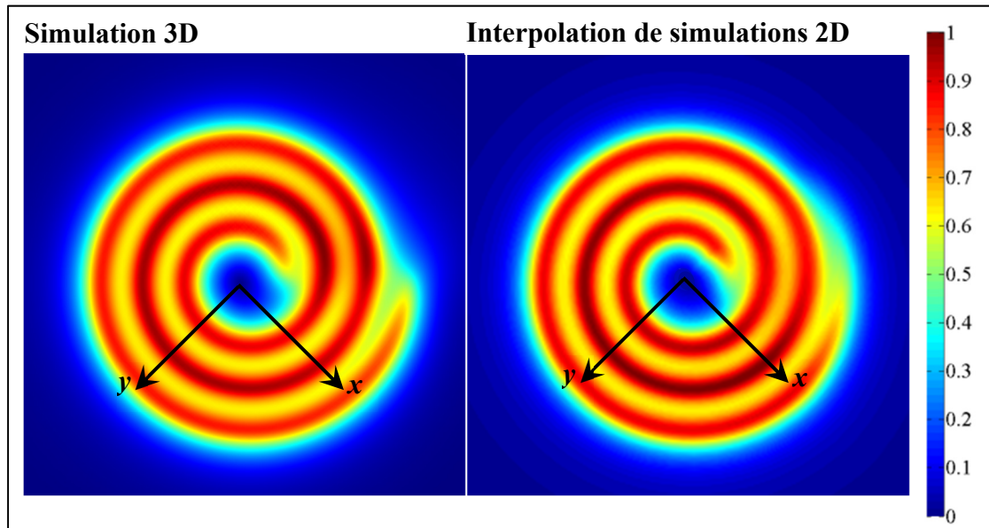
Figure A II-5 Comparaison de la distribution de densité de courant normalisée dans la plaque, obtenue avec une simulation 3D (gauche) et une interpolation de simulations 2D (droite)
