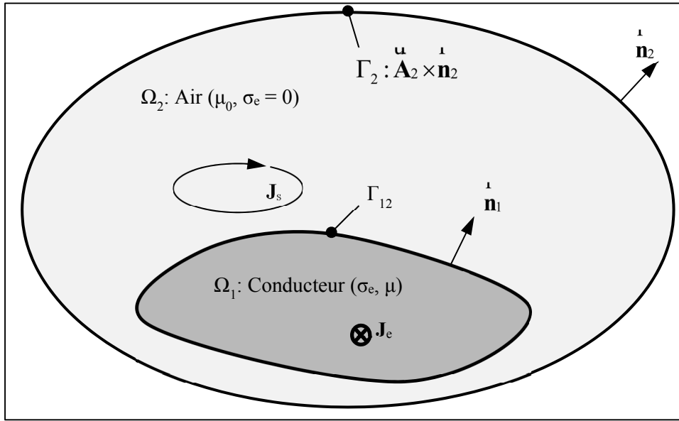
Figure 1.18 Représentation schématique du modèle électromagnétique
