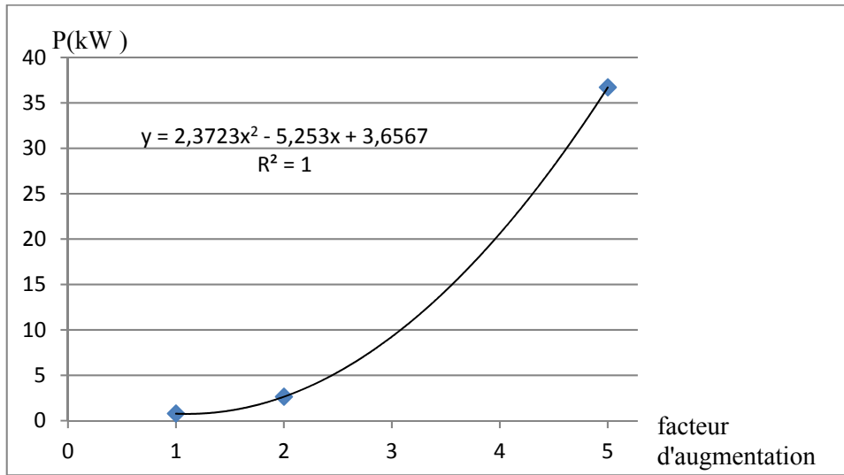
Figure 4.27 L'effet de la largeur de la pièce en forme L sur la puissance de chauffage
