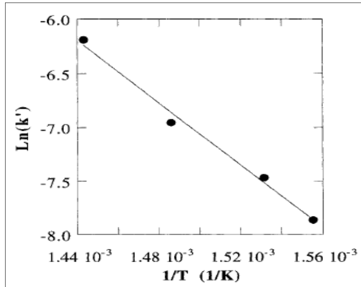
Figure 1.7 L'évolution de la vitesse de réaction \ln(k) en fonction de 1/T pour CF/PEEK tiré de Kessler (1997, p.504)
