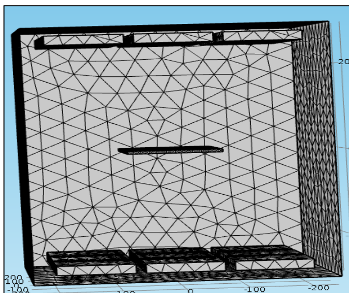
Figure 2.28 Le maillage la pièce concave dans le four
