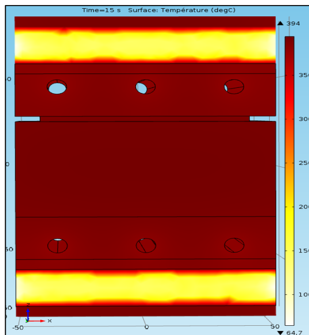
Figure 3.10 La répartition de la température dans le moule après 15s de refroidissement de la pièce en T
