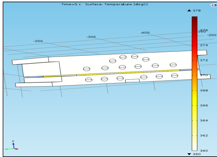
Figure 3.23 La répartition de la température dans le moule après 5s du contact de la pièce avec le moule
