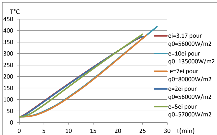
Figure 4.10 Comparaison des cycles de chauffage de la pièce en forme T pour 5 épaisseurs de la pièce
