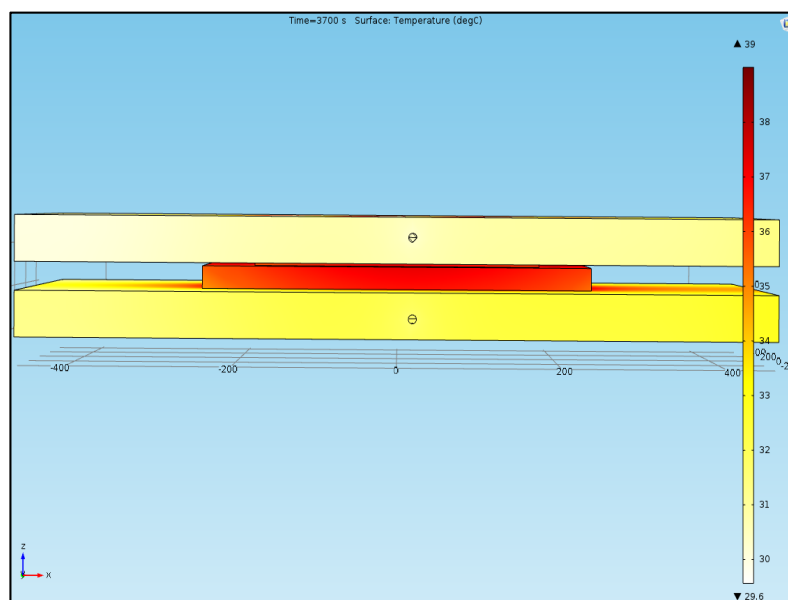
Figure 3.2 La répartition de la température dans le moule et la plaque après 3700s de refroidissement
