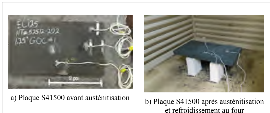
Figure 2-1: Austénitisation complète du matériau 13Cr-4Ni
