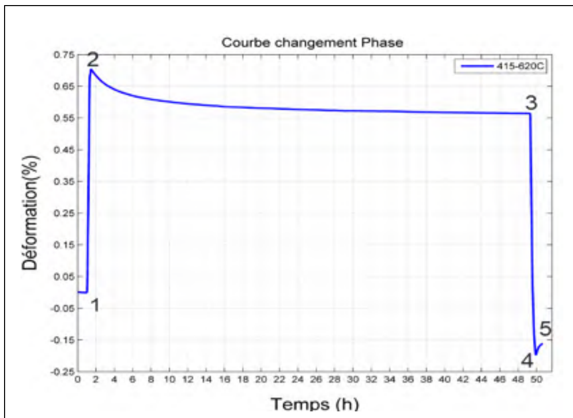
Figure 2-8 : Courbe dilatométrique à 620 °C pour 48 h de maintien suivi d'un refroidissement lent
