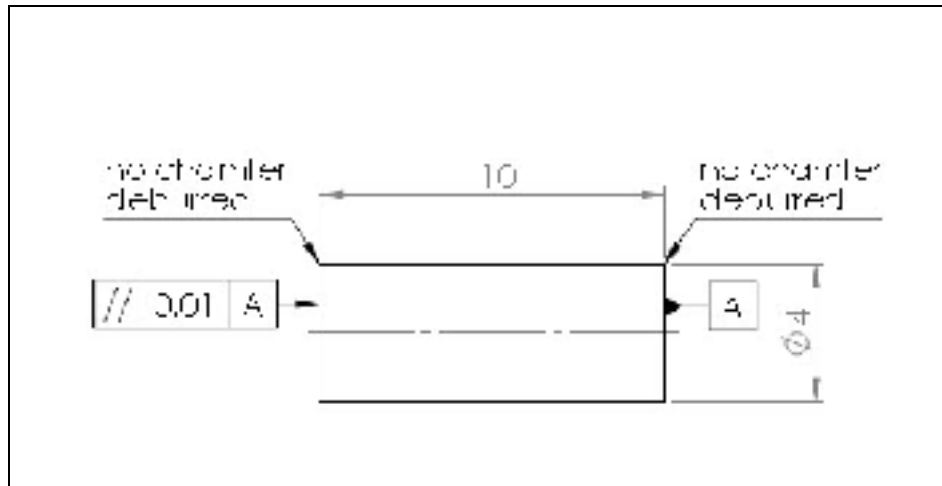
A II-1 : Plan technique éprouvette dilatométrique
