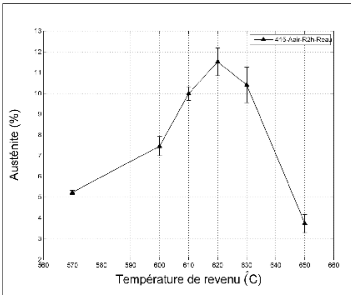
Figure 2-3 : Cloche d'austénite de réversion en fonction de la température de revenu pour 2 h
