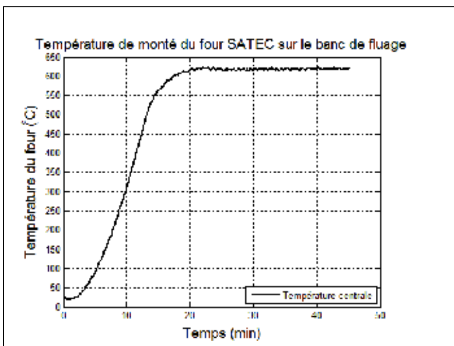
A IV-6 : Courbe de chauffage du four optimisée pour 620 °C
