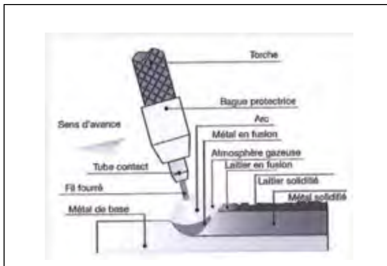
Figure 1-11 : Procédé de soudage par fil fourré (Tiré de http://www.weldx.com/procedes-soudage.html )
