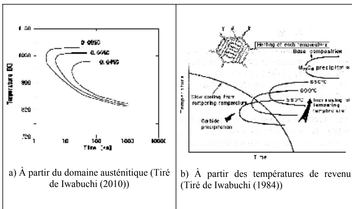
Figure 1-8 : Diagramme TTT indiquant l'influence de la teneur en carbone sur la cinétique de précipitation des carbures de chrome pour un acier de composition 13Cr-4Ni
