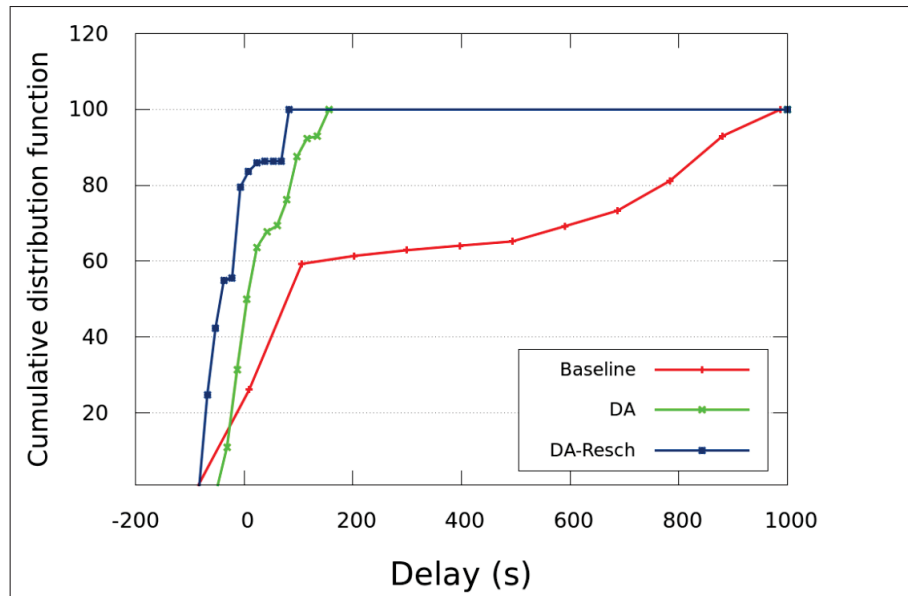
Figure 4.10 Fonction de répartition des retards - Scénario 1
