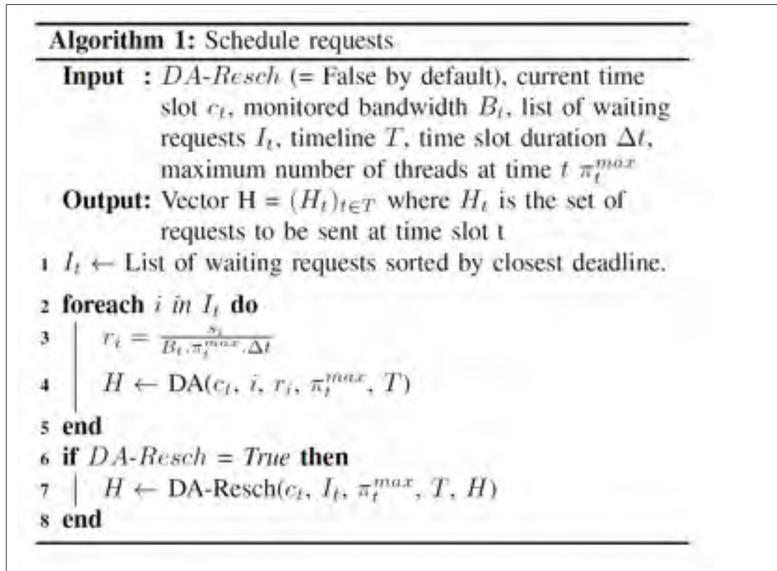
Figure 3.3 Algorithme d'ordonnement de requêtes.
