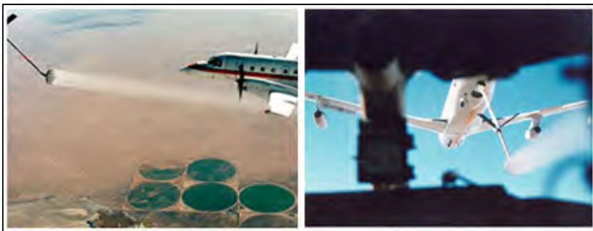
Figure 1.4 Vol d'essai grandeur nature avec buse givrante Tirée de FAA, 2016
