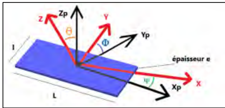
Figure 2.1 Définition de l'orientation de la plaque plane
