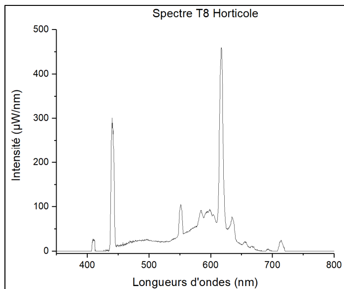
Figure 2.1 Réponse spectrale des T8-Horticole
