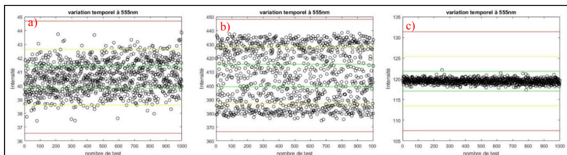
Figure 3.11 Comparaisons de l'uniformité temporelle pour le luminaire a) T8 horticole, b) T8 DEL, c) Multi-DEL
