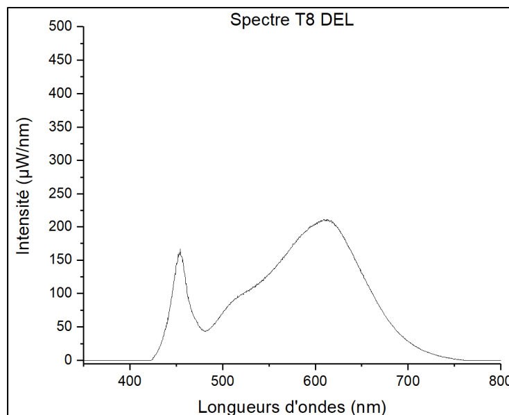
Figure 2.2 Réponse spectrale du T8-DEL
