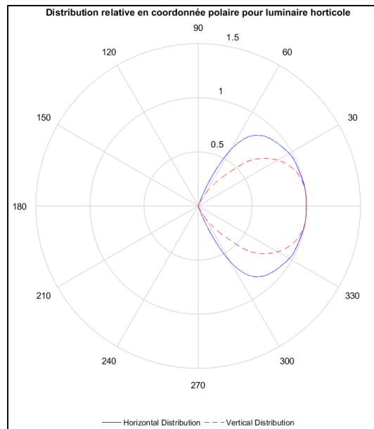
Figure 3.8 Angle de vue horizontal et vertical des T8 horticoles
