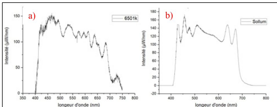
Figure 2.3 Comparaison du spectre initial versus le spectre utilisé pour les tests a) Spectre original D65 b) Spectre D65 modifié par ajout de bleu et rouge
