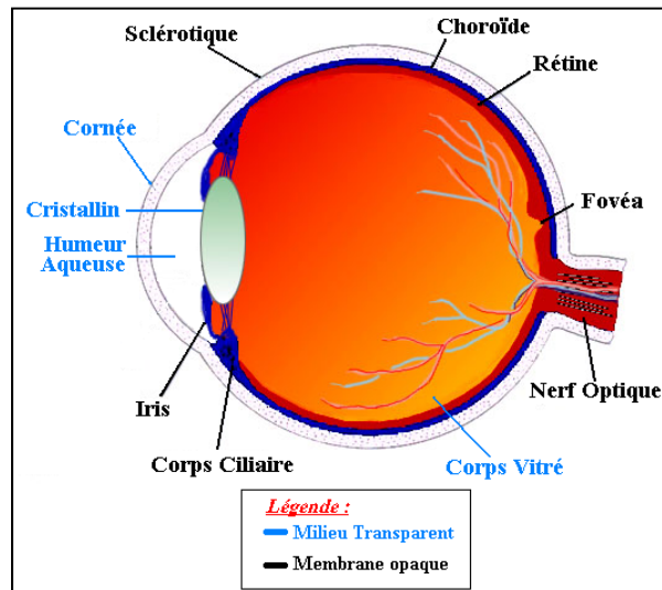
Figure 1.1 Anatomie de l'œil humain Tirée de Bioinformatics Organization (1998)
