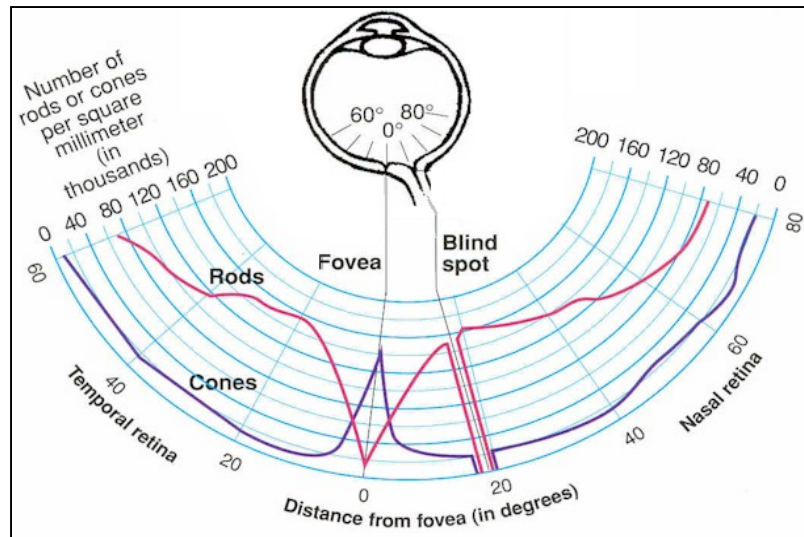
Figure 1.2 Positionnement et quantité des bâtonnets et des cônes dans l'œil humain Adaptée de Purves (2012)
