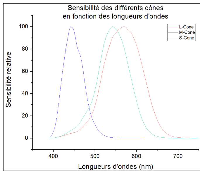
Figure 1.3 Comparaison entre les différents types de cônes Tirée de Stiles et Burch (1959)
