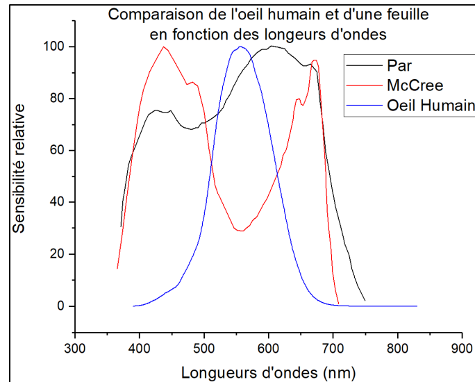
Figure 1.4 Comparaison de la sensibilité de l'œil humain et d'une feuille en fonction de la longueur d'onde
