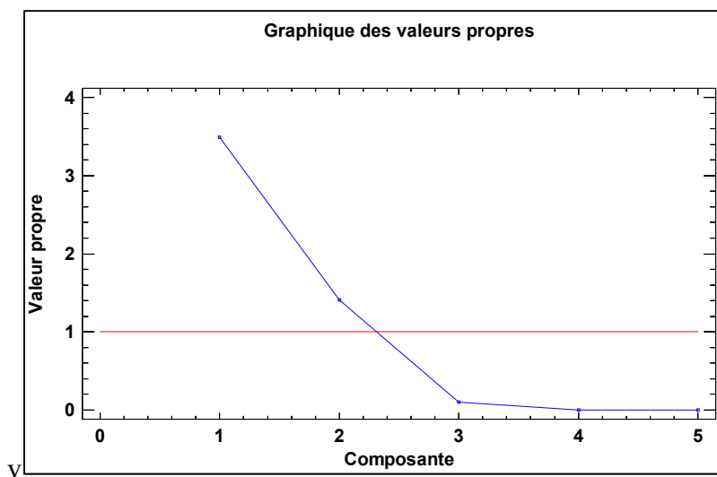
Figure 5.1 Résultats de l'analyse en composante principale
