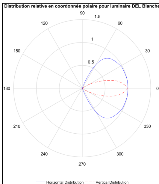
Figure 3.9 Angle de vue horizontal et verticale du luminaire à DEL blanches
