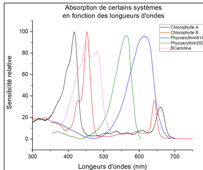
Figure 1.5 Spectre d'absorption de différents systèmes chez une plante
