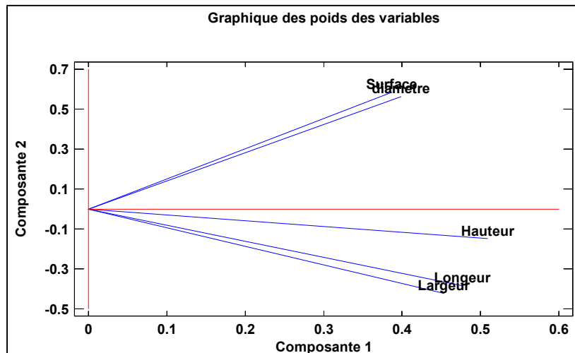
Figure 5.2 Résultats des poids des variables
