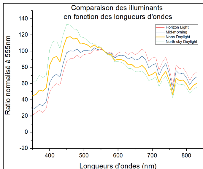
Figure 1.8 Comparaison des illuminants de type D Adaptée de Wyszecki et Stiles (2000)
