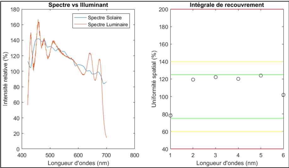
Figure 3.5 Intégrale de recouvrement spectral du luminaire multi-DEL 6500K
