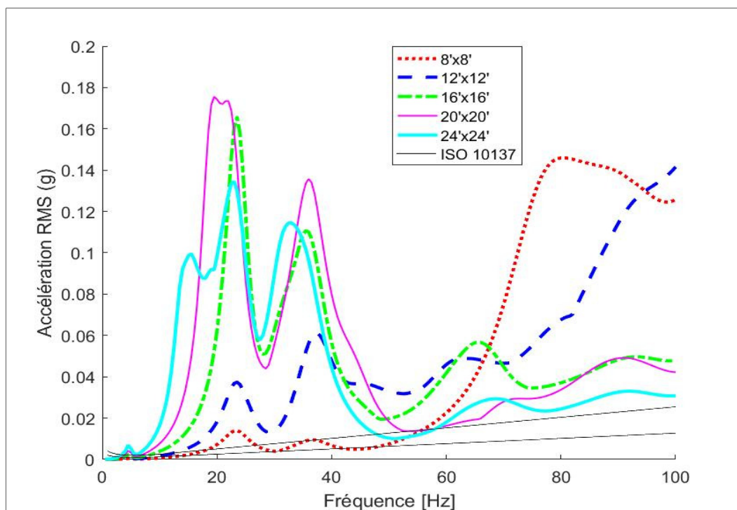
Figure 3.39 : Accélération efficace des planchers avec plateforme lourde et fauteuil décentré sur le côté et vers l'arrière
