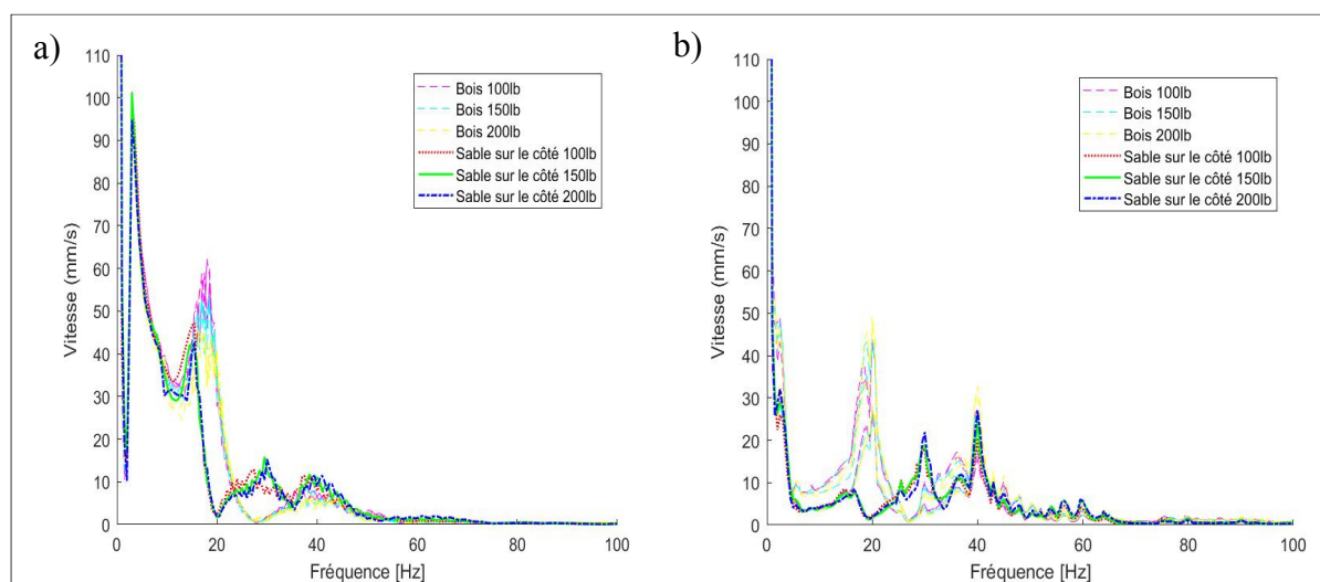
Figure 2.23 : Vibrations du fauteuil avec sable sur le côté lors de a) Balayage et b) Film
