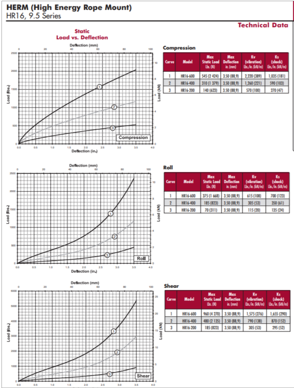
Figure-A V-1 : ITT Enidine Inc. HR16-600
