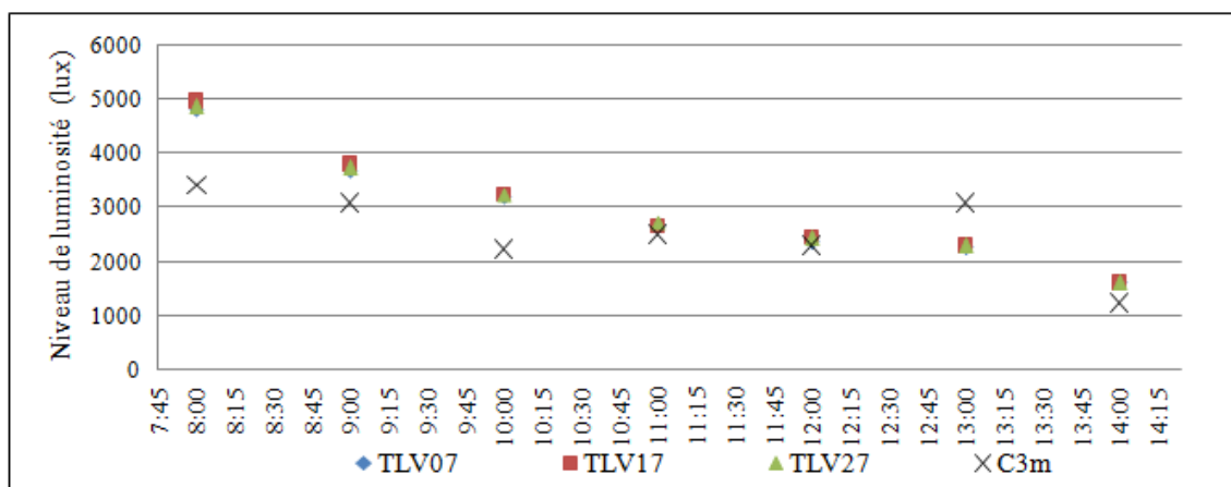
Figure-A V-18 : Variation du coefficient TLV du store, Hsm2, C3s, 22 juin 2017
