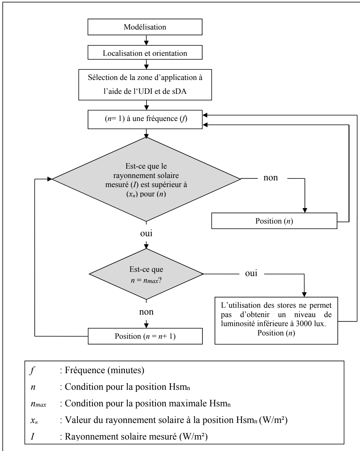
Figure 4.29 : Schéma pour la séquence de contrôle des stores motorisés adapté du schéma de Olbina et Hu (2012).
