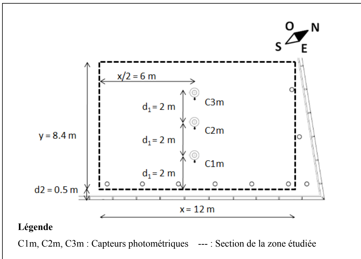
Figure 3.4 : Schéma expérimental pour la zone étudiée
