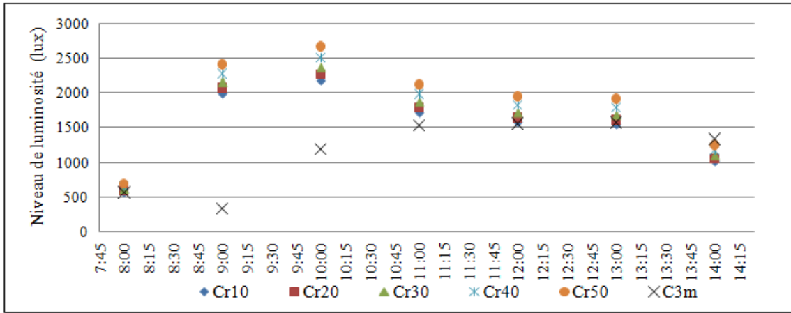
Figure-A V-9 : Variation du coefficient Cr du sol extérieur, Hsm1, C3s, 24 mars 2017
