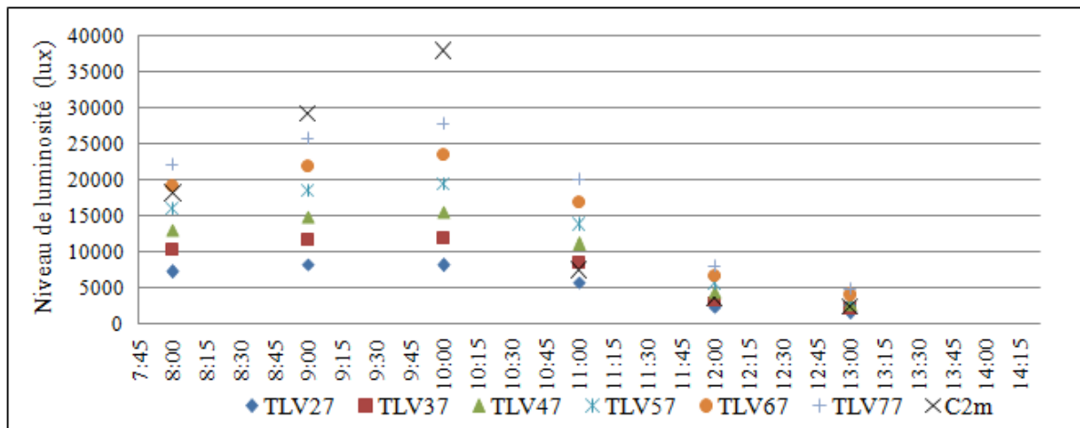
Figure 4.14 : Variation du coefficient TLV du vitrage, Hsm1, C2s, 14 octobre 2016
