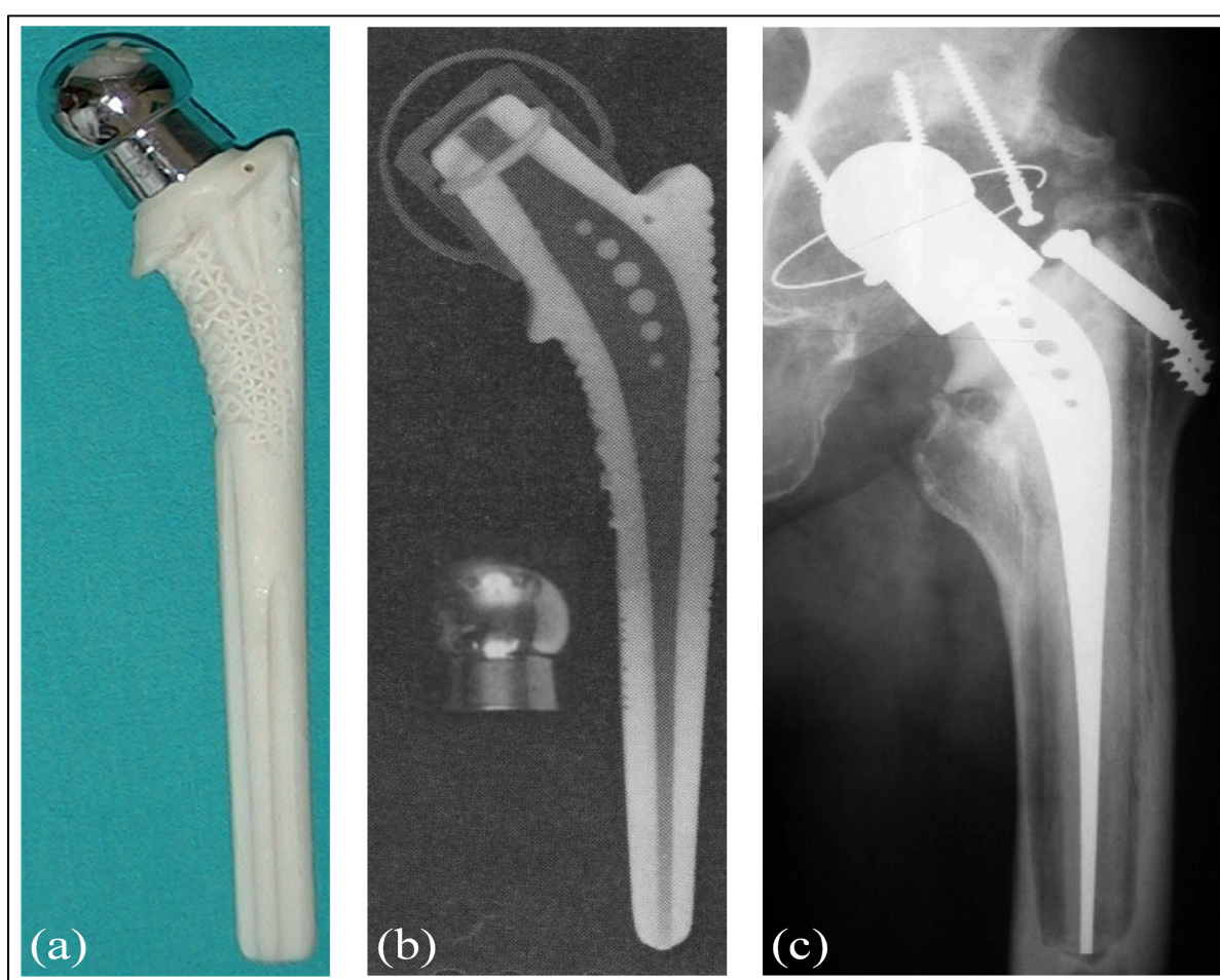
Figure 1.8 (a) Tige isoélastique, (b) Vue en coupe de la tige illustrant l'épaisseur de la couche de polymère et de la tige centrale, (c) Radiographie illustrant l'ostéolyse à l'interface polymère-os après une implantation de 9.7 ans.
