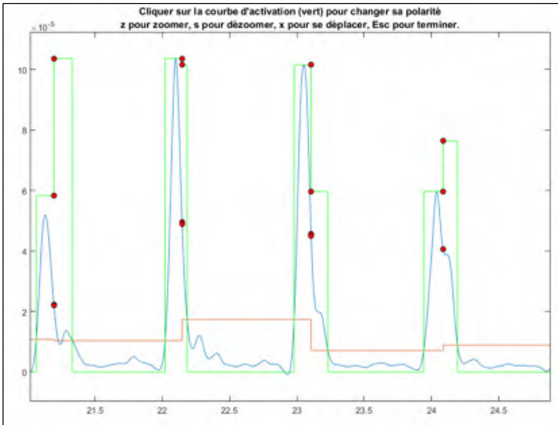
Figure 4.11 : Détection des activations lorsqu'un seuil est défini par cycle de marche
