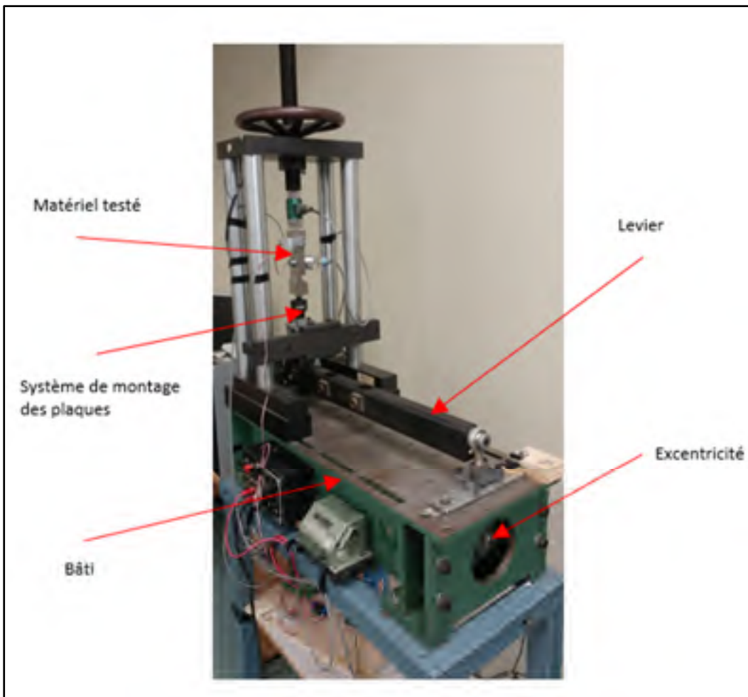
Figure 2.1 Banc d'essai
