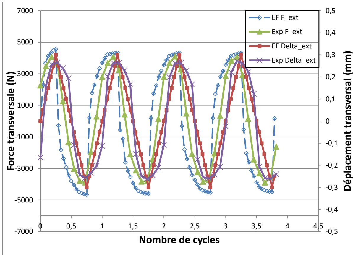
Figure 4.1 Forces transversales et déplacement transversaux en fonction des cycles
