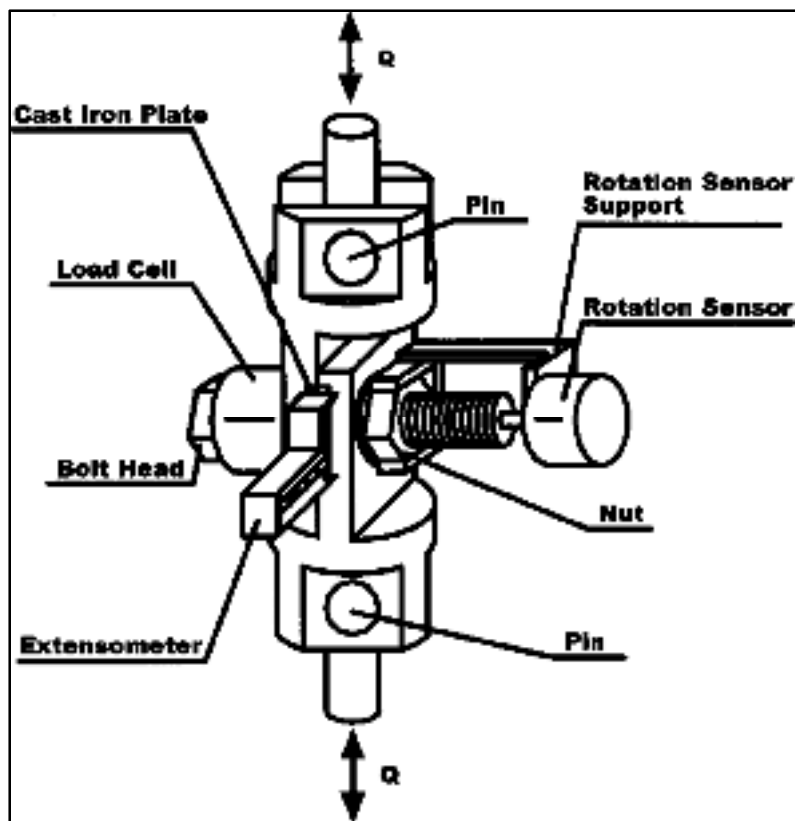
Figure 1.4 Autre montage avec la présence des capteurs Tirée de (Jiang et al., 2003)
