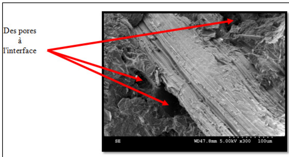
Figure 3.8 Des pores au niveau de l'interface
