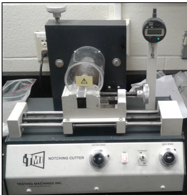
Figure 2.11 TMI coupe échantillon à encoche motorisé
