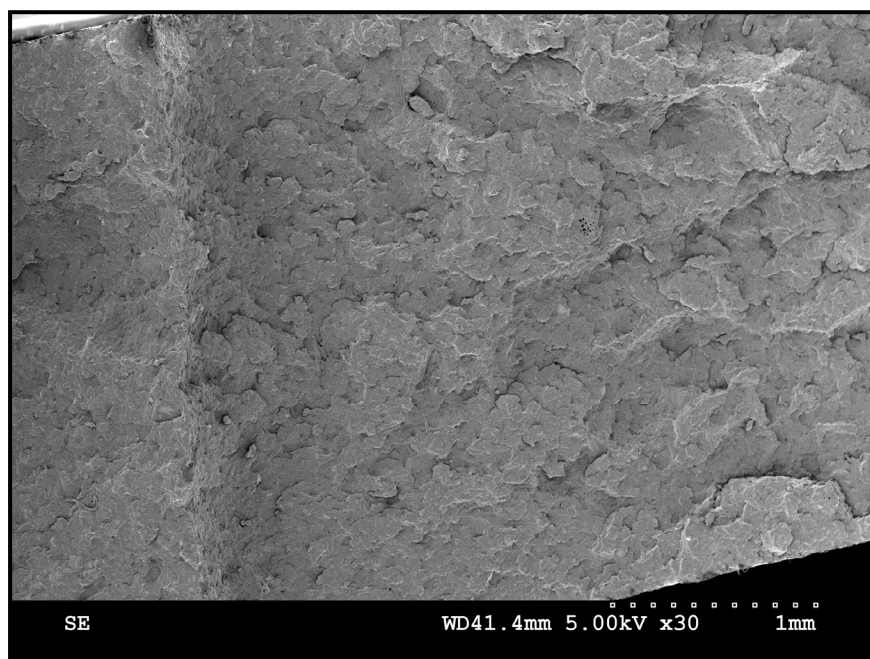
Figure 3.16 Étude microscopique de la surface de rupture d'un échantillon de la F1 de l'essai d'impact
