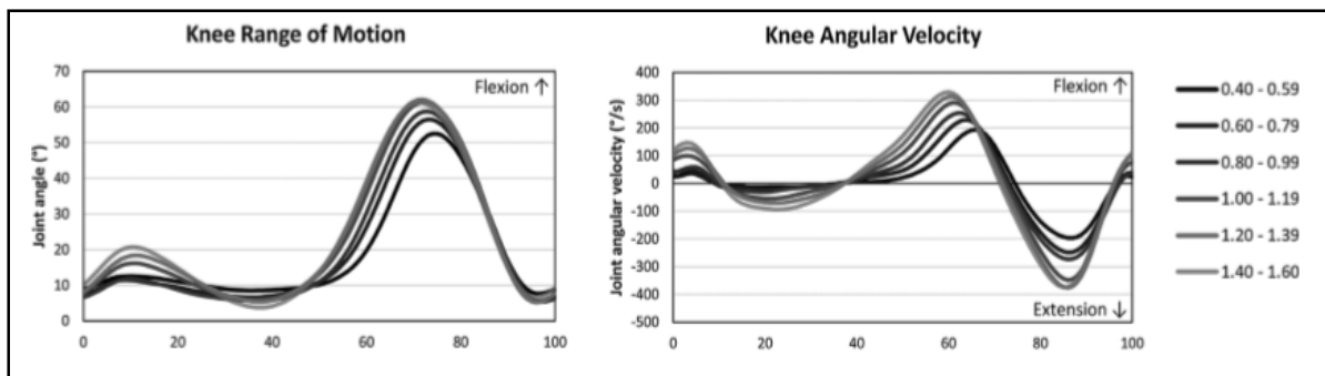
Figure 1.10 Angle et vitesse angulaire du genou dans le plan sagittal à différentes vitesses de marche
