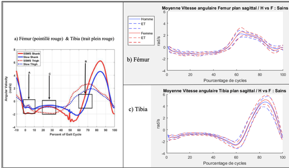
Figure 5.3 Comparaison des courbes de vitesse angulaire du fémur et du tibia dans le plan sagittal – a) Courbes de vitesse angulaire du fémur (pointillé rouge) et tibia (trait plein rouge) – Tiré de Allseits et al., (2017) – b) Résultat de la courbe de vitesse angulaire du fémur – c) Résultat de la courbe de vitesse angulaire du tibia
