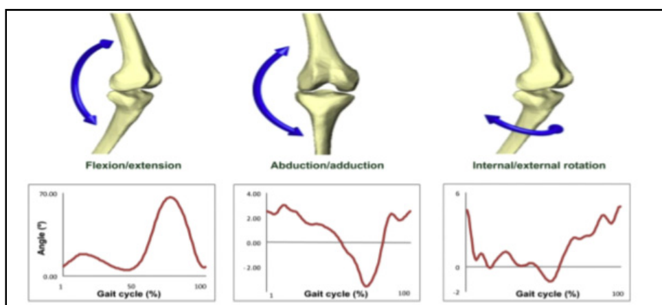
Figure 1.6 Patrons de marche du genou dans le plan sagittal, frontal et transversal
