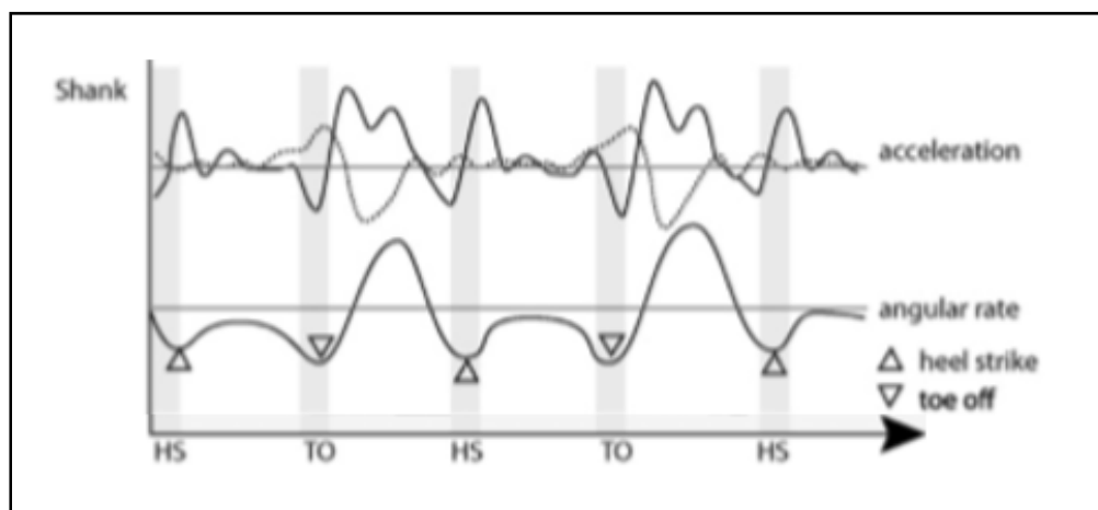
Figure 1.20 Vitesse angulaire et accélération antéro-postérieur du tibia dans le plan sagittal Tiré et adapté de Rueterbories et al. (2010)
