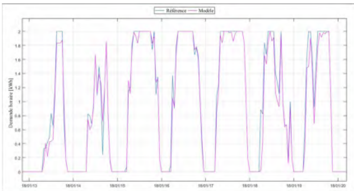
Figure 5.7 Comparaison entre la référence et le modèle de la demande horaire du serpentin électrique du VC 4-49 13-20/01/2018
