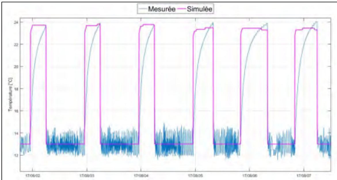
Figure 5.6 Température d'alimentation mesurée et simulée de l'UTA 804 (simulation initiale) 02-07/08/2017
