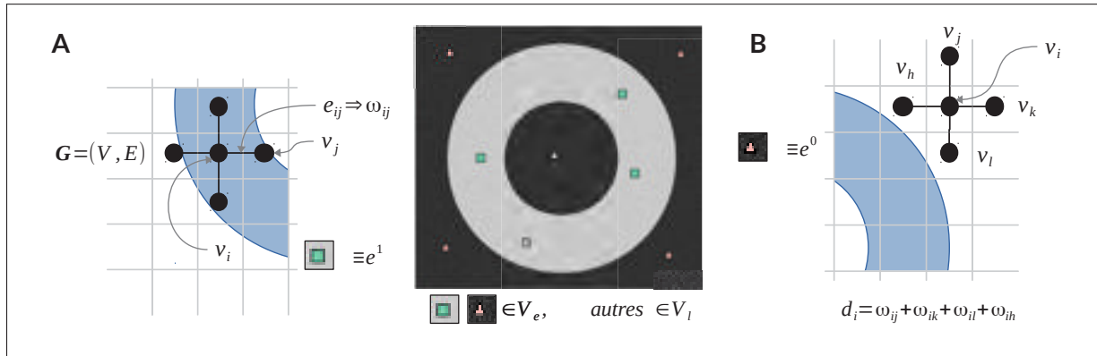
Figure 5.7 Construction du graphe pondéré pour représenter l'image dans la formulation de la segmentation par marche aléatoire sur un fantôme numérique 2D. (A) Le graphe pondéré G est composé de nœuds v_i \in V , qui sont reliés par des arêtes e_{ij} \in E . Chacune d'elles possède un poids \omega_{ij} qui quantifie la relation existante entre deux nœuds voisins. (B) Le degré d'un nœud correspond à la somme des poids associés aux arêtes incidentes à ce nœud.
