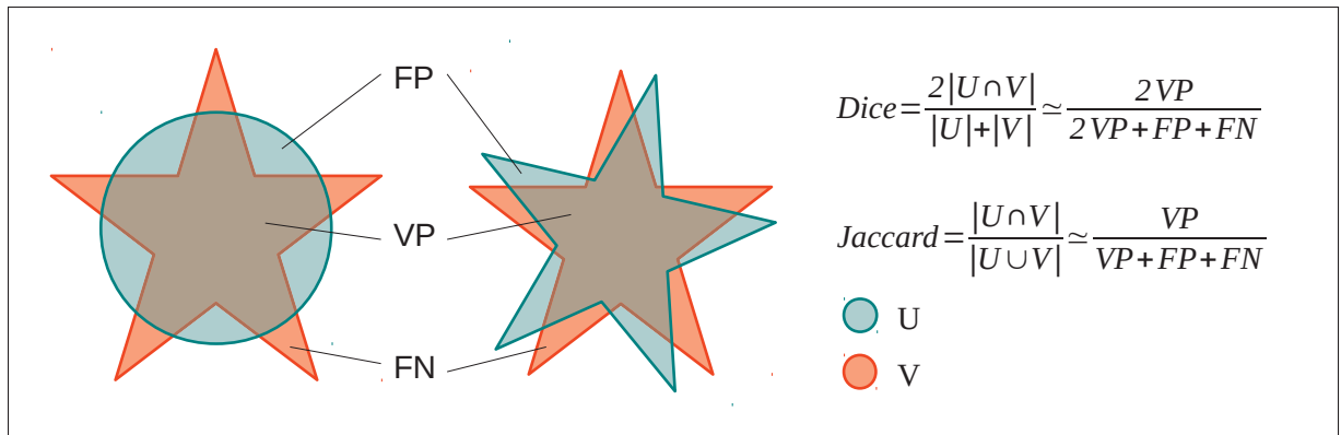
Figure 2.13 Importance du choix des métriques de validation pour appuyer l'analyse de la performance d'un algorithme de segmentation : cas de l'indice de Dice et de Jaccard. L'étoile est comparée avec un cercle (gauche) et avec une étoile de taille similaire qui a subi une rotation (droite). Dans les deux cas, la quantité de faux négatifs (FN) et de faux positifs (FP) est équivalente par rapport à la quantité de vrais positifs (VP). Les métriques basées sur le chevauchement, comme Dice ou Jaccard, donneront des résultats équivalents, alors que la forme de gauche se rapproche beaucoup plus de la réalité que la forme de droite, tirées et adaptées de Taha & Hanbury (2015).
