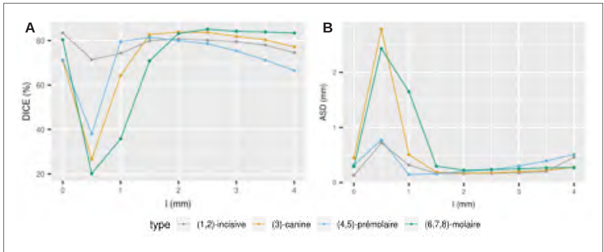
Figure 4.12 Évolution de deux métriques de performance de détection de la pulpe dentaire en fonction de la taille de l'élément structurant utilisé pour rehausser les vallées de l'image. (A) L'indice de Dice informe sur le chevauchement entre le masque de la pulpe et le masque de référence. (B) La distance surfacique moyenne-symétrique informe sur l'écart entre les surfaces des deux masques. La valeur à l = 0 \text{ mm} représente la valeur que prend la métrique avec l'image originale.
