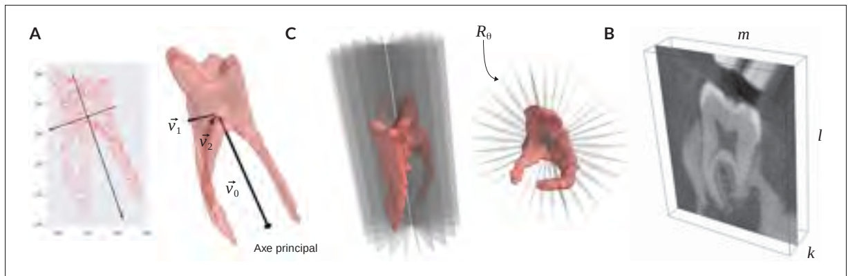
Figure 5.3 Principes de la re-formation multiplanaire centrée autour de la pulpe. (A)
