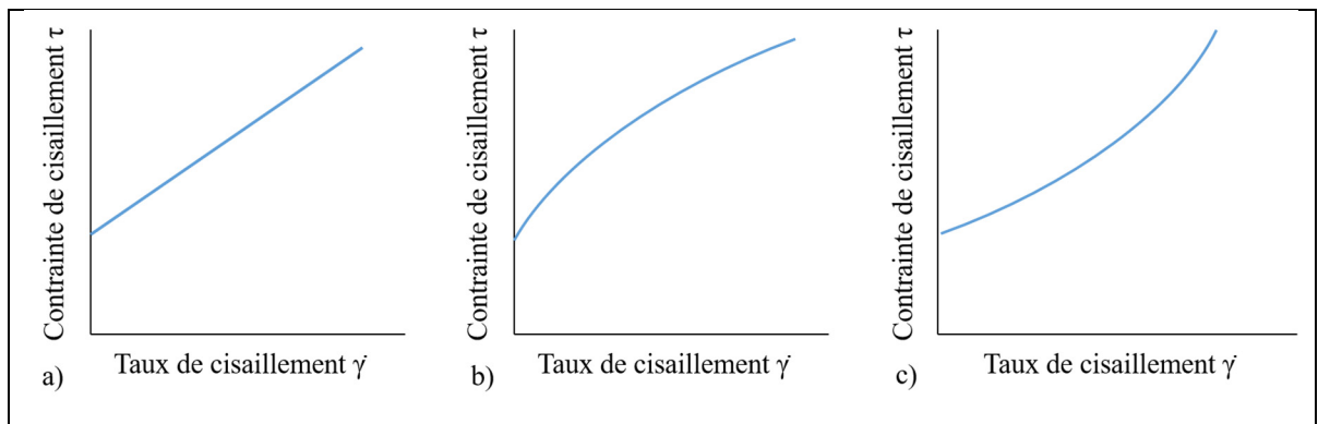
Figure 1.6 Courbe d'écoulement pour un a) fluide à seuil ; b) fluide viscoplastique rhéofluidiant ; c) fluide viscoplastique rhéopéaissant
