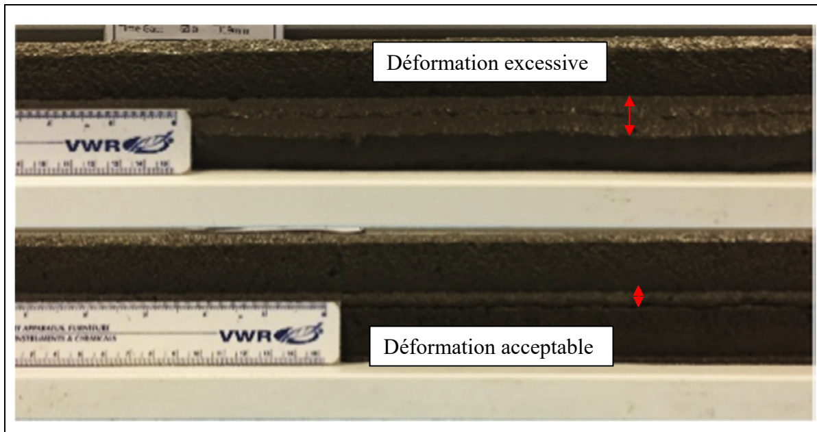
Figure 1.20 Différence entre des couches passant le critère d'imprimabilité (en bas) et des couches ayant subi une trop grande déformation (en haut) Tirée de Kazemian et al. (2017)
