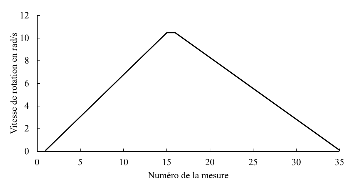
Figure 1.10 Procédure de contrôle de la vitesse de rotation pour effectuer la mesure d'après les recommandations du NIST
