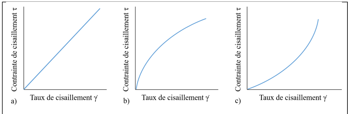
Figure 1.5 Courbes d'écoulement pour un comportement a) newtonien ; b) rhéofluidifiant ; c) rhéopéaissant
