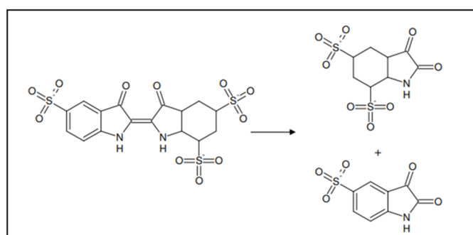
Figure 2.4 : Réaction du Carmin Indigo avec l'ozone
