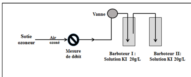
Figure 2-5 : Représentation schématique de la méthode iodométrique
