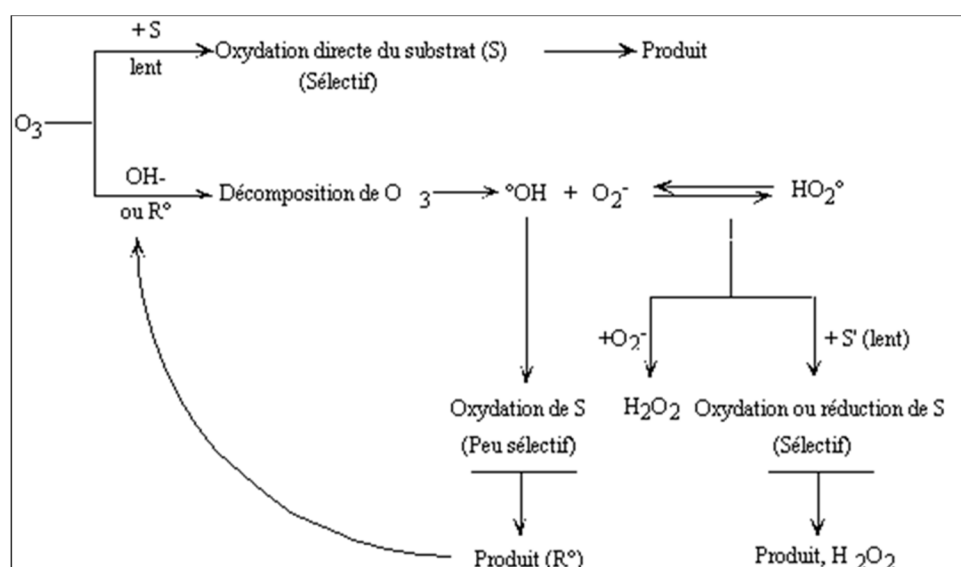
Figure 1.4 : Différentes modalités d’interaction de l’ozone dans une solution aqueuse (Hoigne & Bader, 1976 ; Hoigne & Bader, 1978)
