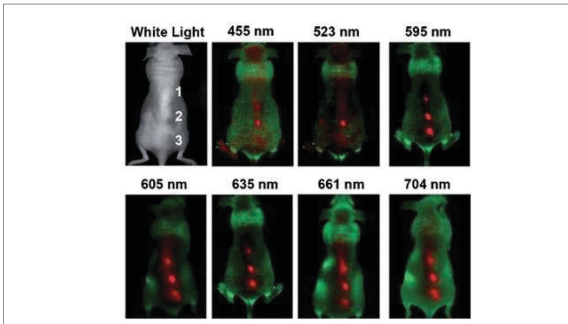
Figure 1.4: Images à différentes longueurs d'onde d'excitation de la fluorescence in vivo d'une souris ayant reçu une injection de PQC. Le rouge et le vert représentant les signaux fluorescents des PQC et la fluorescence propre des tissus, respectivement. (H. Tao et al, 2012)
