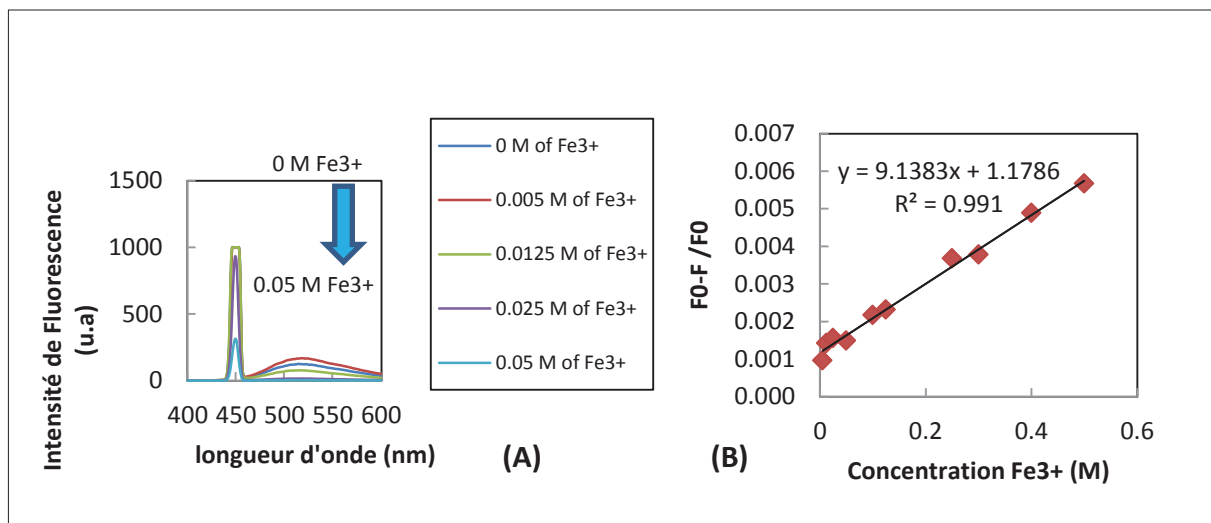
Figure 3.10: A) Spectres de fluorescence des PQC à concentration croissante en \text{Fe}^{3+} B) Intensité maximale de fluorescence des PQC avec des concentrations de \text{Fe}^{3+} (excitation 350 nm)
