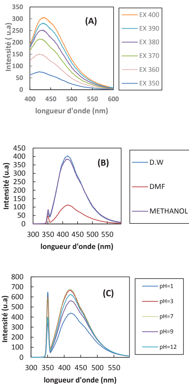
Figure 3.3: Spectres d'émission de fluorescence des points carbonés avec A) à 250 °C pendant 10 minutes avec longueurs d'onde d'excitation variables B) avec des solvants variables C) dans une plage de pH.
