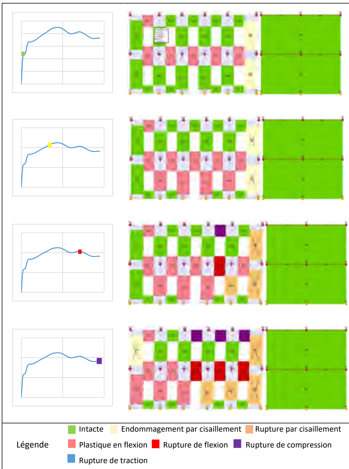
Figure 3.5 Identification des différents états de dommage
