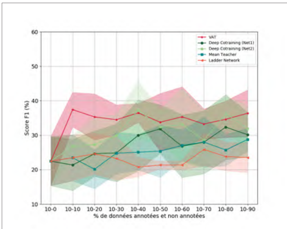
Figure 4.9 Expérience 1 sans pré-entraînement, base TUPAC
