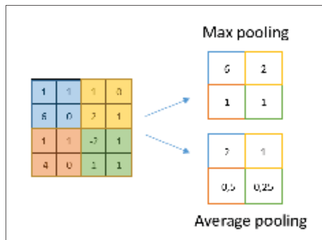
Figure 1.6 Exemple de couches de pooling
