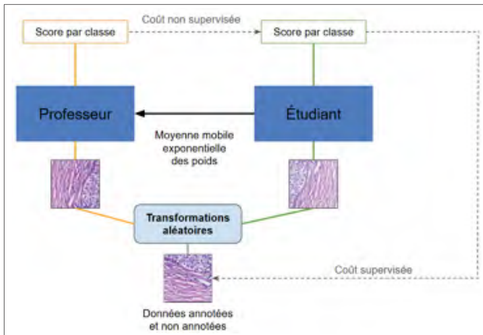
Figure 2.8 Schématisation du fonctionnement de Mean teacher (Tarvainen & Valpola (2017))
