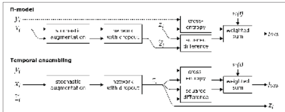
Figure 2.3 Schématisation du fonctionnement de \Pi -net et de Temporal ensembling (Laine & Aila (2016)).
