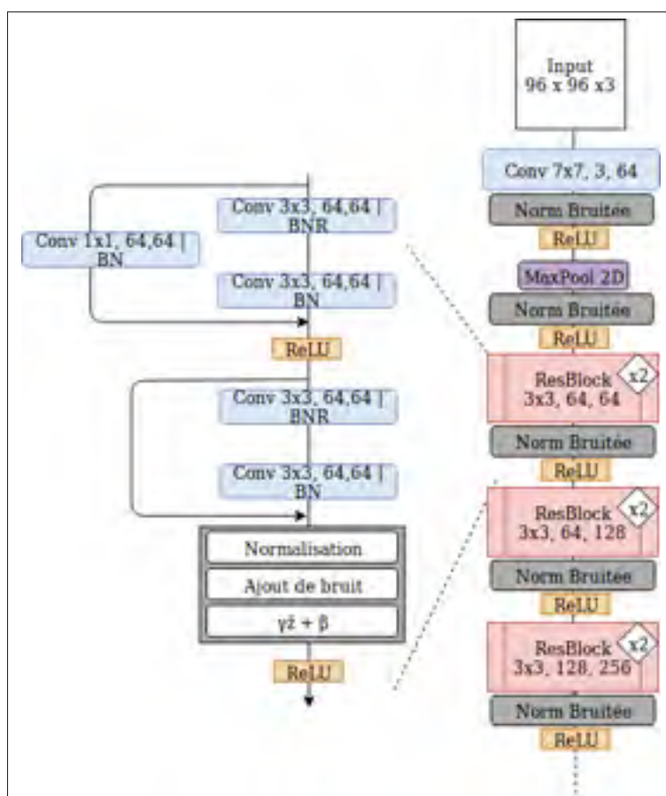
Figure 2.6 Schématisation d'une partie de l'encodeur bruité basé sur un ResNet-18
