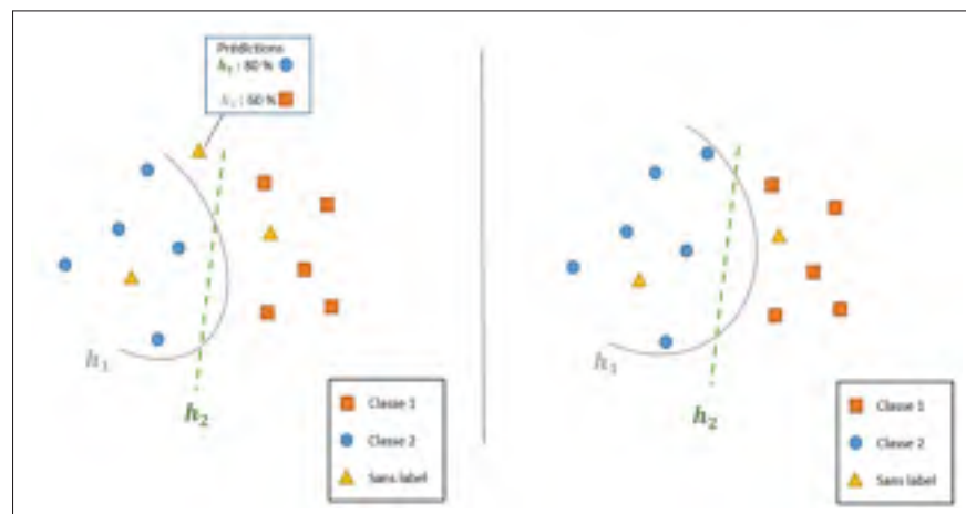
Figure 2.2 Schématisation d'une itération de co-training
