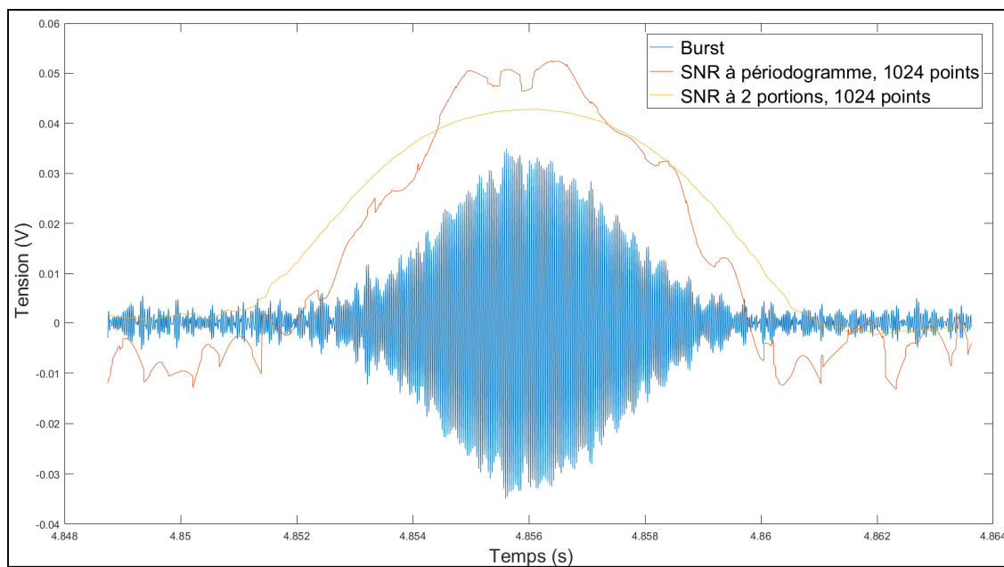
Figure 4.7 Différences entre un SNR à périodogramme et SNR à 2 portions
