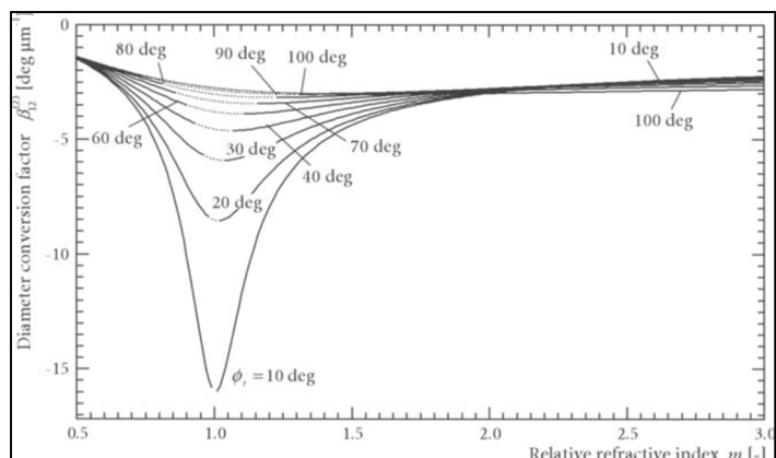
Figure 1.13 Influence de l'indice de réfraction relatif sur le facteur de conversion Tirée de Albrecht (2003, p. 422)
