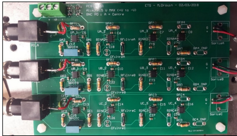
Figure 3.11 Photographie du circuit imprimé
