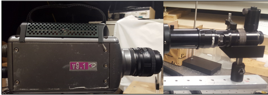
Figure 2.8 Caméra Nikon avec son objectif de 50 mm (à gauche) et microscope Navitar Zoom 6000 (à droite)
