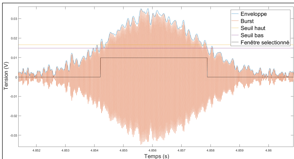
Figure 4.6 Détection par bascule de Schmitt
