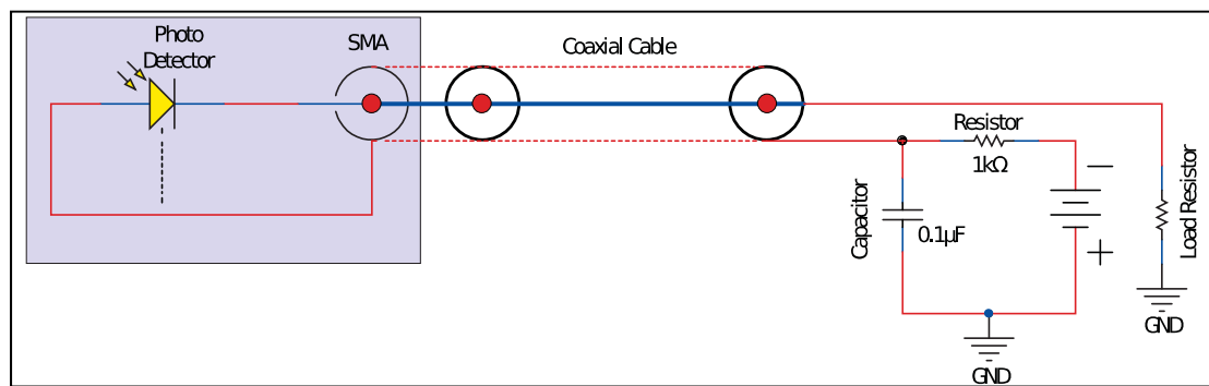
Figure 3.8 Circuit électrique conseillé par Thorlabs Source : Thorlabs
