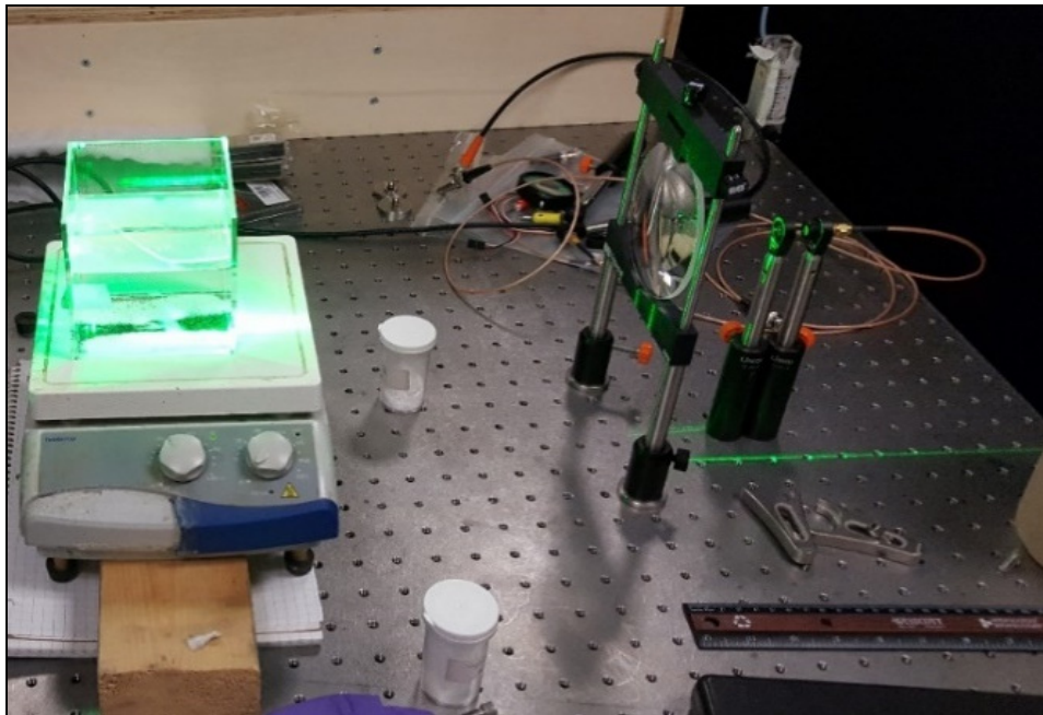
Figure 2.5 Disposition du capteur
