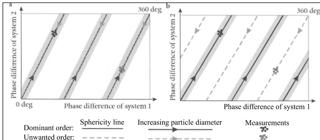
Figure 1.17 Technique pour détecter l'effet gaussien a. Le rapport des coefficients de conversion est de 3 et b. Le rapport des coefficients de conversion est de 2.5 Adaptée de Albrecht et al. (2003, p. 456)
