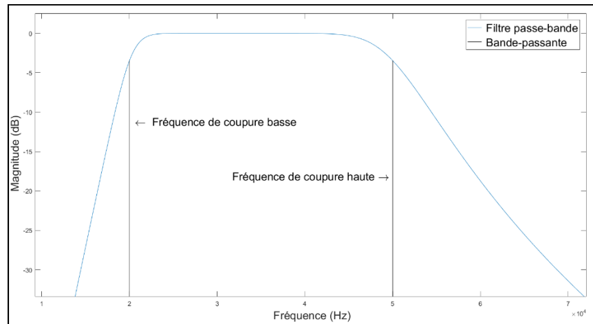
Figure 4.2 Filtre bande-passante
