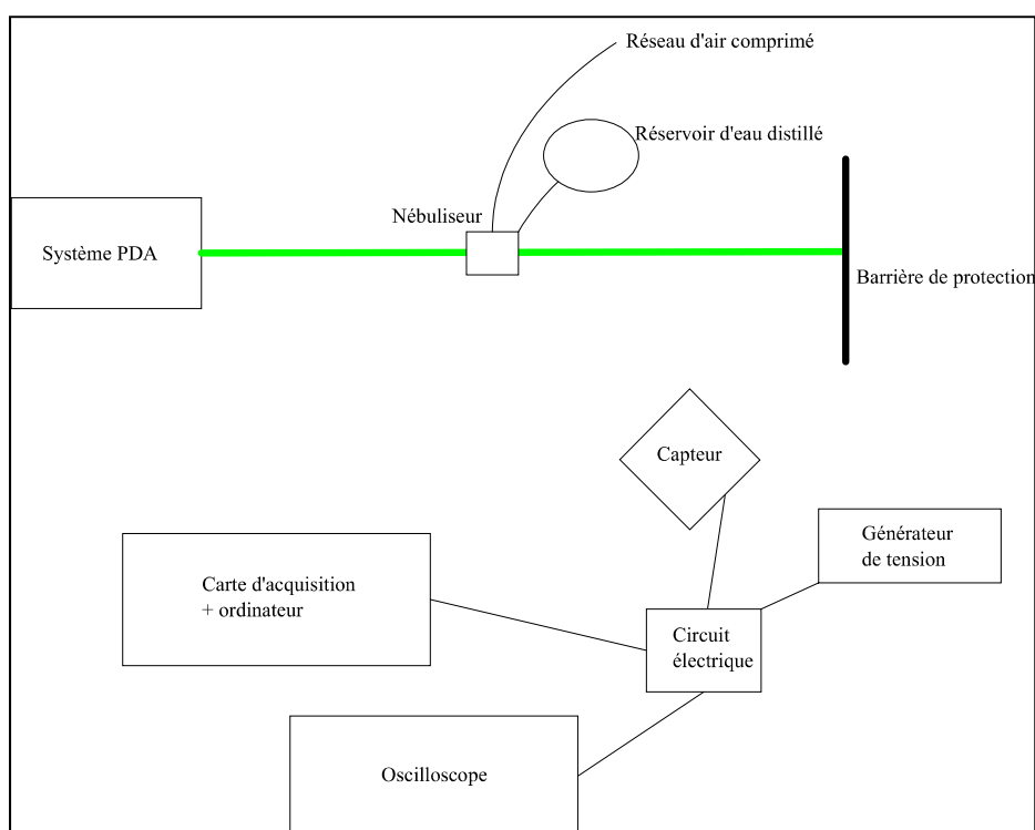
Figure 2.7 Représentation schématique du montage expérimental avec dispositif de génération de sprays
