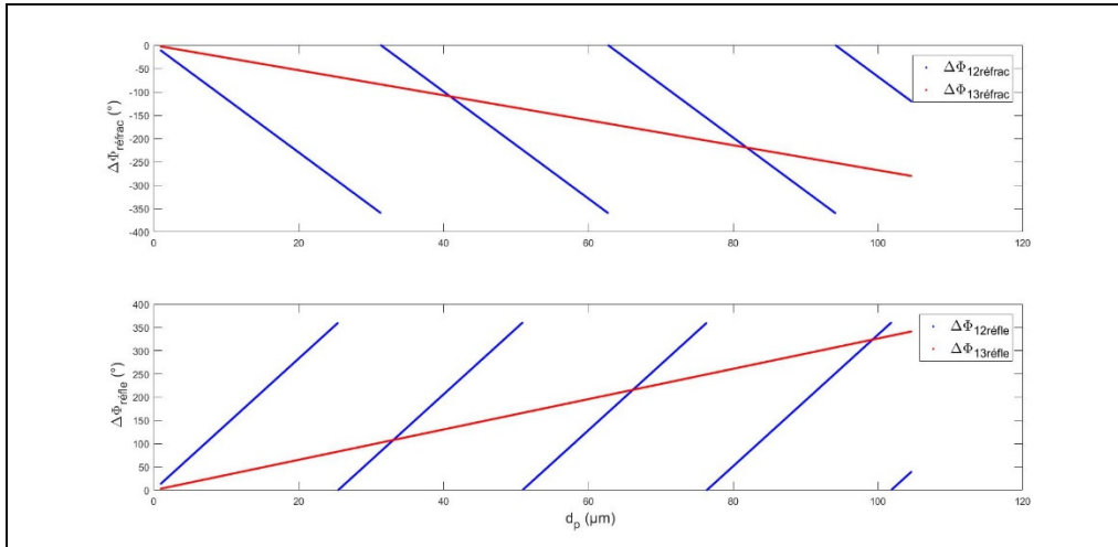
Figure 3.5 Diagramme déphasage/diamètre du système PDA pour un angle hors-axe de 30^\circ
