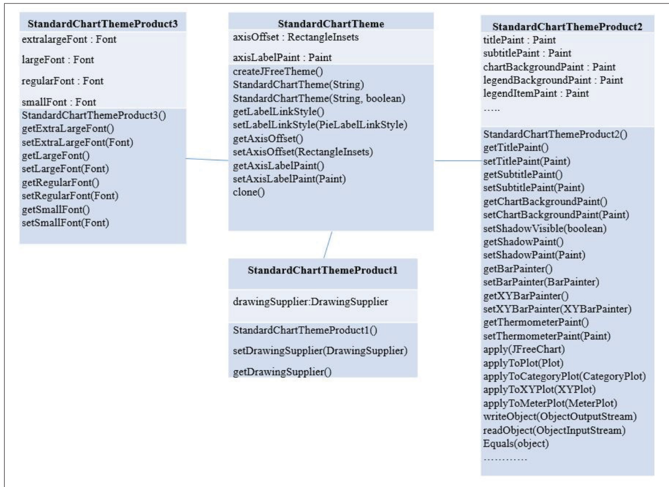
Figure 2.2 Restructuration de la classe StandardChartTheme avec notre outil
