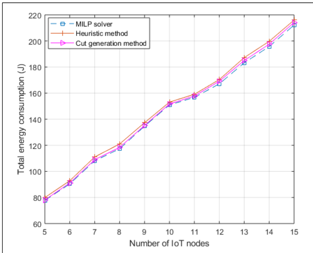
Figure 4-20 La comparaison des résultats de solver MILP avec la méthode de coupe du plan et la méthode heuristique en appliquant l'algorithme DT_IoTMC
