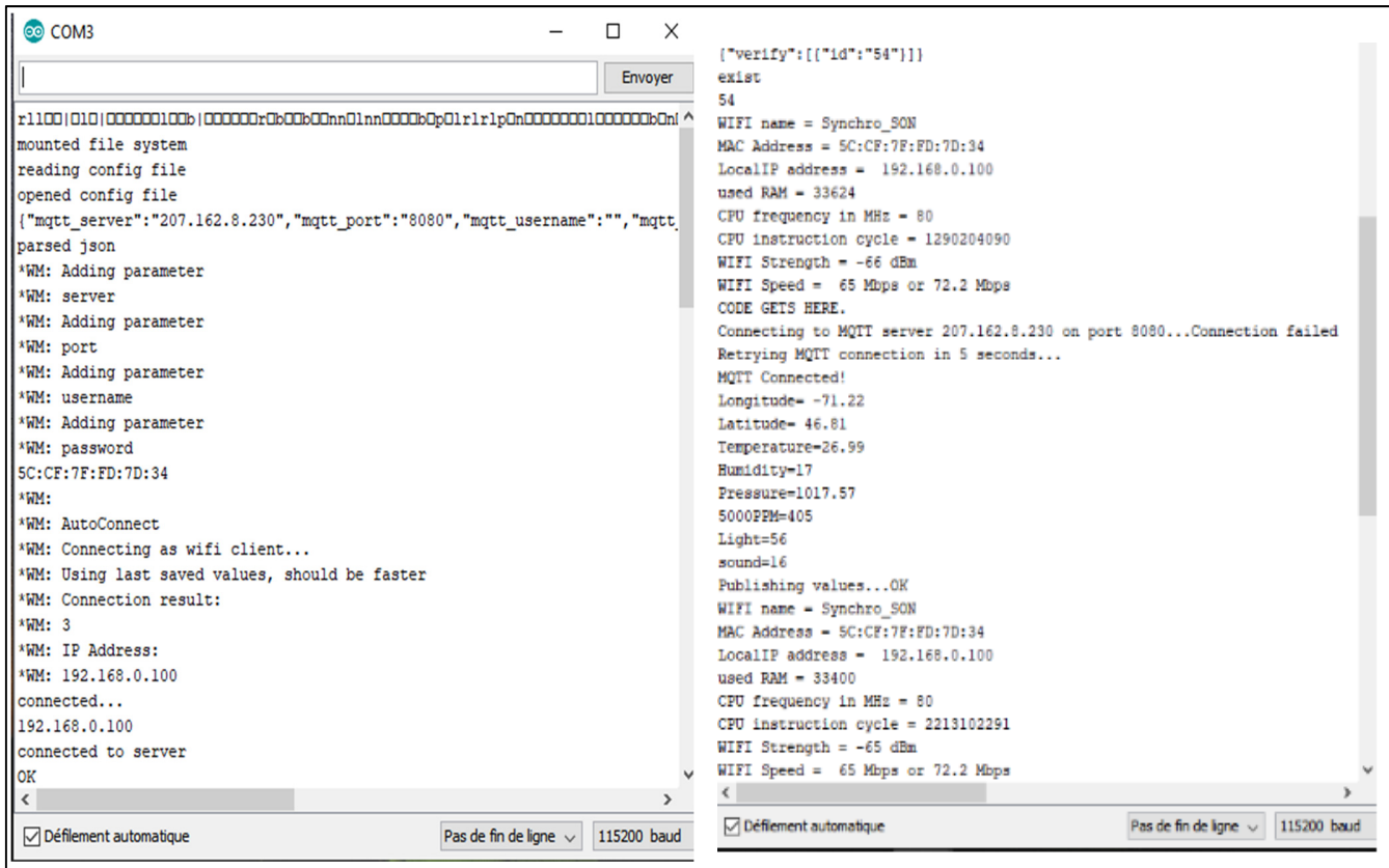
Figure 4-2 Les données interceptées au niveau un nœud IdO de type ESP8266
