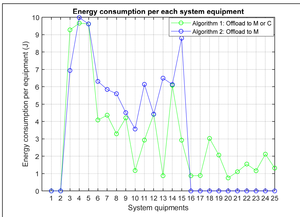
Figure 4-19 La consommation d'énergie de chaque équipement du système
