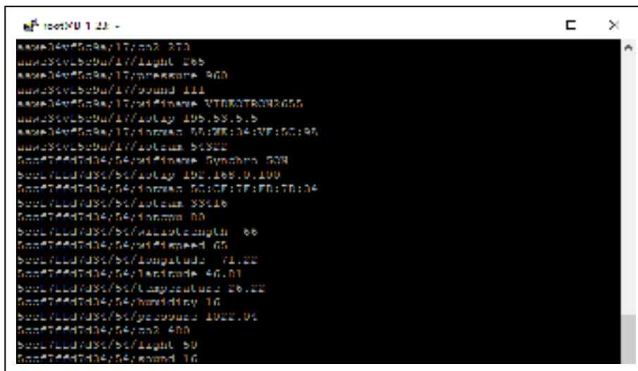
Figure 4-3 Les données interceptées au niveau de courtier Mosquitto
