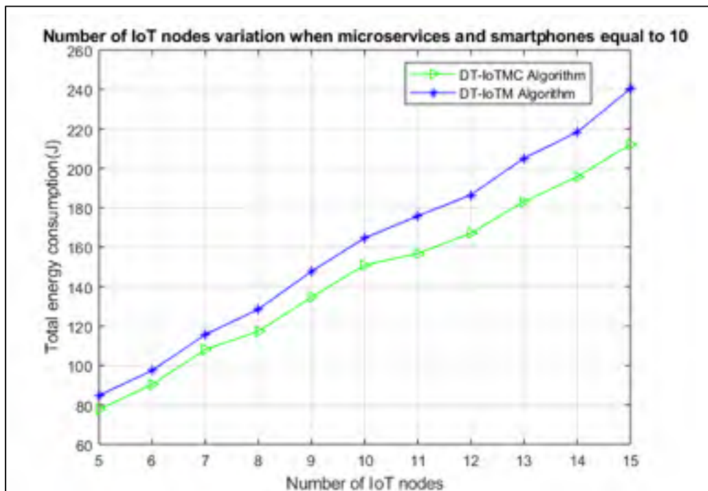
Figure 4-18 L'effet de variation du nombre des nœuds IdO sur la consommation totale de l'énergie quand M et les microservices sont égales à 10
