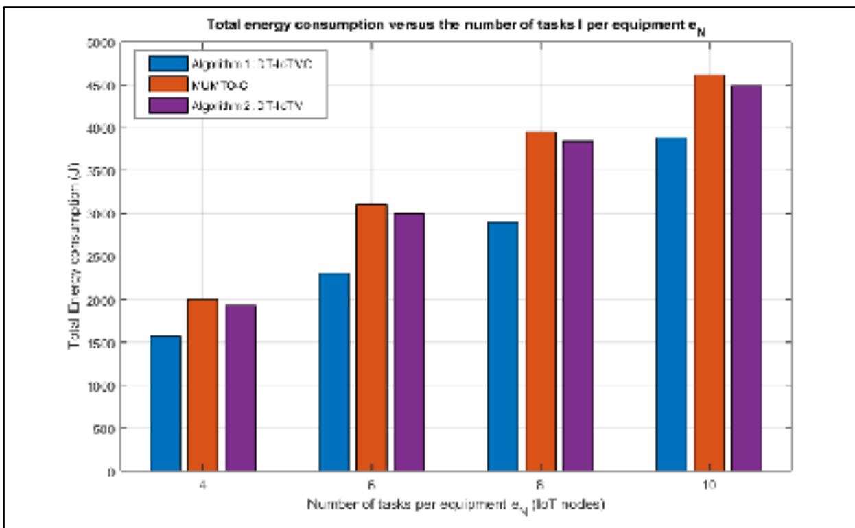
Figure 4-23 L'effet de la variation de nombre de tâches déchargeables par nœud IdO sur la consommation totale d'énergie en utilisant les deux algorithmes proposés et la solution Baseline
