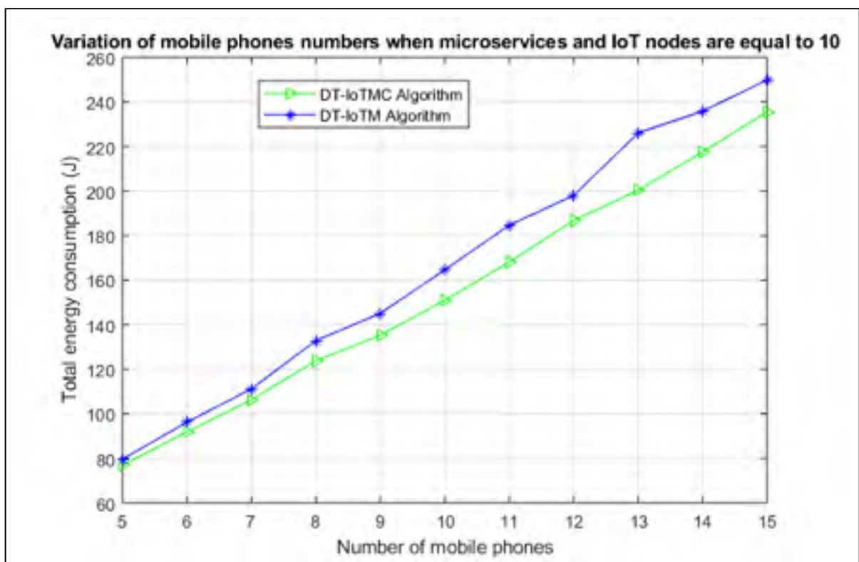
Figure 4-22 L'effet de la variation de nombre des appareils mobiles M sur la consommation totale d'énergie quand les microservices et le nombre N sont égales à 10
