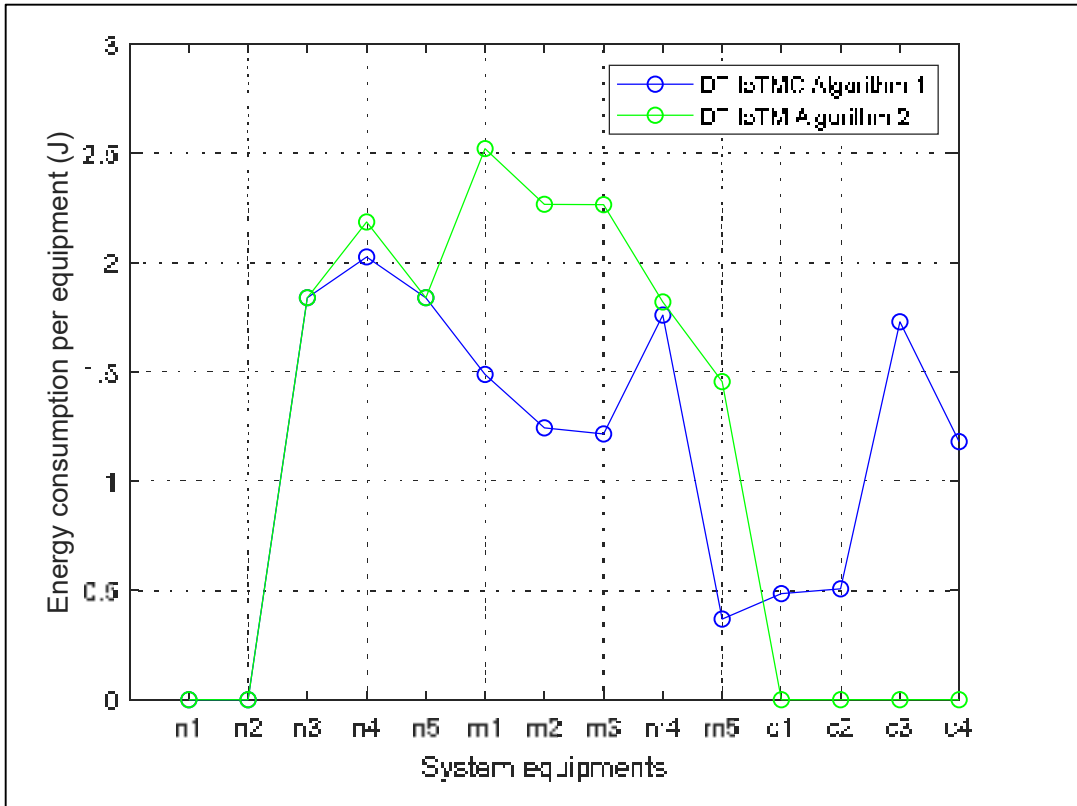
Figure 4-17 La consommation énergétique totale de chaque équipement du système en exécutant les deux algorithmes
