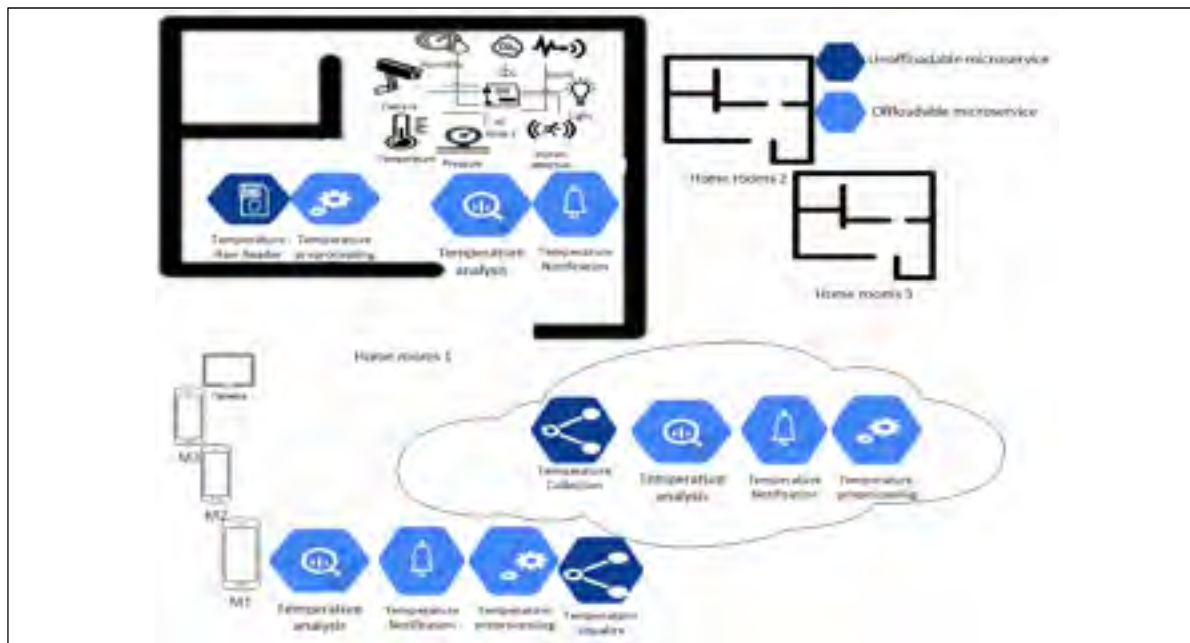
Figure 3-1 Application IdO basée sur des microservices distribués dans un milieu hétérogène
