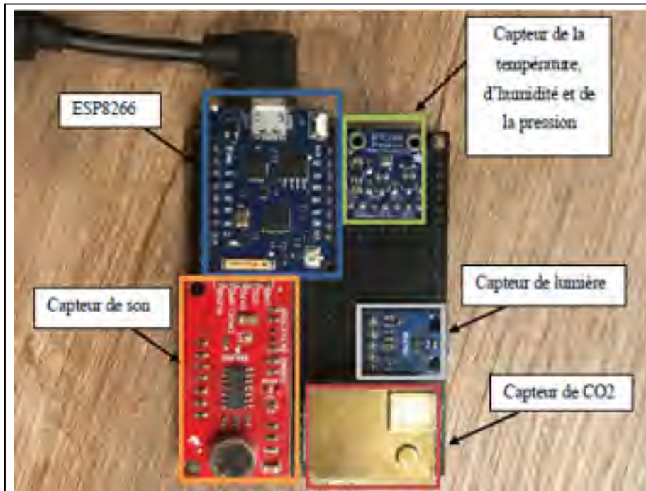
Figure 4-1 Un ESP8266 équipé par différents capteurs (nœud IdO)
