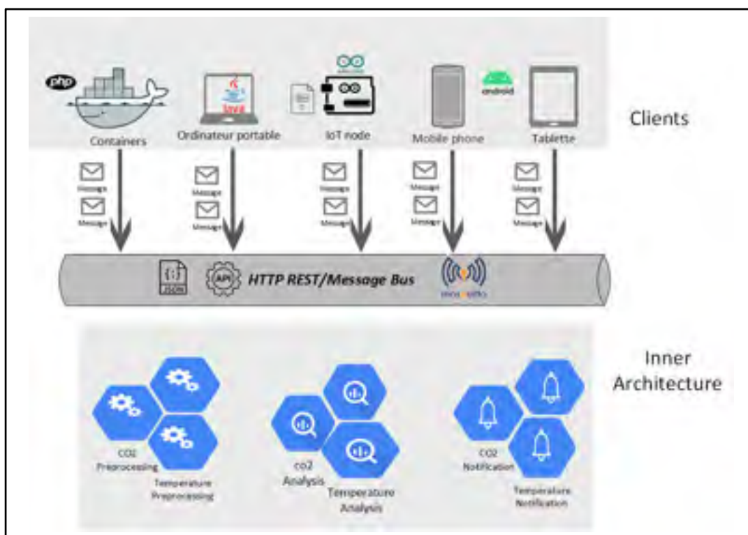
Figure 1-2 Architecture microservices adaptée pour une application IdO
