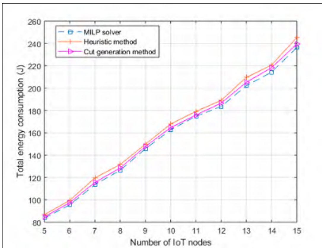
Figure 4-21 La comparaison des résultats de solver MILP avec la méthode de coupure du plan et la méthode heuristique en appliquant l'algorithme DT_IoTM
