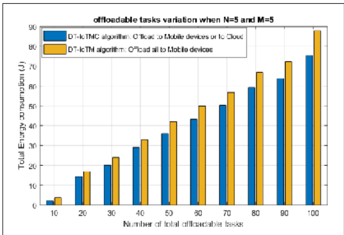
Figure 4-16 Effets de la variation du nombre des tâches déchargeables sur la consommation totale d'énergie quand N=M=5
