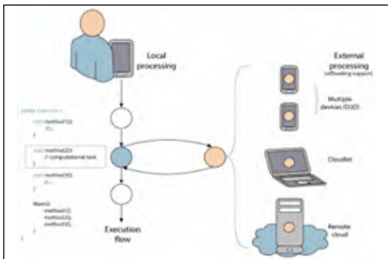
Figure 2-1 Système de déchargement informatique hybride ((Flores et al. , 2017)
