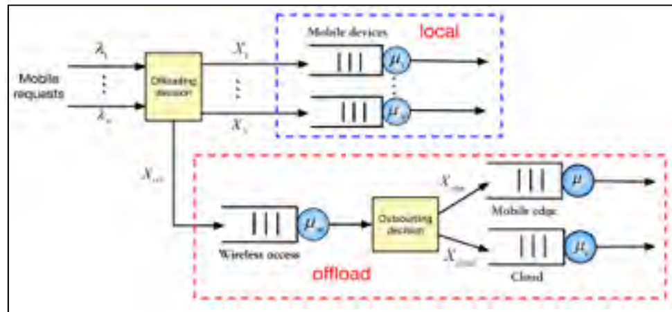
Figure 2-2 Un système hybride de déchargement (Mobile à bord ou nuage) (Ma et al., 2017) et (WU, 2018)
