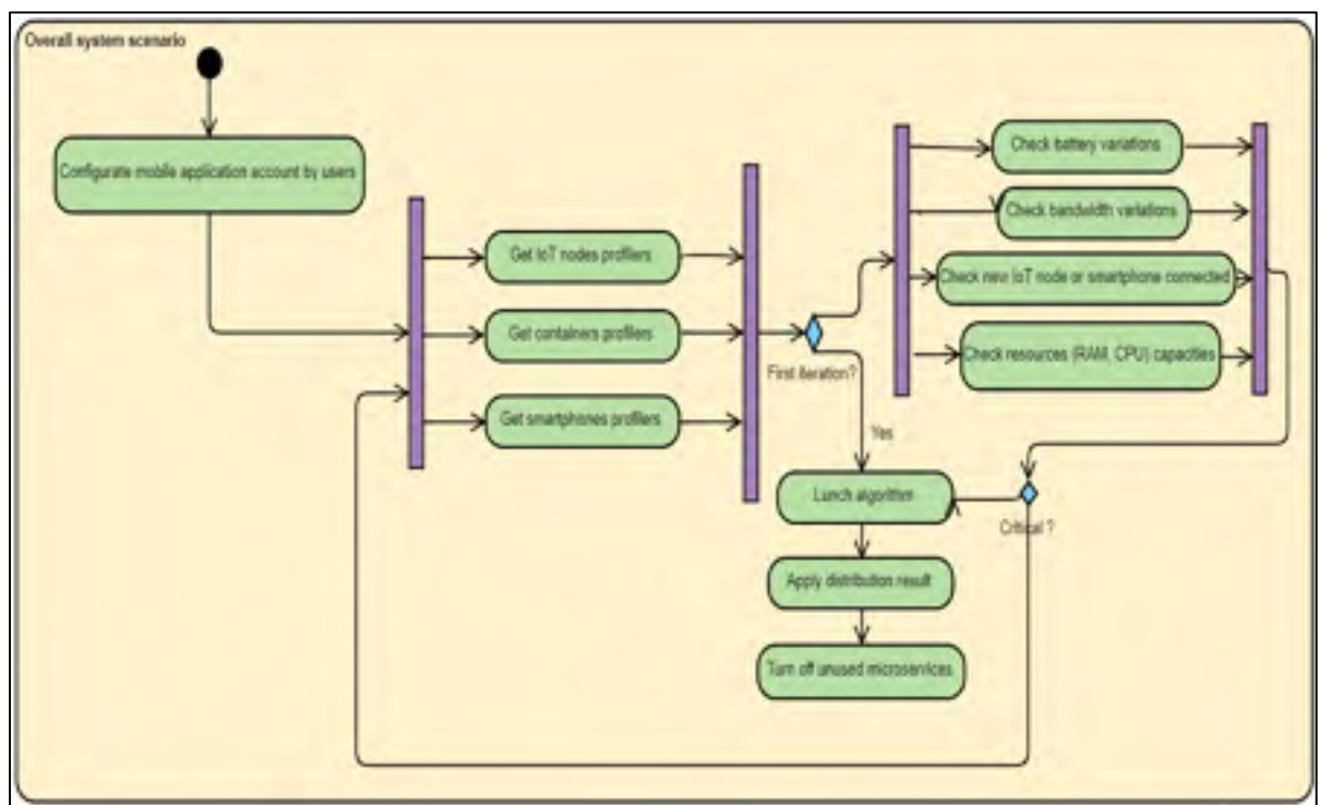
Figure 4-14 Diagramme d'activité pour la solution proposée
