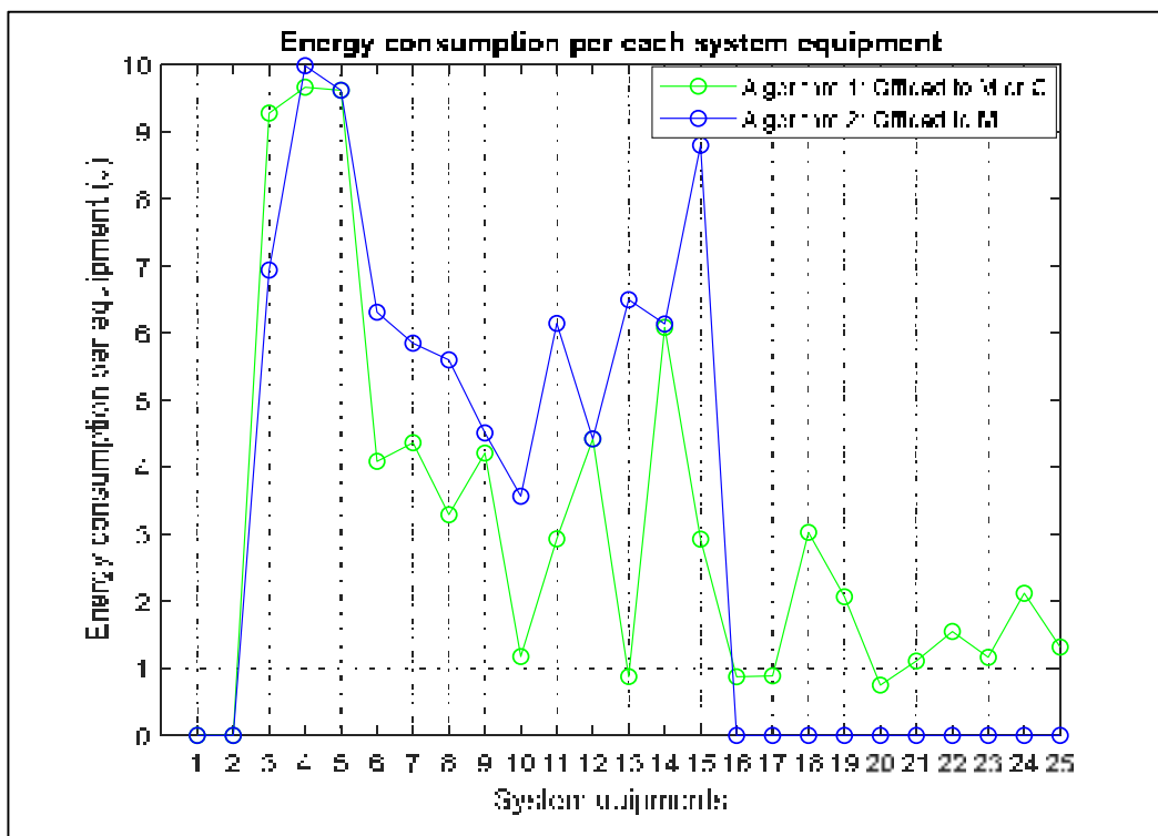
Figure 4-19 La consommation d'énergie de chaque équipement du système
