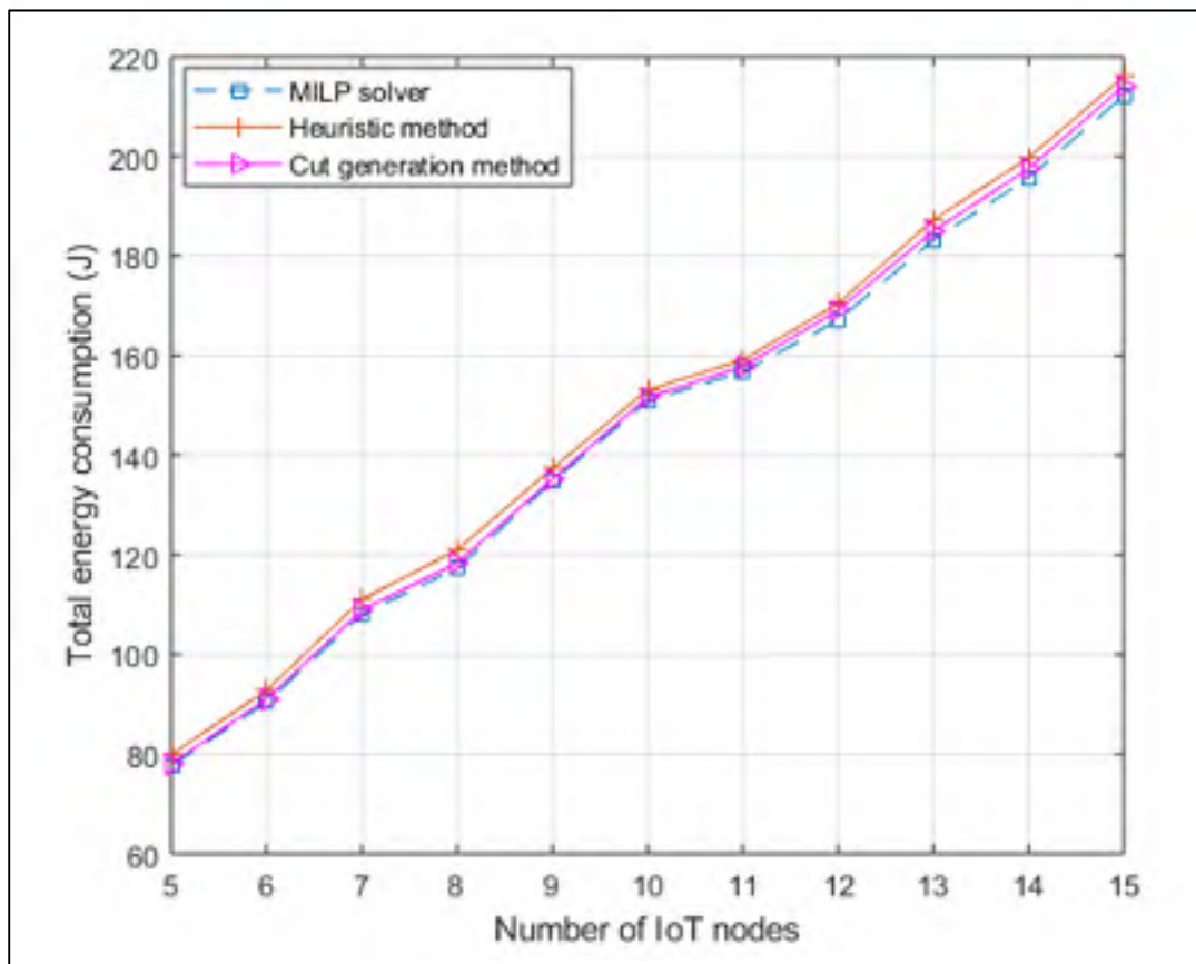
Figure 4-20 La comparaison des résultats de solveur MILP avec la méthode de coupure du plan et la méthode heuristique en appliquant l'algorithme DT_IoTMC
