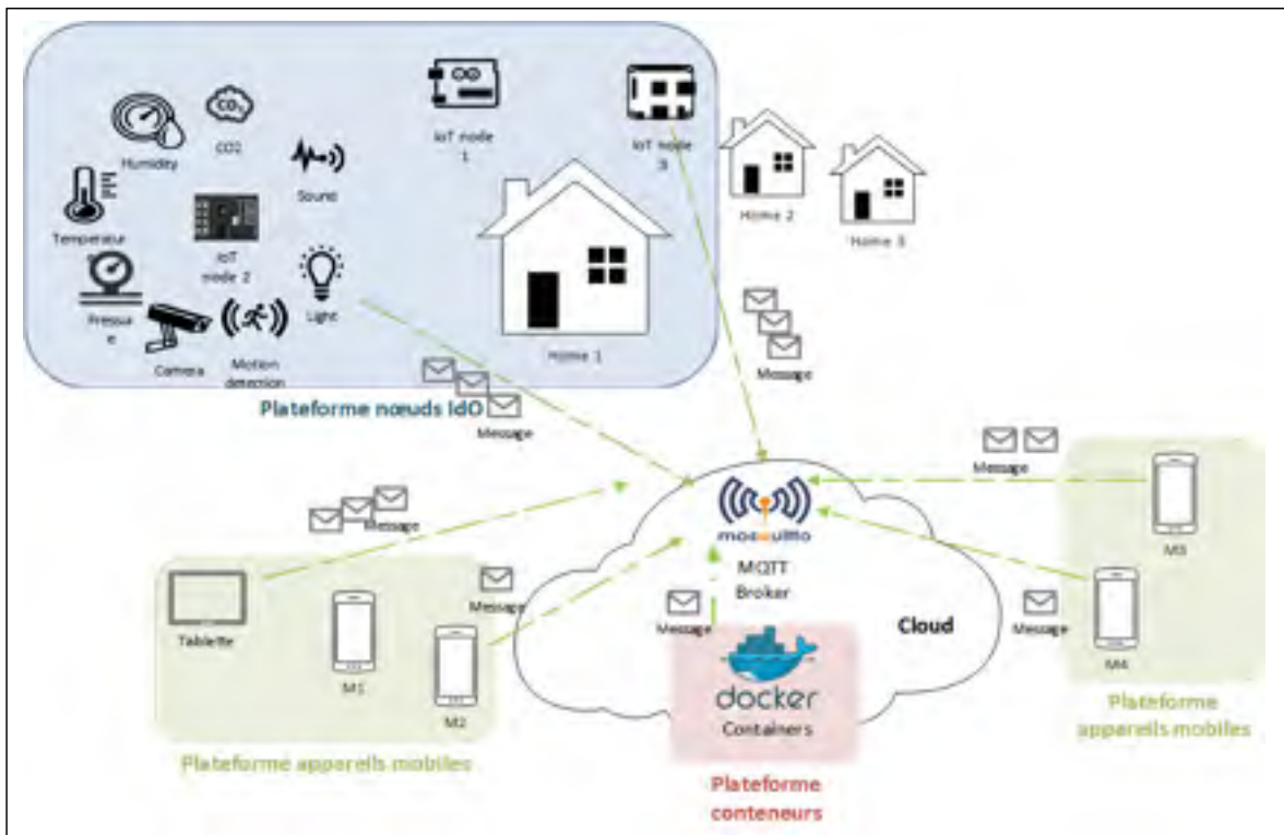
Figure 1-1 Vue globale d'une application IdO pour la maison intelligente
