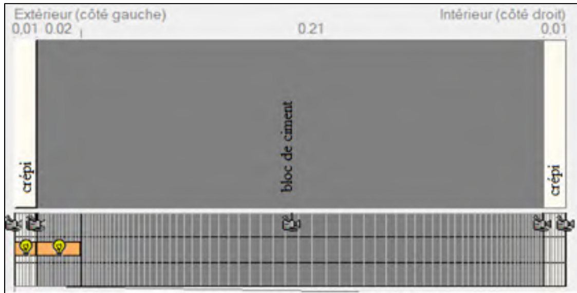
Figure 6.3 Configuration du mur et maillage du cas 1 dans WUFI Pro 6.2 pour la ville de Dori
