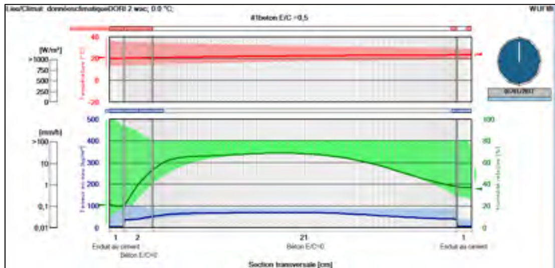
Figure 6.4 Animation du cas 1 pour le taux d'infiltration d'eau de 1\text{m}^3/\text{m}^2\text{h} , la ville de Dori
