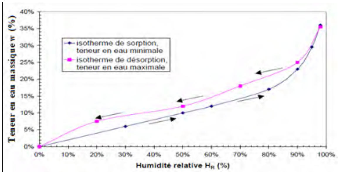
Figure 1.24 Isotherme d'adsorption-désorption des particules de chanvre à T = 20°C Tirée de Cérézo (2005, p.67)
