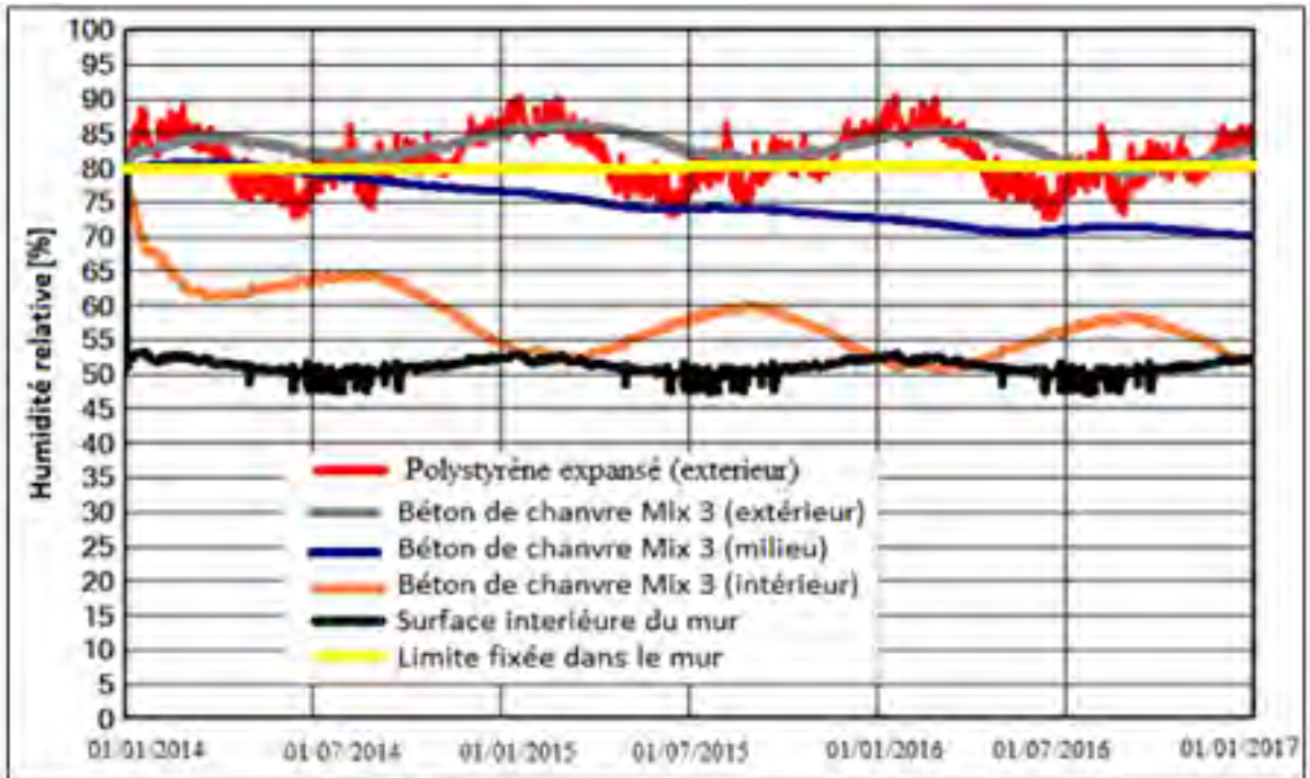
Figure 6.18 Évolution de l'humidité pour un taux d'infiltration de 5 \text{ m}^3/\text{m}^2 \text{ h} : cas 2
