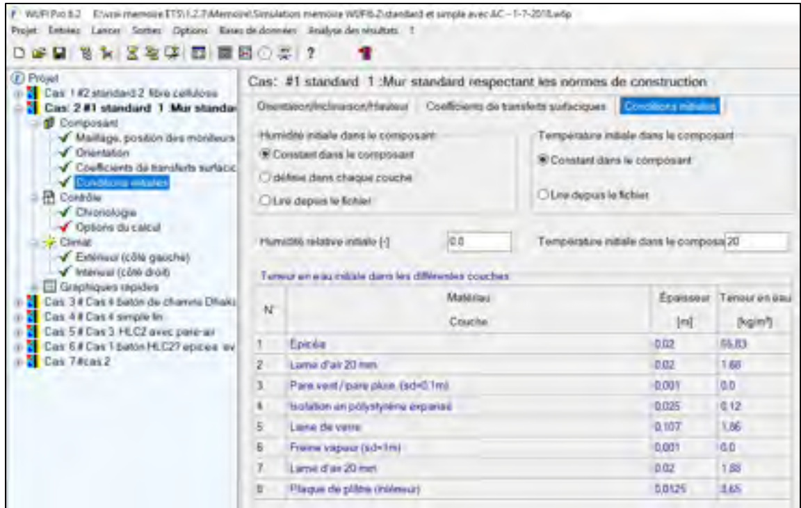
Figure-A II-10 conditions aux limites dans les murs
