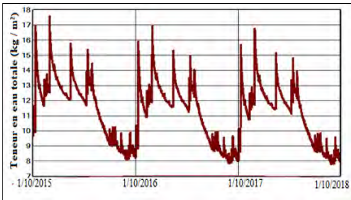
Figure 4.8 Teneur en eau ( \text{kg}/\text{m}^2 ) du mur 1, WUFI Pro 6.2 [Aguérata Kaboré]
