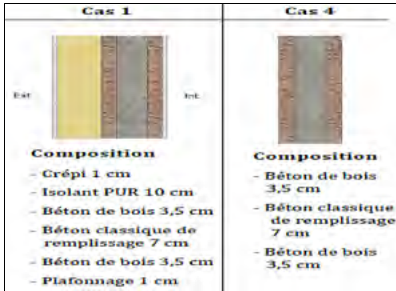
Figure 4.2 Assemblage de mur de simulation pour Lamalle et WUFI Pro 6.2; Tirée de (Lamalle, 2016), p.79)
