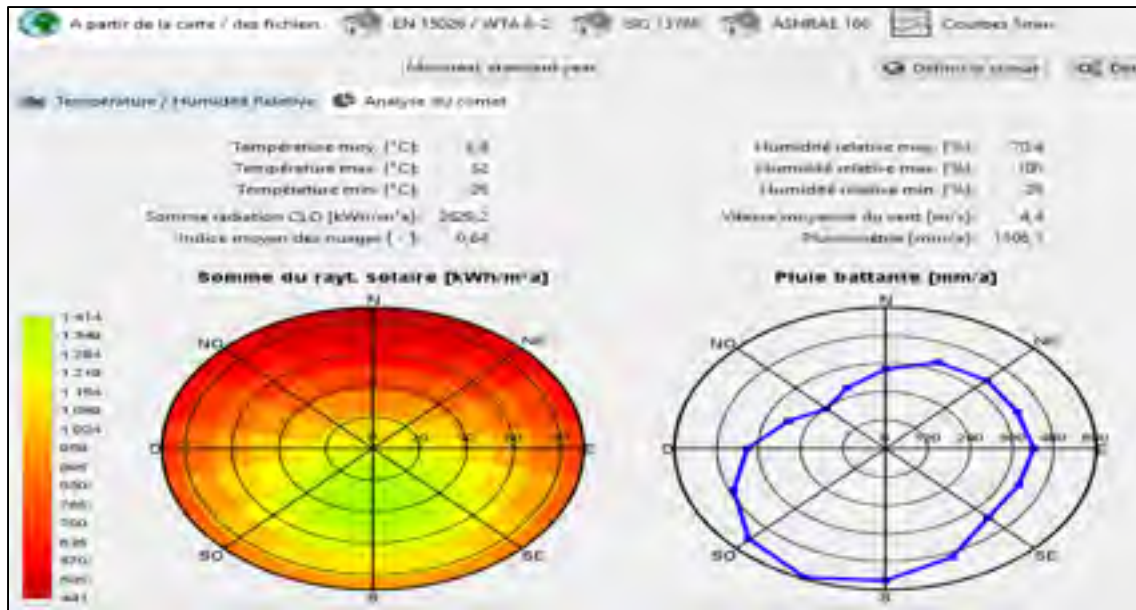
Figure A-II-5 Profil de radiation solaire et profil de la pluie battante pour la ville Montréal analysés par WUFI Pro 6.2 pour le pire cas de pluie battante et exposition de soleil
