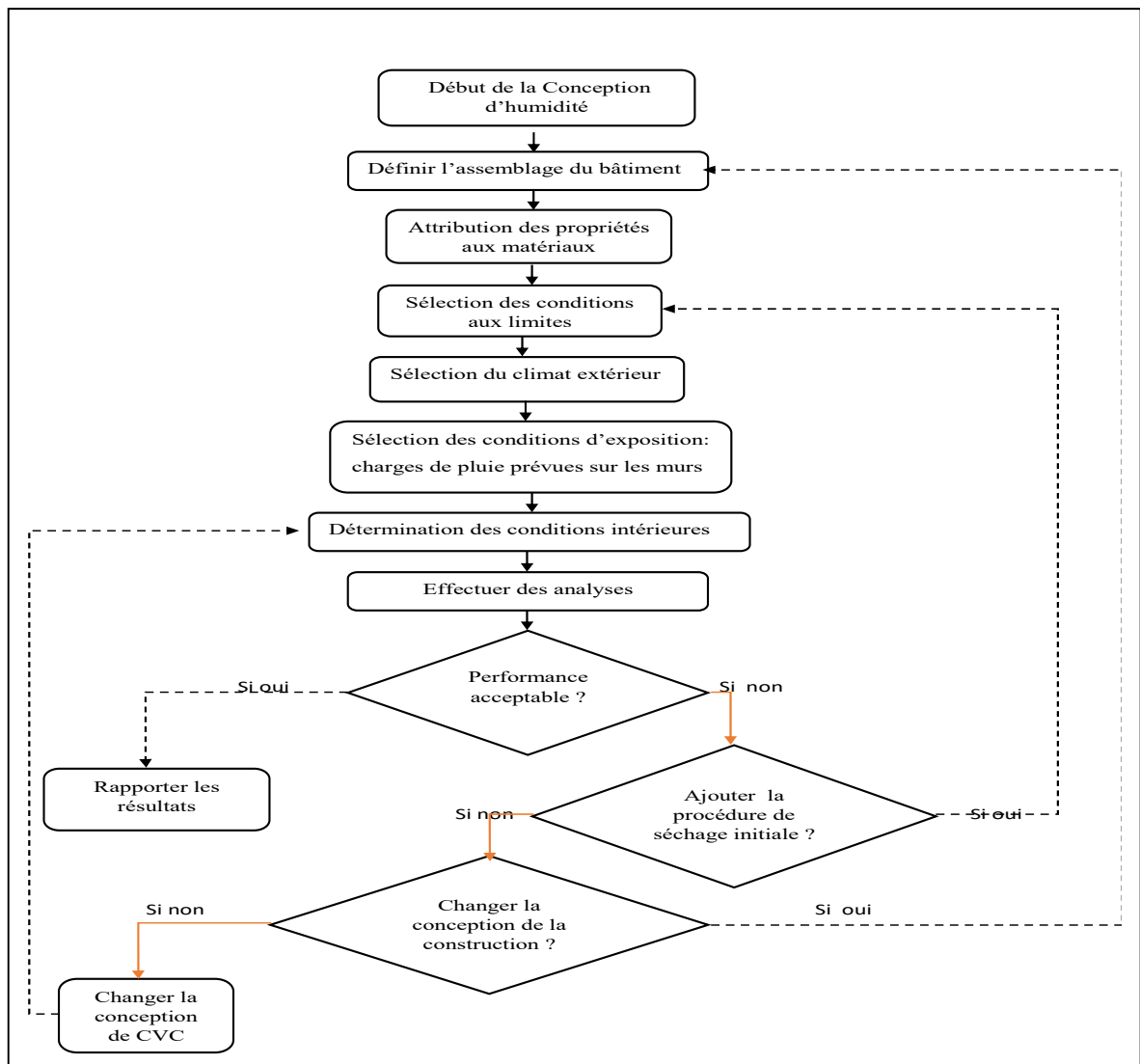
Figure 3.4 Organigramme de calcul avec la norme ANSI/ASHRAE 160
