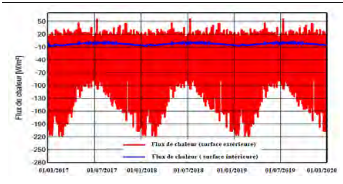
Figure-A II-32 Flux de chaleur du mur Cas 2
