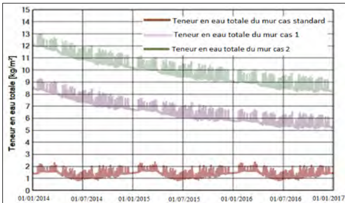
Figure 6.5 Teneur en eau totale des murs cas standard, mur 1 et mur 2 à Montréal pour un taux d'infiltration d'eau de 1 \text{ m}^3/\text{m}^2 \text{ h}
