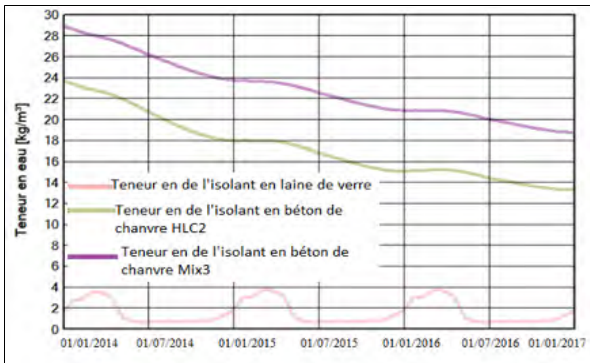
Figure 6.11 Teneur en eau de l'isolant en laine de verre, du béton de chanvre HLC2 et du béton de chanvre Mix3 pour le taux d'infiltration de 5 \text{ m}^3/\text{m}^2 \text{ h}
