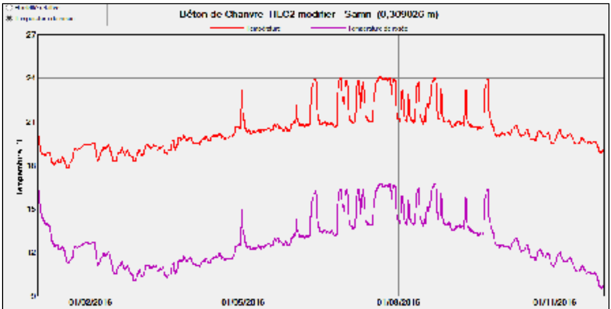
Figure-A II-22 Risque de condensation sur la surface intérieure du béton de chanvre HLC2 : 1ans un taux d'infiltration de 15\text{m}^3/\text{m}^2\text{h}
