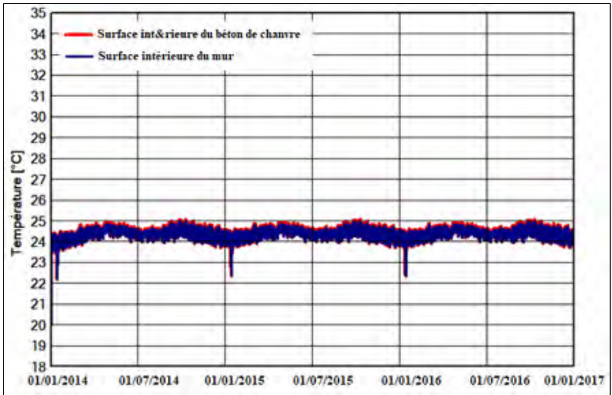
Figure-A II-27 Évolution de la température intérieure du mur en béton de chanvre pour un taux de rayonnement solaire incident de 20%
