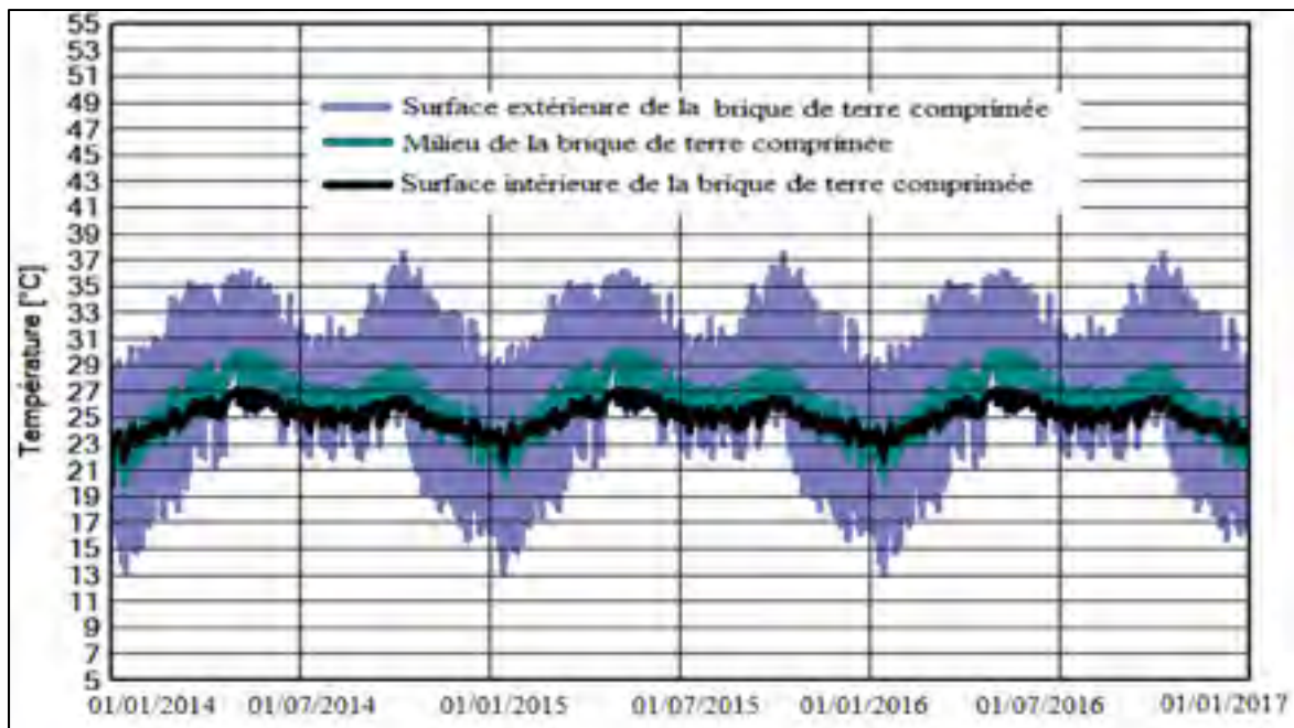
Figure 6.28 Évolution de la température dans un mur en brique de terre comprimée pour une fraction de rayonnement solaire incidente de 5 %
