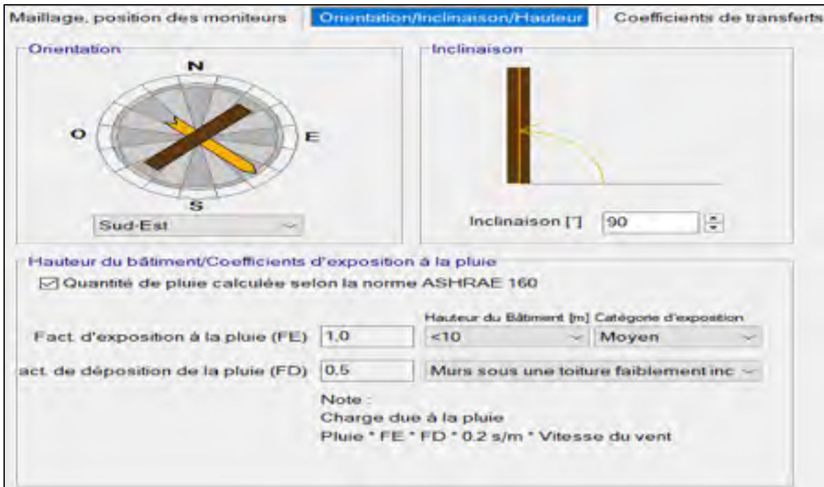
Figure-A II-8 Orientation et inclinaison des murs d'étude pour la ville de Dori
