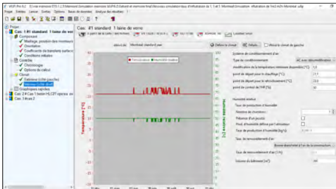
Figure-A II-15 Profil de température et du taux d'humidité intérieur de la ville de Montréal
