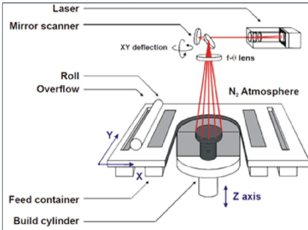
Figure 1.1 Schématisation du procédé de fusion sélective sur lit de poudre Tirée et adaptée de (Kruth et al., 2005)
