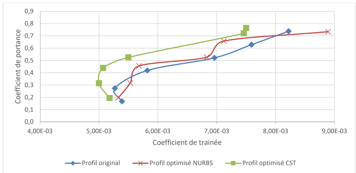
Figure 3-4 Polaires des profils modélisés par les méthodes NURBS et CST comparés à la polaire du profil original de l'UAS-S45
