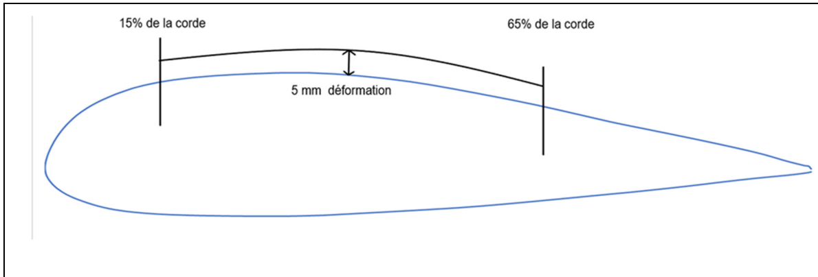
Figure 2-2 Position de la zone de déformation de l'extrados du profil de l'UAS-S45
