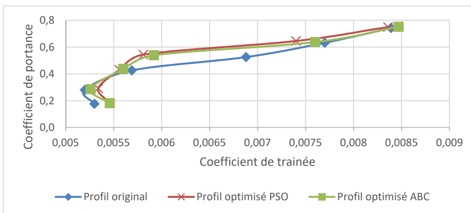
Figure 4-4 Comparaison des polaires des profils optimisés et du profil original de l'UAS-S45
