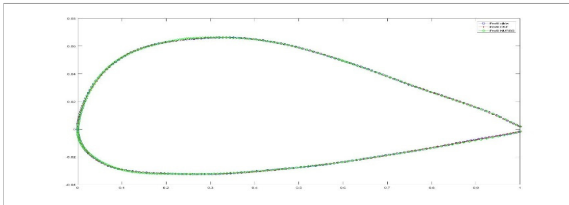
Figure 2-4 Modélisation des profils par les méthodes NURBS et CST comparées au profil original de l'UAS-S45
