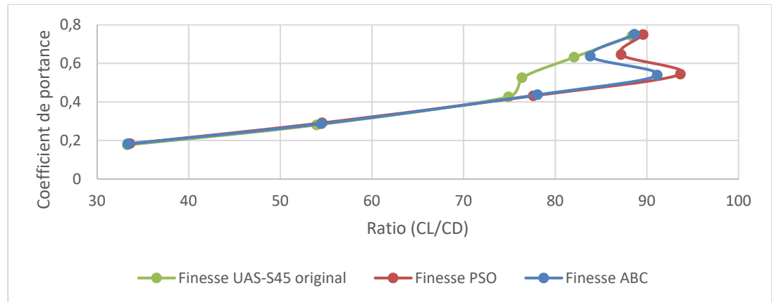
Figure 4-5 Comparaison des courbes de la finesse des profils
