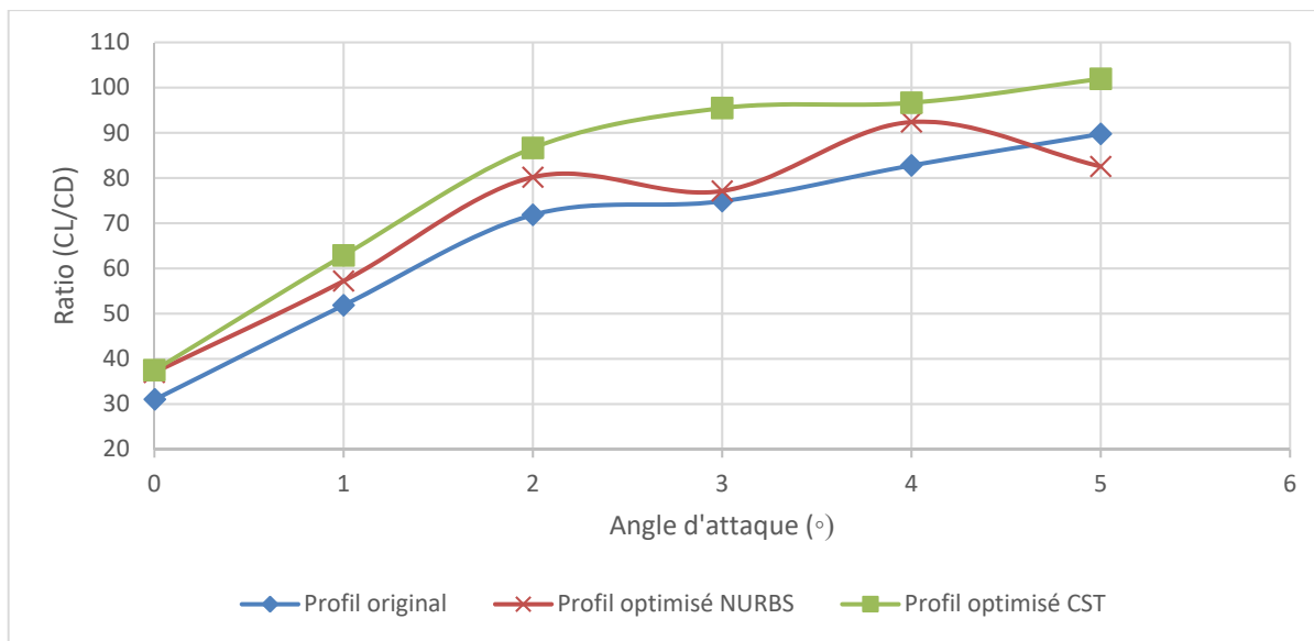
Figure 3-3 Comparaison des ratios ( C_L/C_D ) du profil original de l'UAS-S45 et des profils modélisés par les méthodes NURBS et CST
