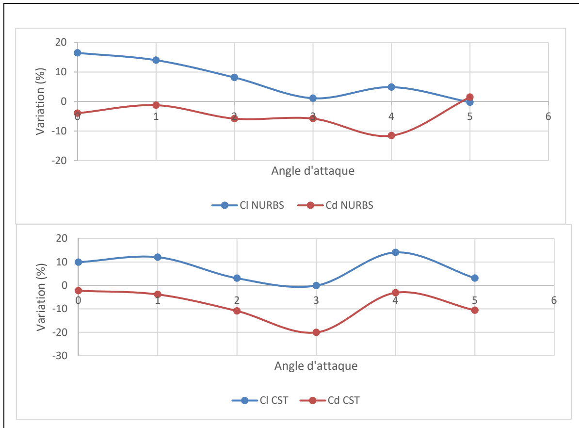
Figure 3-2 Variations des coefficients de portance et de trainée des profils optimisés par rapport au profil original en fonction de l'angle d'attaque
