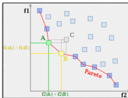
Figure 1-2 : Illustration d'un front de Pareto
