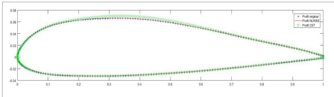
Figure 2-9 Comparaison des profils modélisés avec le profil original de l'UAS-S45 pour un angle d'attaque de 3 degrés
