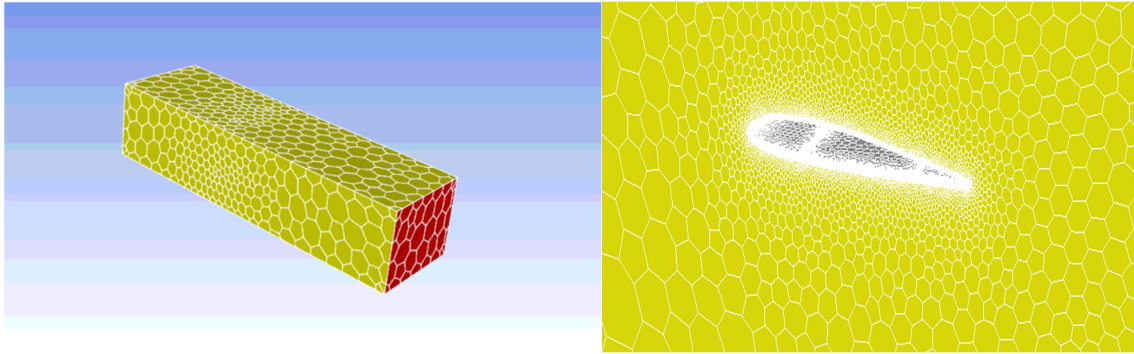
Figure 6-4 : Maillage polyédrique du domaine autour de l'aile et de l'aile
