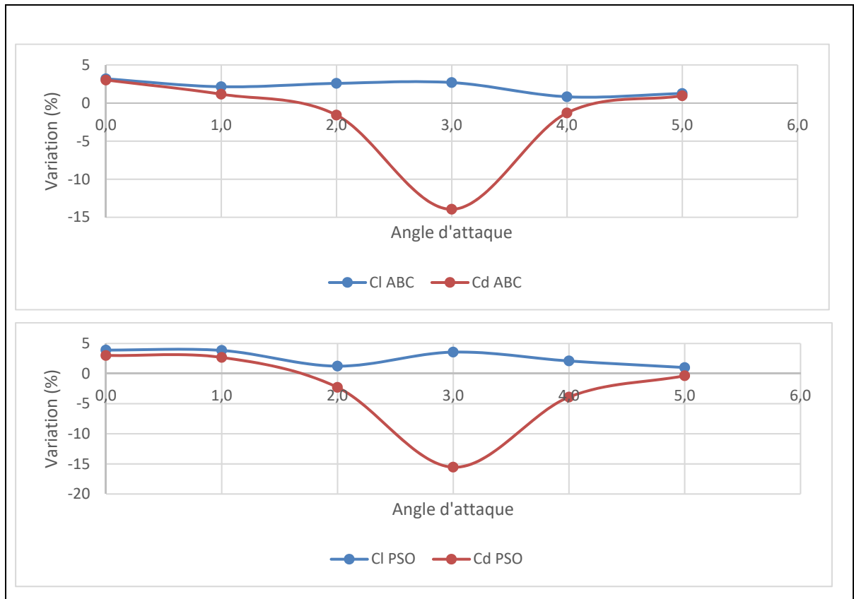
Figure 4-2 Comparaison des variations des coefficients aérodynamiques pour les deux profils optimisés
