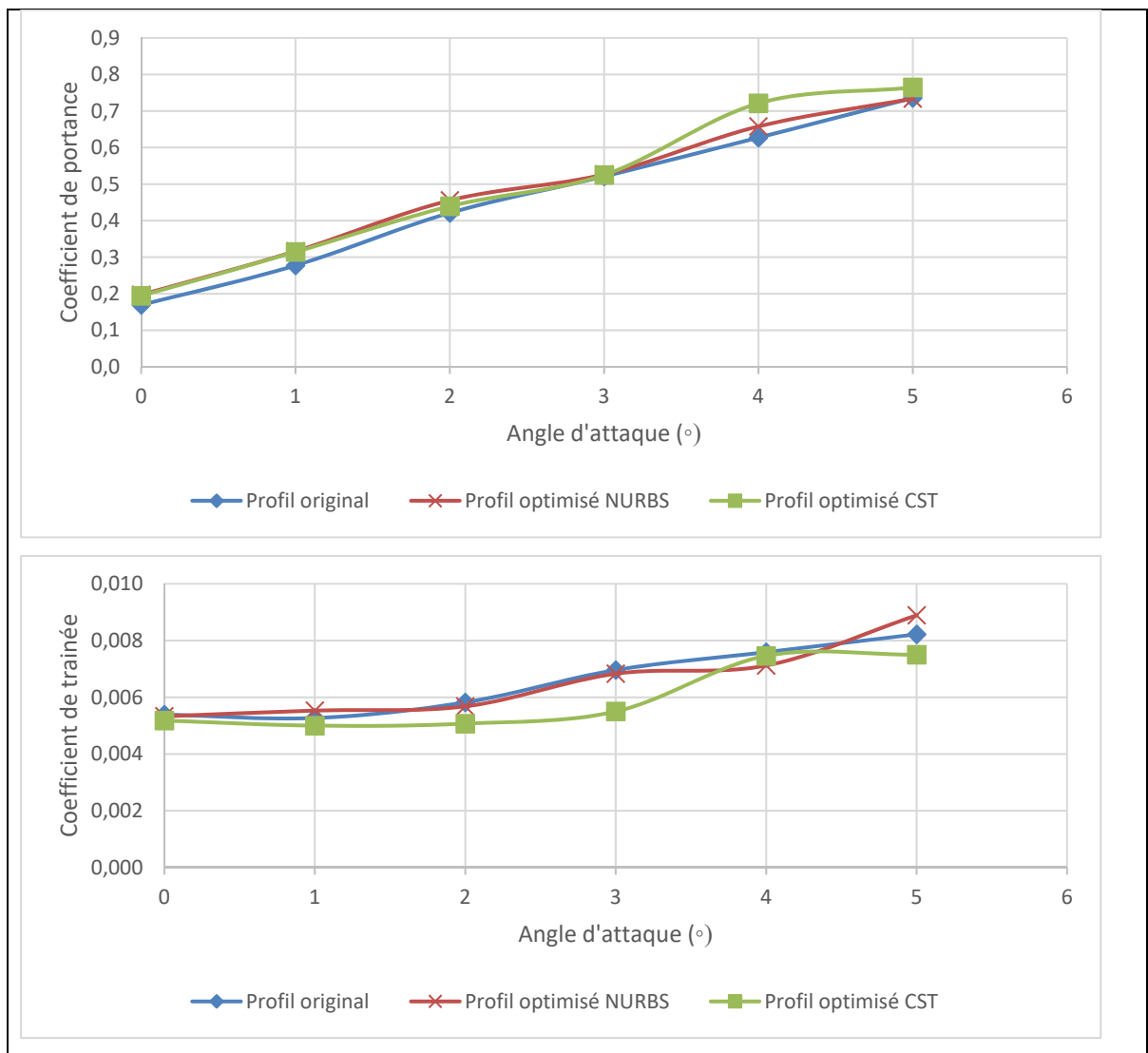
Figure 3-1 : Comparaison des coefficients de portance et de trainée des profils modélisés par NURBS et CST et du profil original de l'UAS-S45
