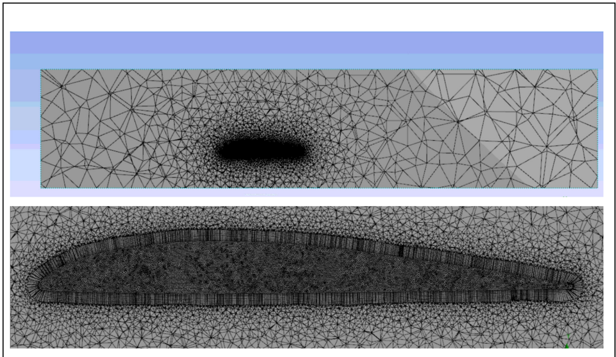
Figure 6-3 : Maillage du domaine et de l'aile avec inflation pour représenter la couche limite
