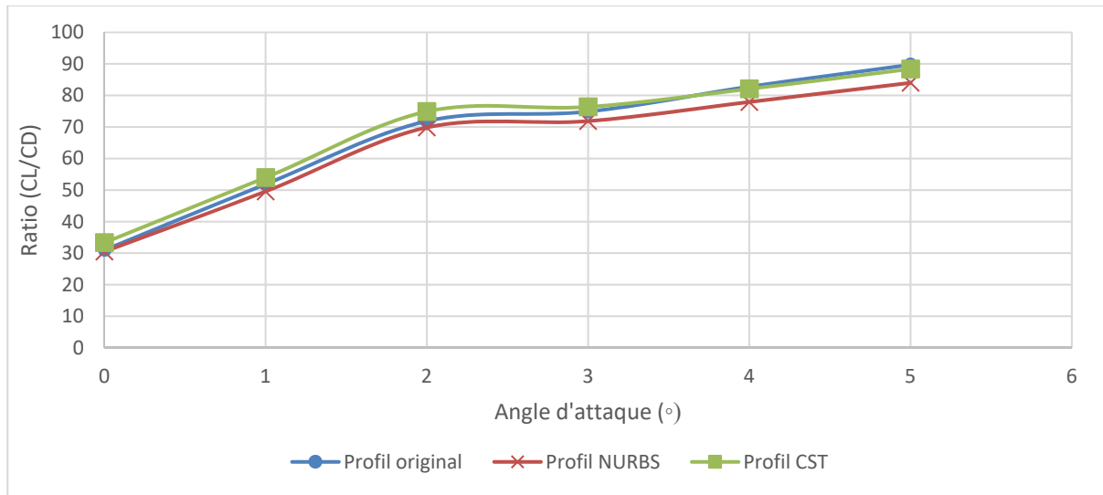
Figure 2-5 Comparaison des ratio ( C_L/C_D ) du profil original de l'UAS-S45 et des profils modélisés par les méthodes NURBS et CST
