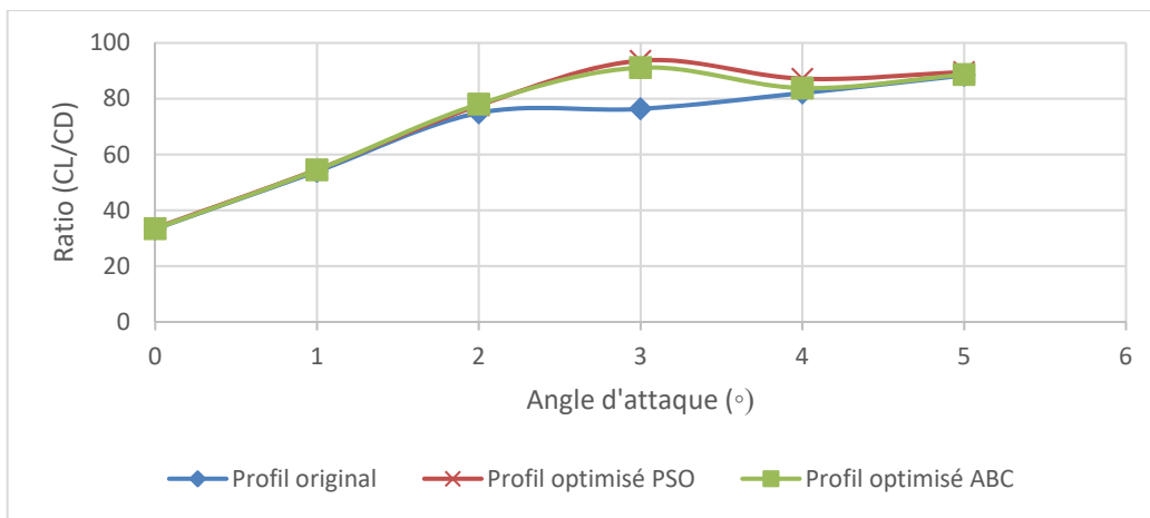
Figure 4-3 Comparaison des ratios ( C_L/C_D ) des profils optimisés et du profil original de l'UAS-S45
