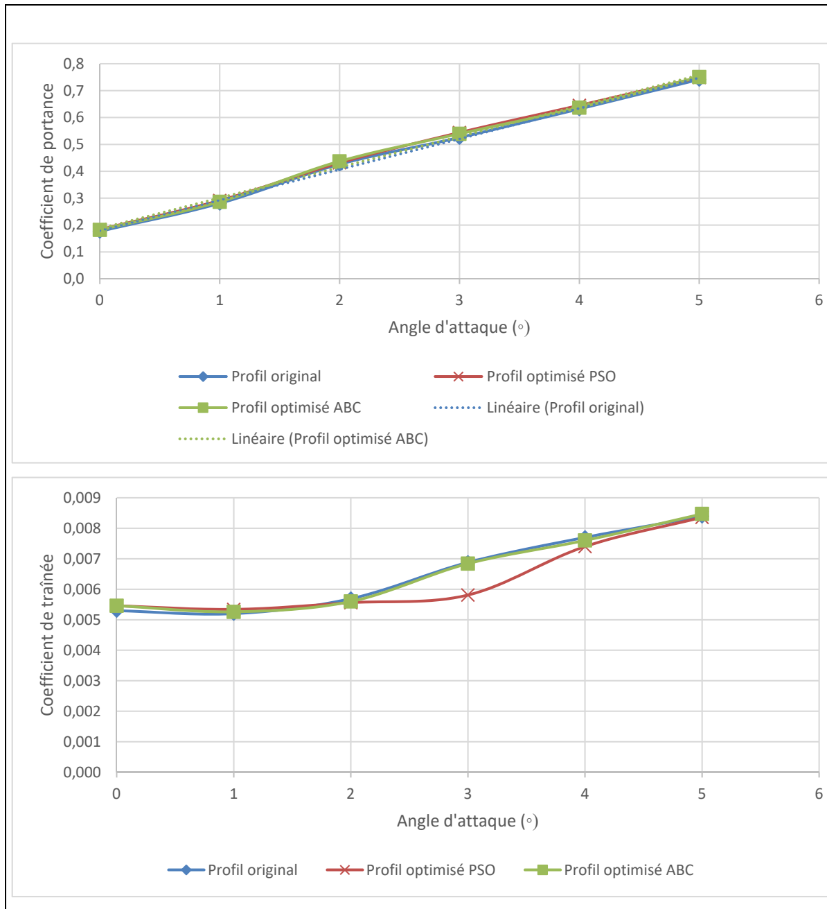
Figure 4-1 Comparaison des coefficients de portance et de trainée pour les profils optimisés par les algorithmes ABC et PSO ainsi que le profil original de l'UAS-S45
