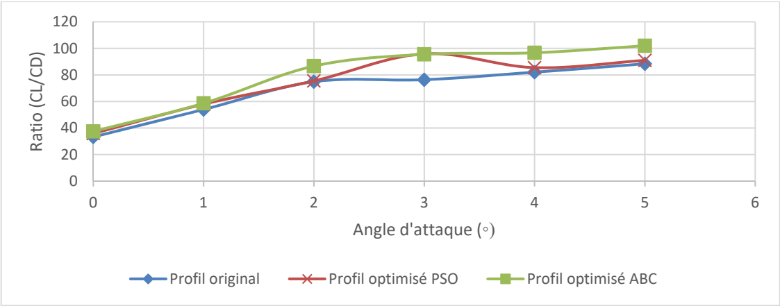
Figure 5-3 Comparaison des ratios (CL/CD) en fonction de l'angle d'attaque pour les trois profils
