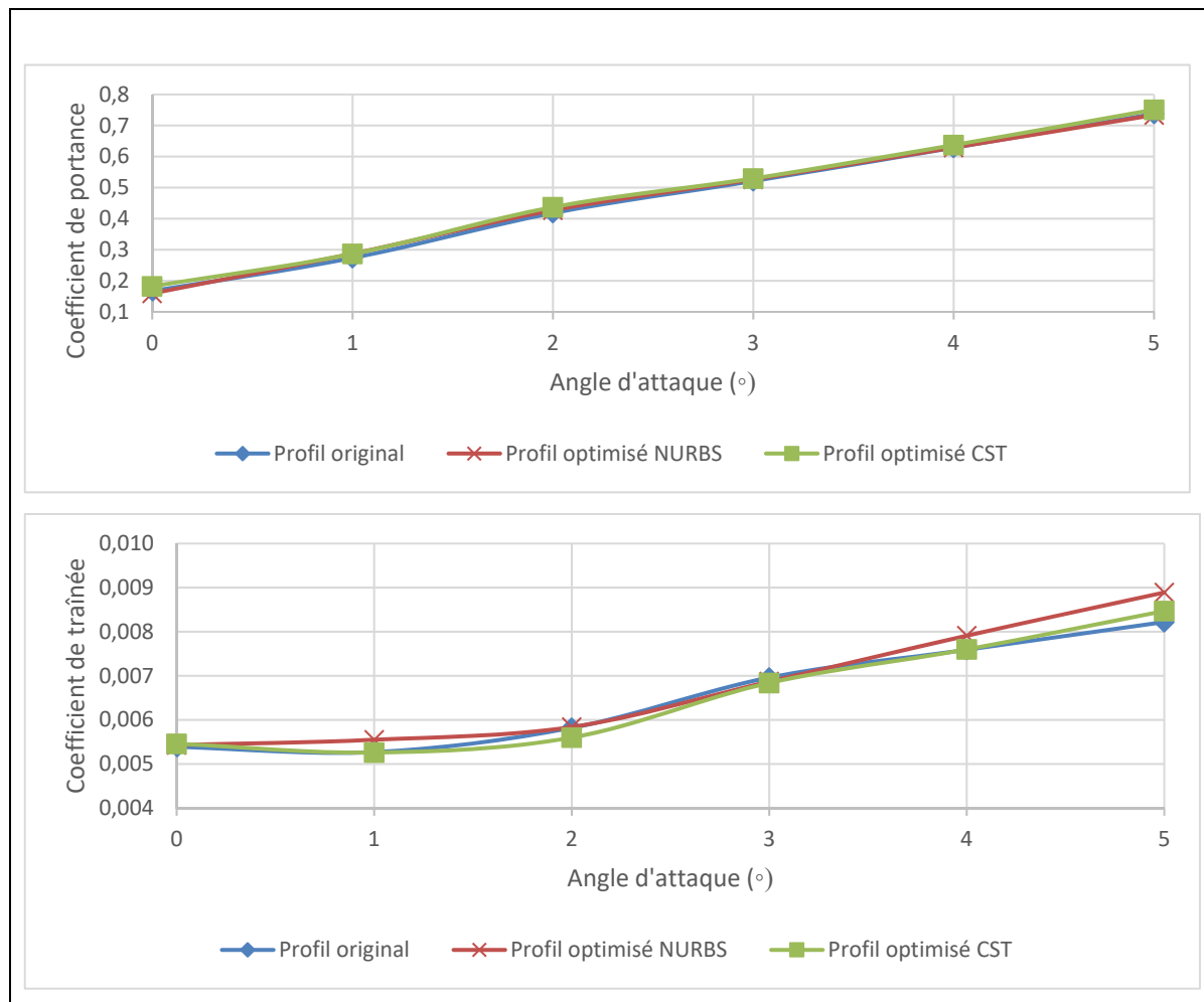
Figure 2-6 Comparaison des coefficients de portance et de traînée du profil original et des profils optimisés représentés par les méthodes NURBS et CST
