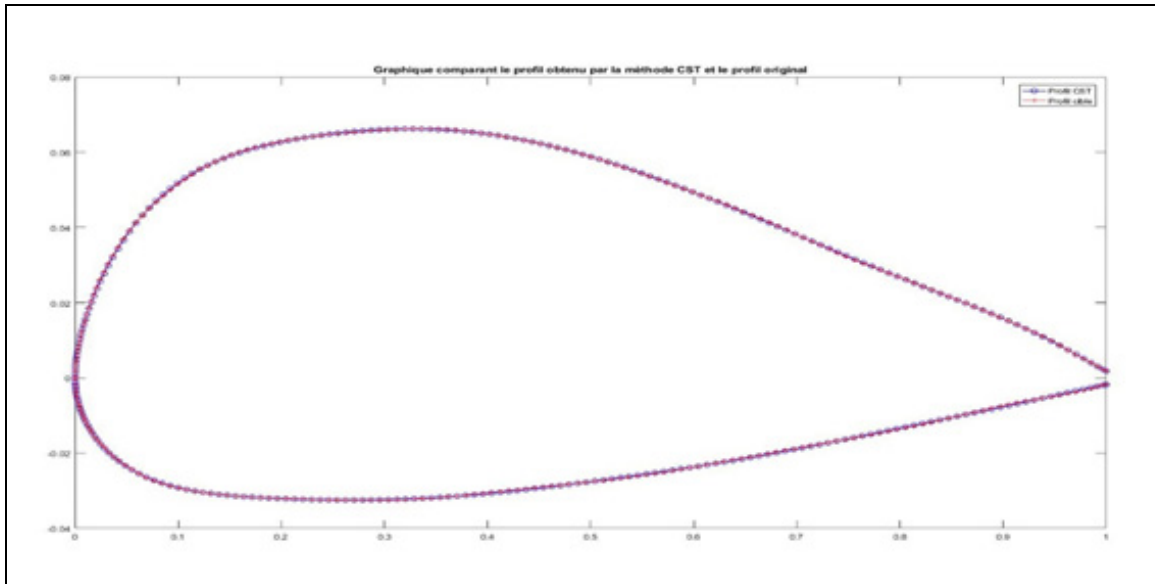
Figure 2-1 Graphique illustrant le profil original et le profil original modélisé par la méthode CST
