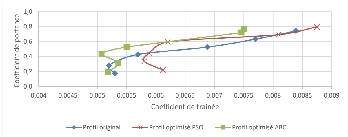
Figure 5-4 Comparaison de la polaire des profils optimisés et du profil original de l'UAS-S45
