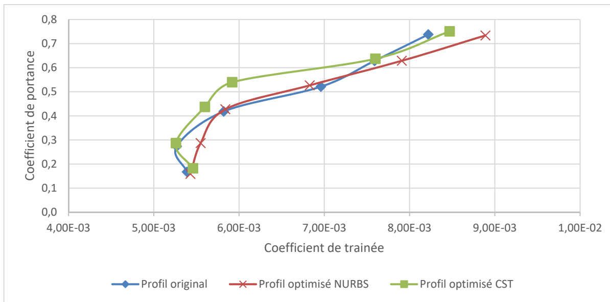
Figure 2-8 Comparaison des polaires du profil d'origine de l'UAS-S45 et des profils optimisés modélisés par les méthodes NURBS et CST
