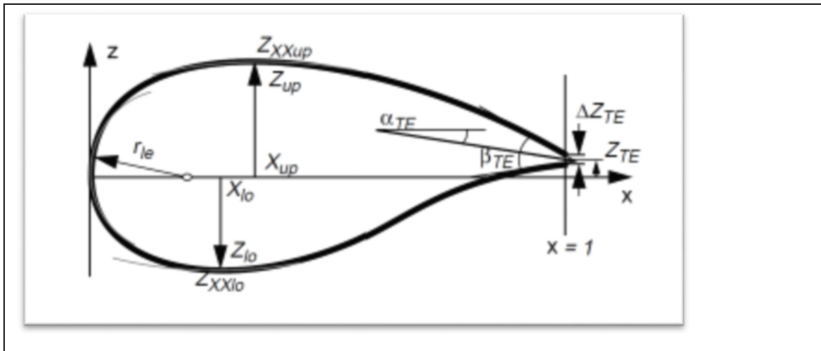
Figure 1-2 : Représentation géométrique des paramètres utilisés dans la méthode PARSEC
