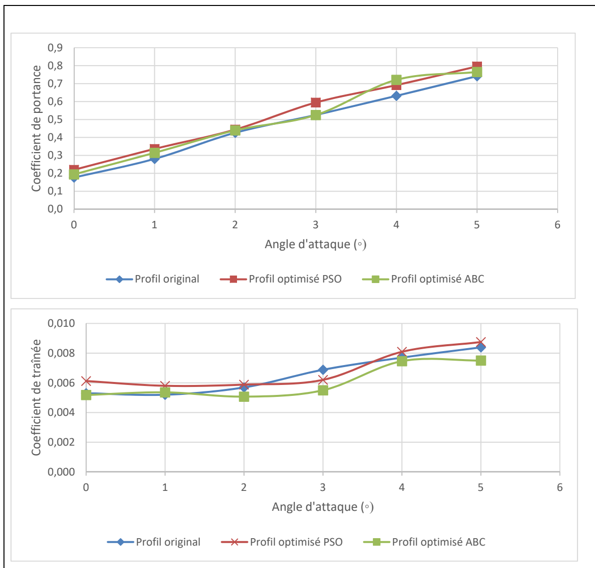
Figure 5-1 Comparaison des coefficients de portance et de traînée pour les deux profils optimisés et le profil de l'UAS-S45
