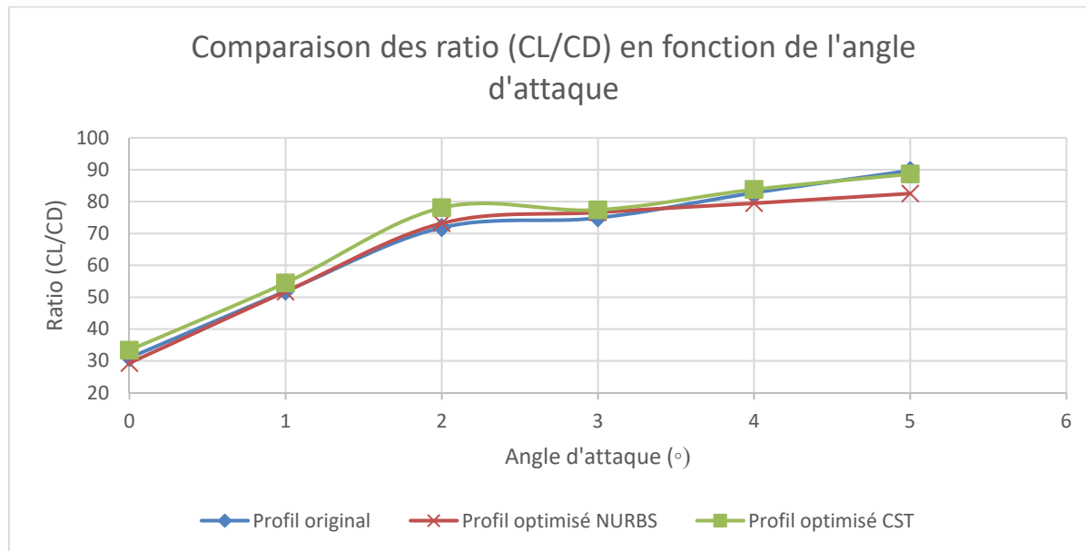
Figure 2-7 Comparaison des ratio ( C_L/C_D ) en fonction de l'angle d'attaque pour le profil original de l'UAS-S45 et les profils modélisés par les méthodes NURBS et CST et optimisés par l'algorithme ABC
