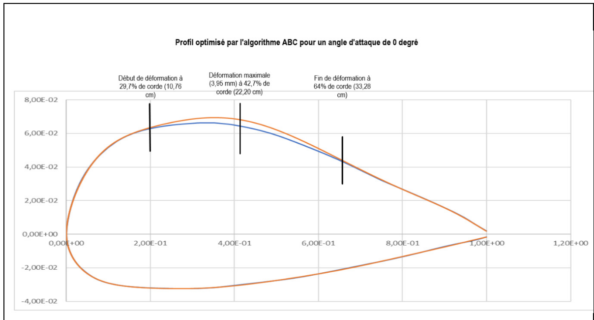
Figure 6-5: Exemple des côtes des déformations d'un profil optimisé par rapport au profil original
