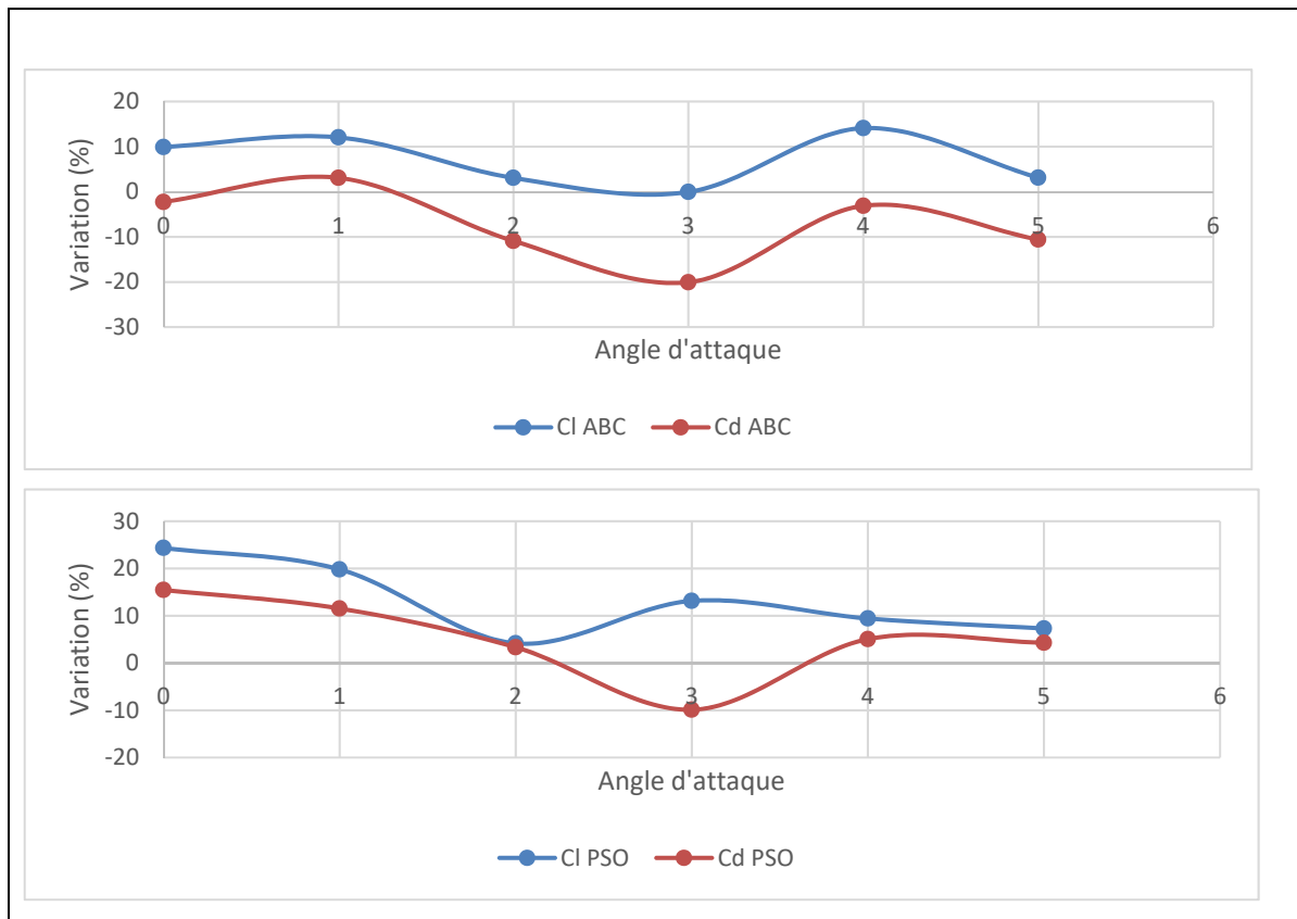
Figure 5-2 Variation des coefficients de portance et traînée pour chacun des profils optimisés par rapport au profil original en fonction de l'angle d'attaque
