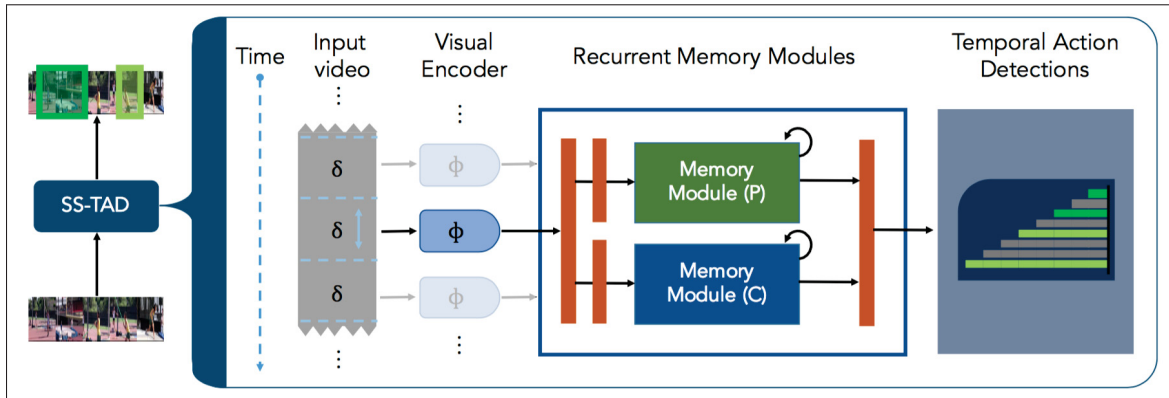
Figure 1.8 Modèle de détection d'activités à flux unique. SS-TAD : Single Stream-Temporal Action Detection . P : Proposal. C : Classification Tirée de Buch et al. (2017a)
