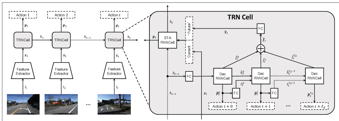
Figure 1.9 Modèle récurrent temporel prédictif. TRN : Temporal Recurrent Network .
