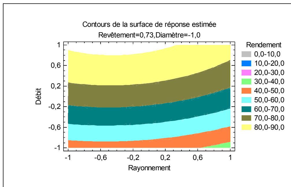
Figure 6.15 Contours de surface de réponse débit-rayonnement.
