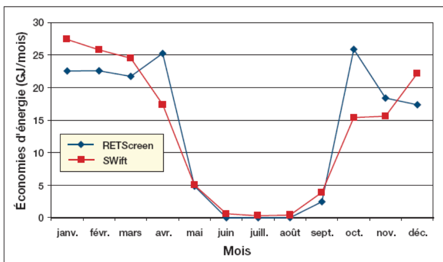
Figure 2.5 Comparaison des économies d'énergie annuelles calculées par RETScreen et Swift (bâtiment industriel, Toronto).
