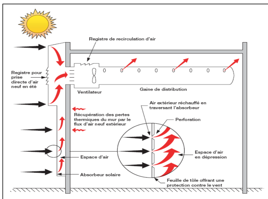
Figure 3.2 Représentation schématique d'un système de chauffage solaire de l'air. Tirée de (RETScreen, 2009)
