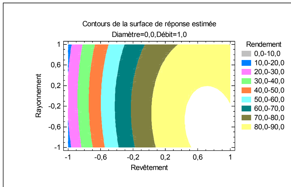
Figure 6.14 Contours surface de réponse revêtement-rayonnement.
