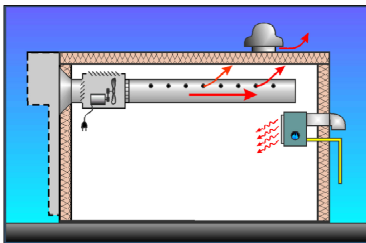
Figure 3.5 Projet CSA sur un bâtiment industriel. Tirée de (RETScreen, 2009)
