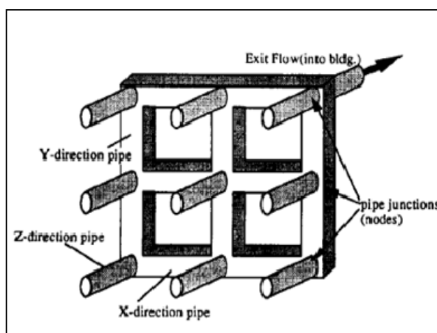
Figure 2.6 Réseau de conduites fictives développées par Dymond et Kutscher. Tirée de (Dymond et Kutscher, 1997).
