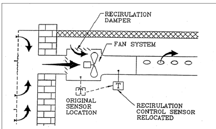
Figure 3.3 Système de contrôle de la température. Tirée de (Shc. IEA, 1999)
