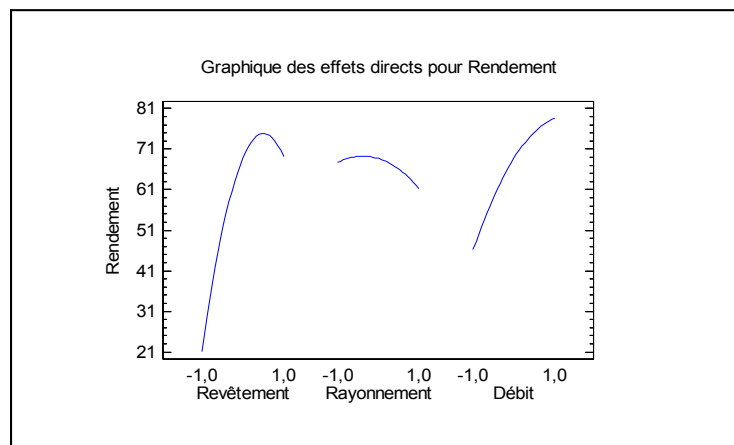
Figure 6.8 Graphique des effets principaux pour le rendement.
