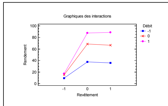
Figure 6.9 Effet d'interaction revêtement-débit.
