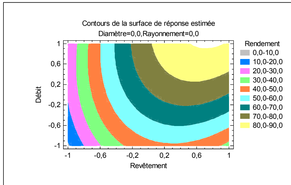
Figure 6.13 Contours surface de réponse revêtement-débit.
