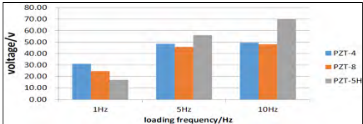
Figure 3.3 Comparaison du voltage sous 1000N de charge de pointe pour les trois PZT Tirée de X.Xu et al (2018, p391)
