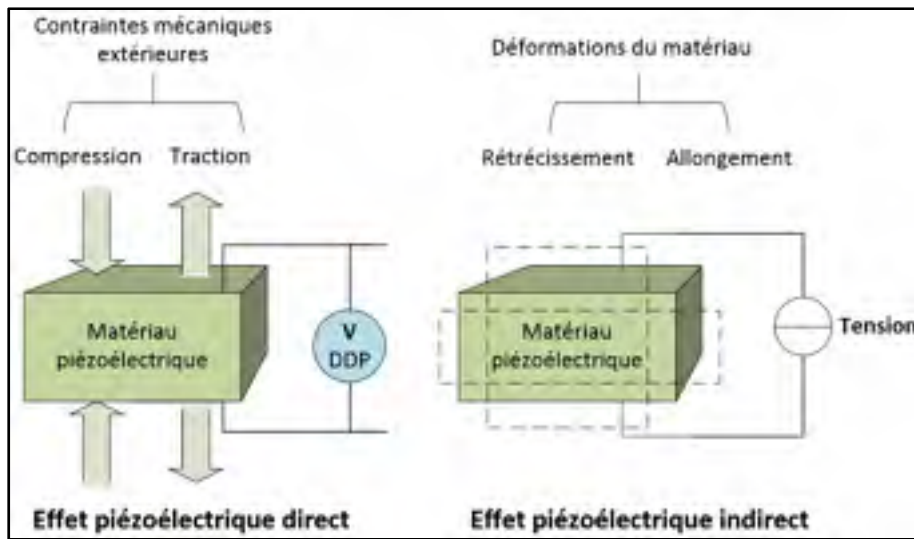
Figure 1.25 Effets piézoélectriques
