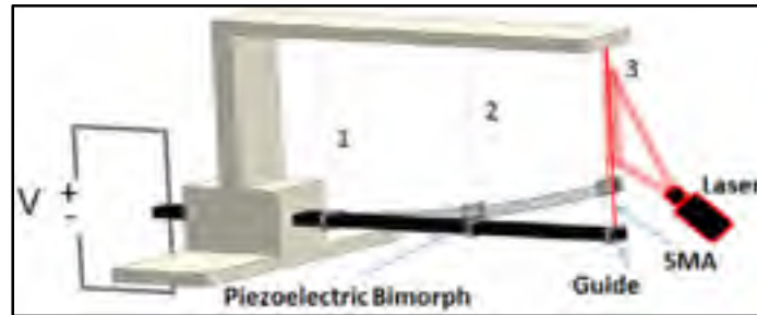
Figure 1.33 Générateur thermomécanique (SMA) à transduction piézoélectrique Tirée de Avirovik et al (2013, p2)
