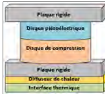
Figure 2.5 Composition finale du générateur proposé
