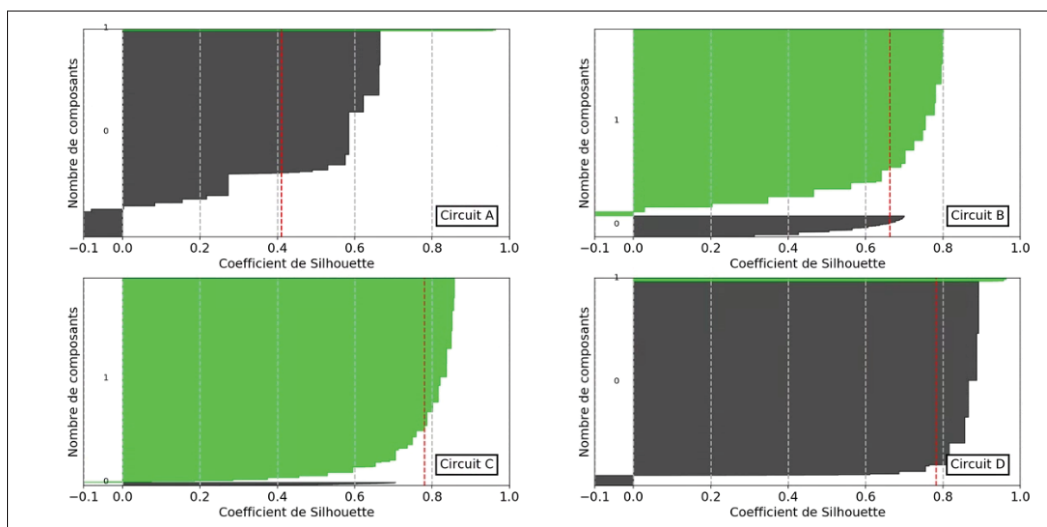
Figure 3.6 Représentation des coefficients de silhouette en fonction du nombre de composantes pour les circuits sélectionnés
