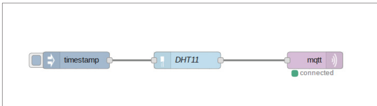
Figure 3.33 Flux de données de l'objet DHT11 dans le cas des objets distribués
