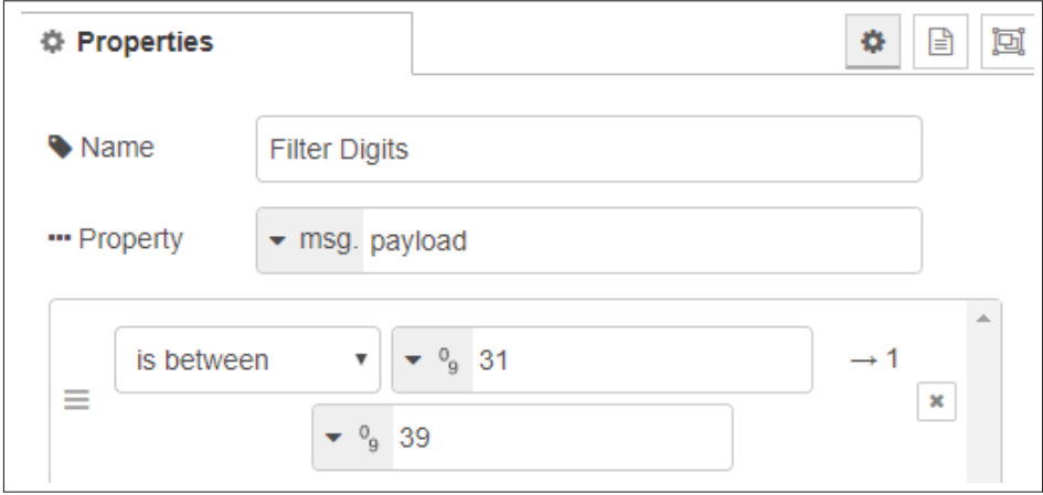
Figure 3.22 Nœud FilterDigit
