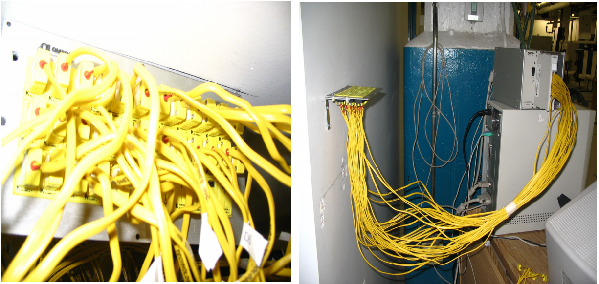
Figure II.5 Connexion des thermocouples vers l'ordinateur.
