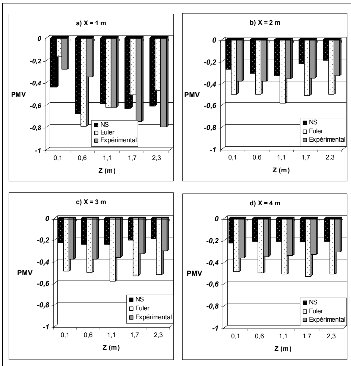
Figure 5.6 Indice PMV en fonction de la hauteur ( y=1,83 m).
