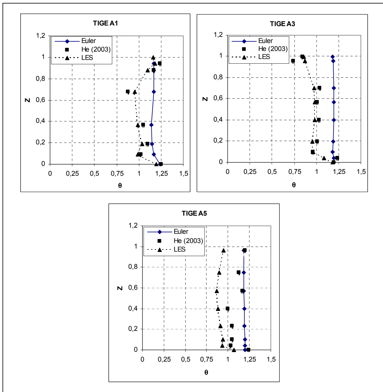
Figure 6.3 Rapport de température en fonction de la hauteur pour la ventilation par mélange ( T_s=18,5\text{ }^{\circ}\text{C} ; T_e=24,16\text{ }^{\circ}\text{C} ; H=2,26\text{ m} ).
