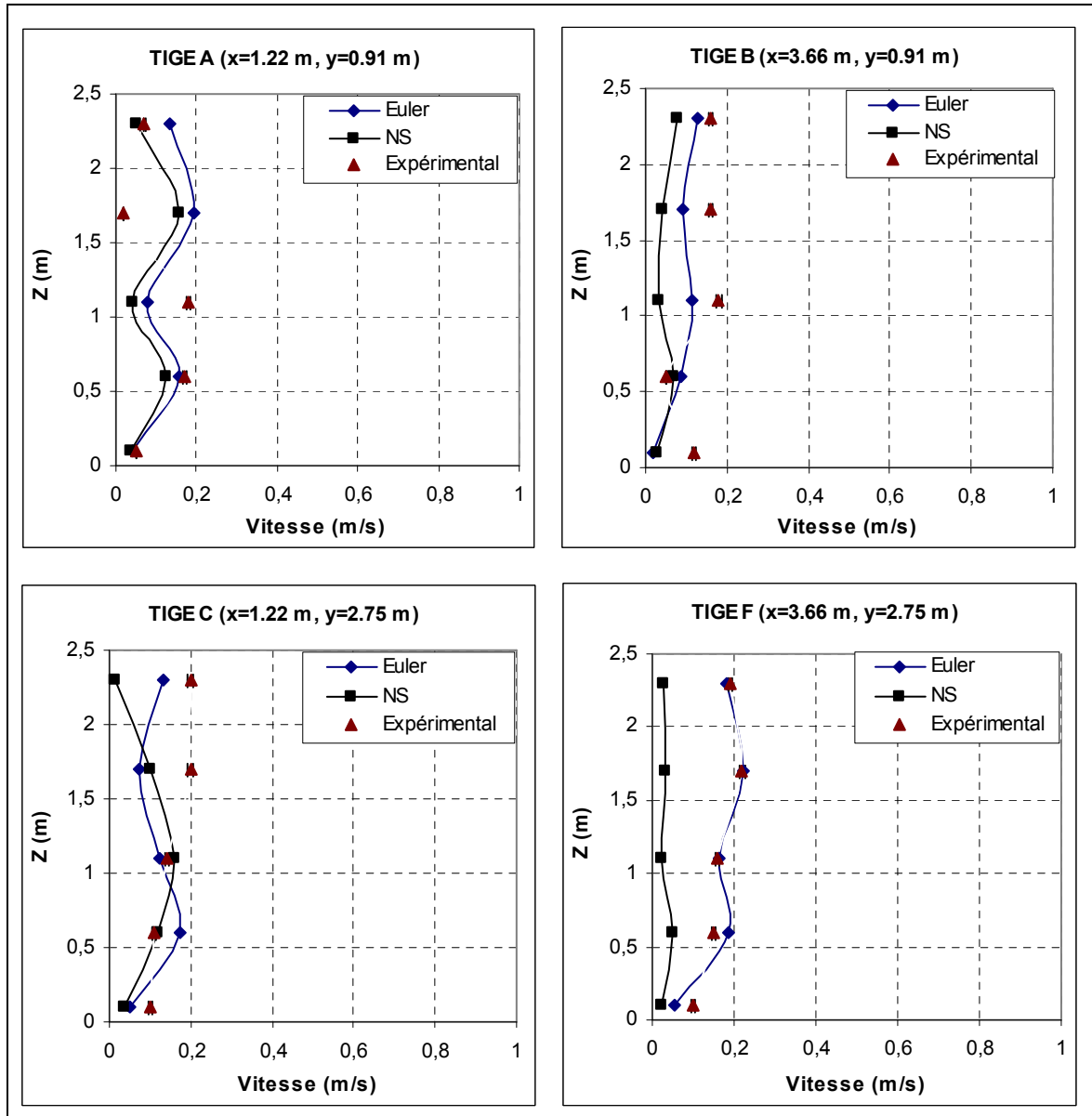
Figure 5.12 Distribution des vitesses d'écoulement pour le cas de climatisation.
