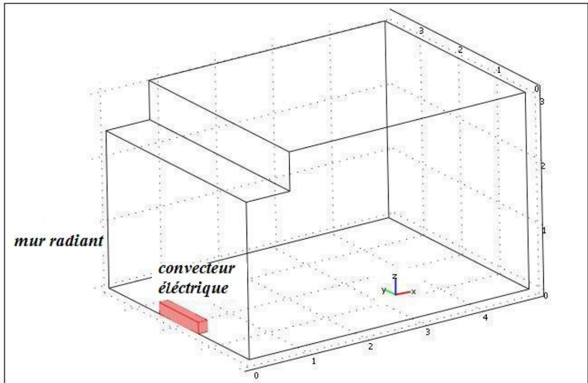
Figure 4.1 Schéma de la chambre climatique pour le cas de chauffage par convection naturelle.
