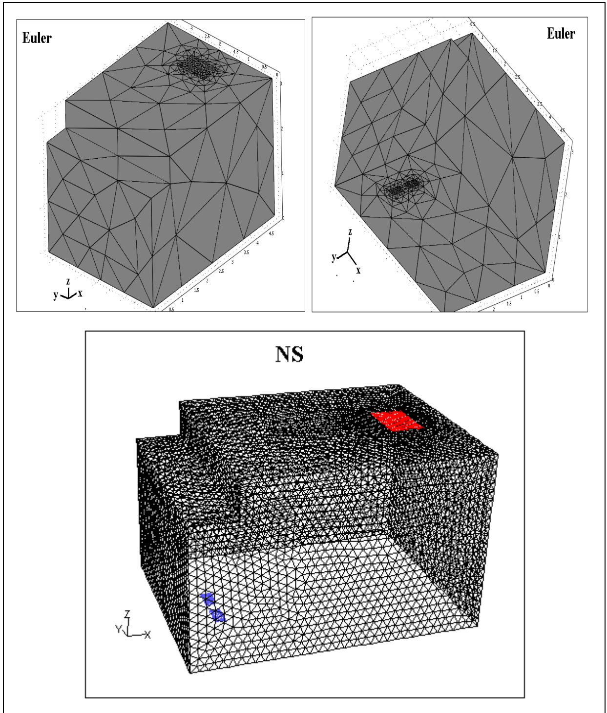
Figure 5.2 Maillage pour le cas de chauffage et ventilation par le plancher.
