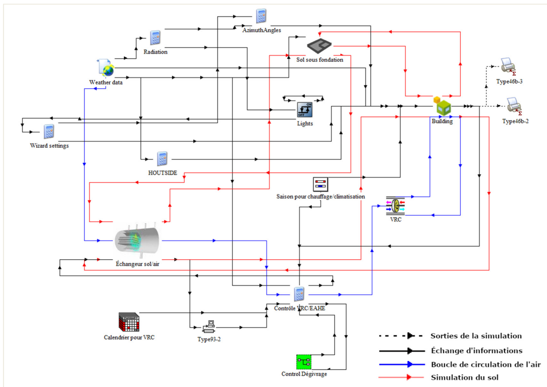
Figure 2.7 Schéma de la simulation sous TRNSYS
