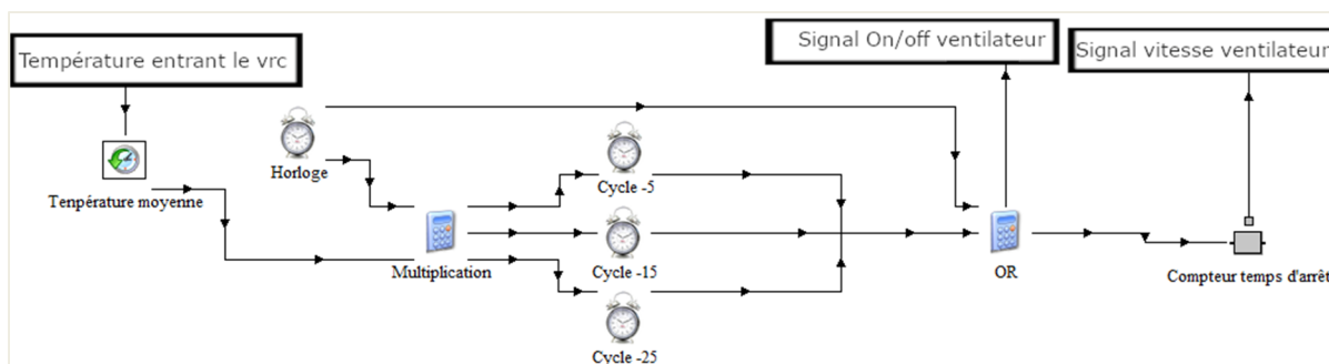
Figure 2.4 Commande des cycles de dégivrage
