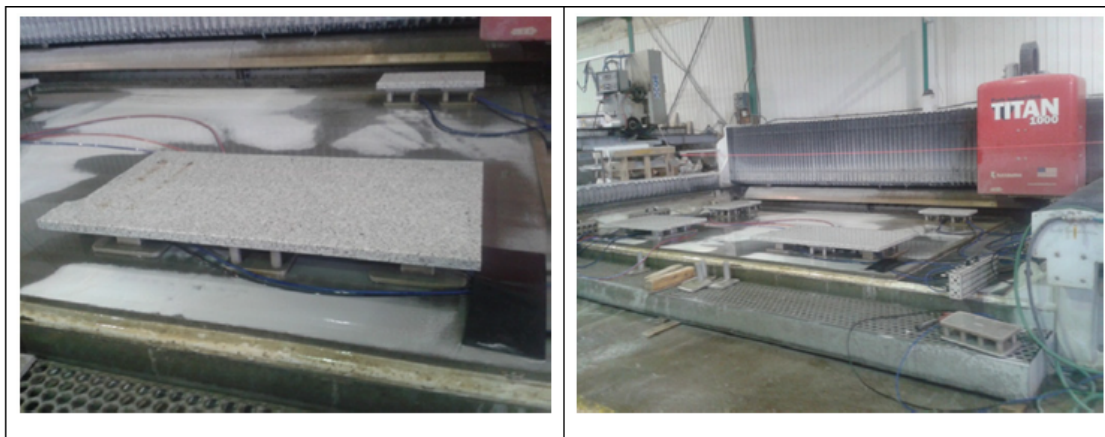
Figure 2.1 Polissage des blocs de granit à l'aide d'une machine à commande numérique Titan 1000 tiré de Migan (2015)
