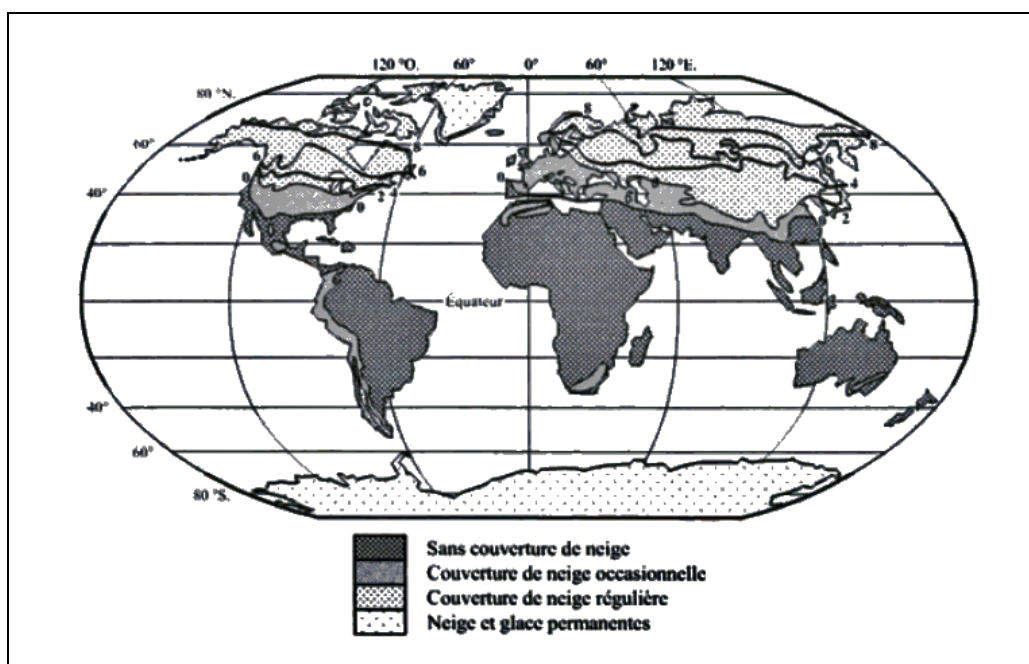
Figure 1.2 Répartition géographique des couverts neigeux et durée de vie. Tirée d'Anctil et al. (2005, p. 82)
