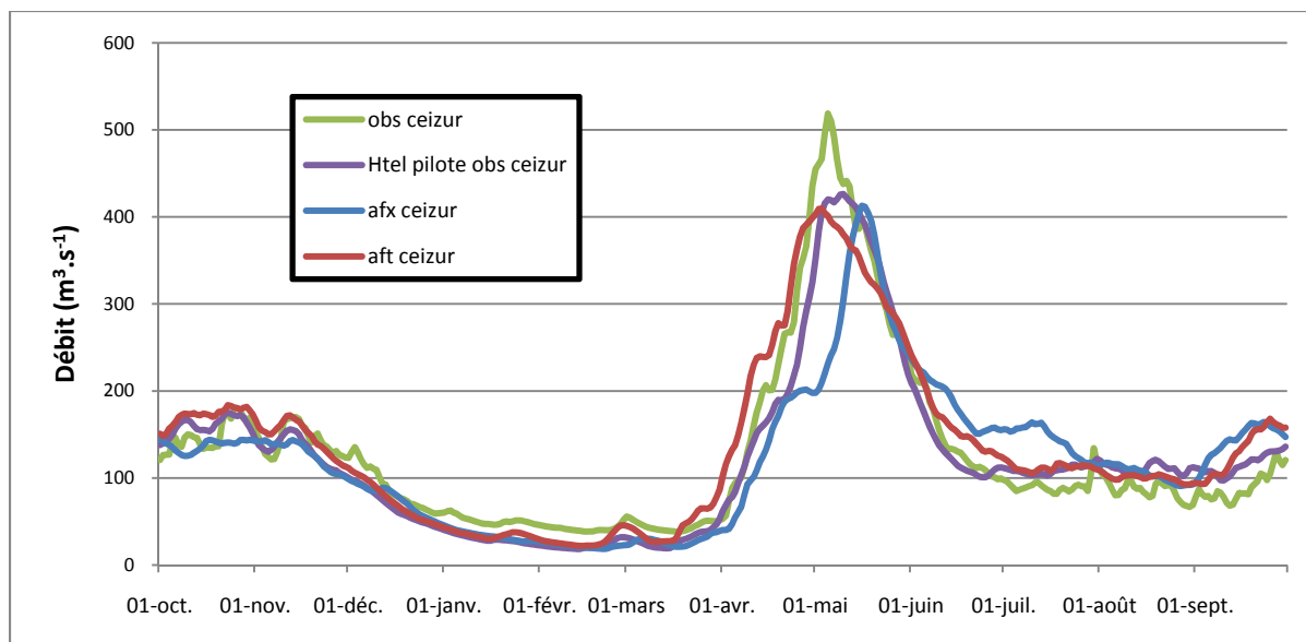
Figure 6.8 Hydrogrammes moyens observés et produits par Hydrotel sous plusieurs options de pilotage à l'endroit du sous-bassin Ceizur et pour l'horizon 1980-1997.
