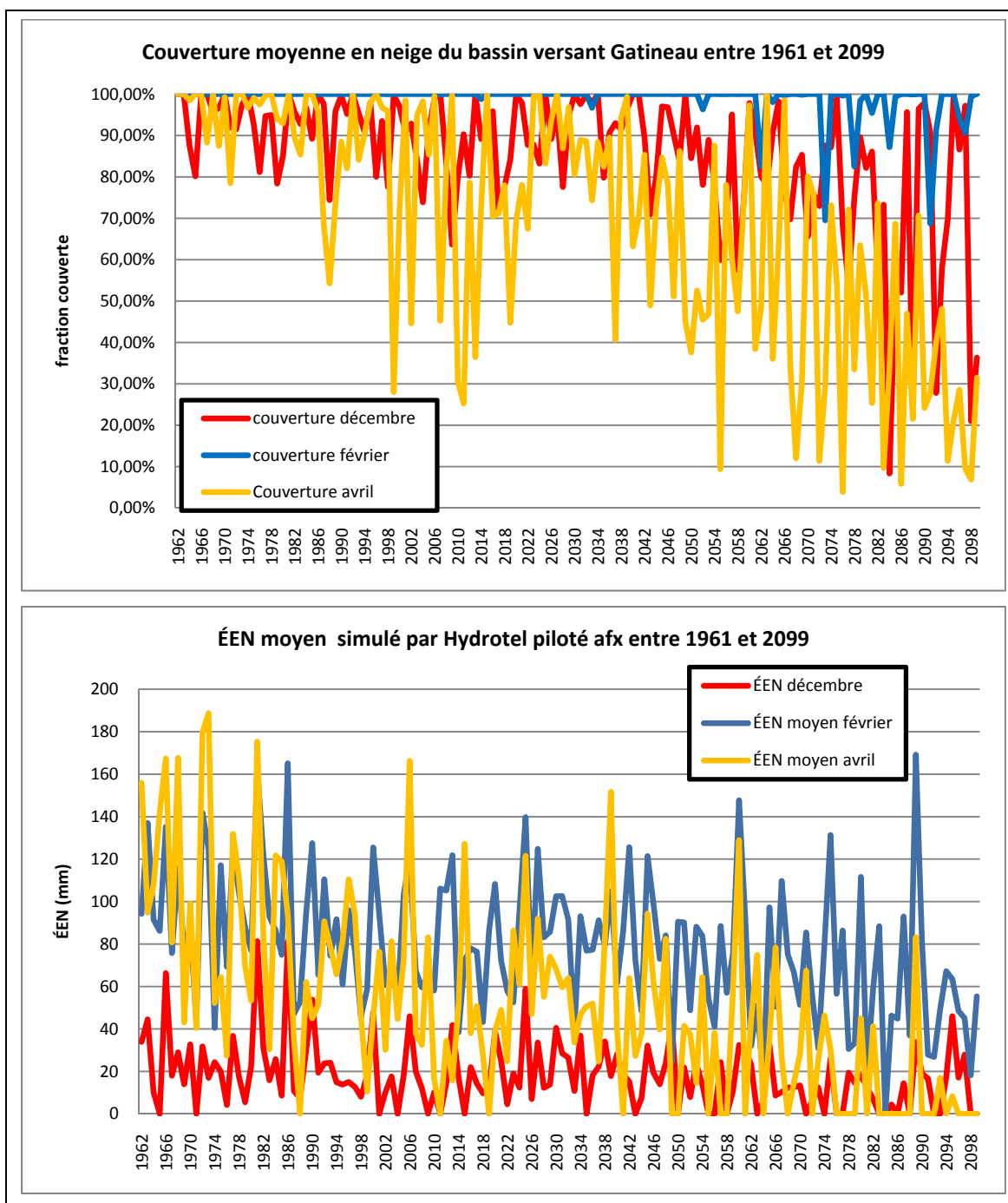
Figure 5.25 Évolutions de l'ÉÉN moyen (bas) et de la fraction couverte par la neige (haut) moyennées sur les mois de décembre, février et avril telles que simulées par Hydrotel piloté afx entre 1961 et 2099.
