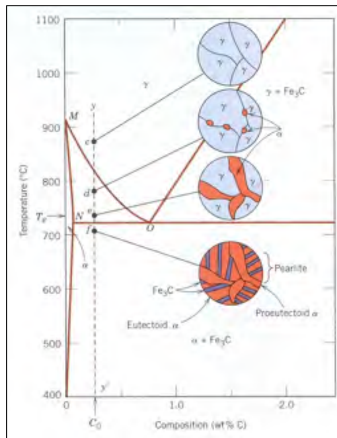
Figure 1.7 Diagramme des phases Fer-Carbone avec les microstructures stables associées pour un alliage hypoeutectoïque. Tirée de Callister et Rethwisch (2008, p. 386)
