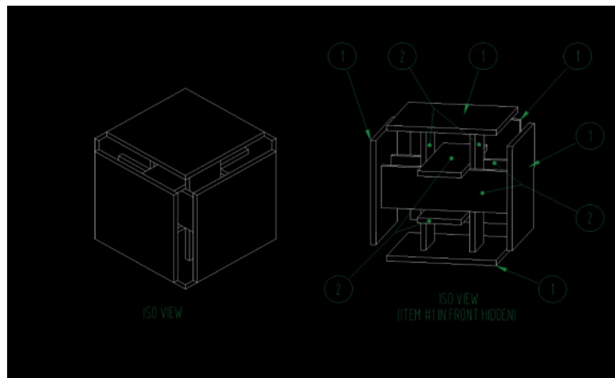
Figure 5.2 Vue isométrique de l'enveloppe mécanique
