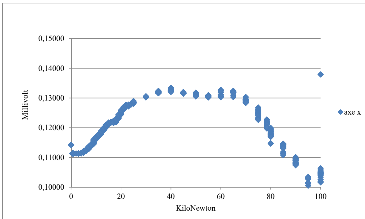
Figure 5.27 Acquisition statique des données sur le capteur nommé X (Les résultats sont mV sur l'axe des y et kN sur l'axe des x)
