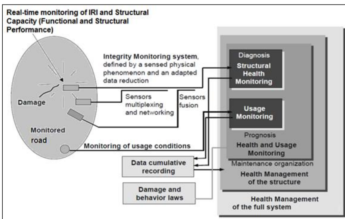
Figure 2.9 Diagnostic, pronostic et gestion du système (Balageas dans OWI, 2013)
