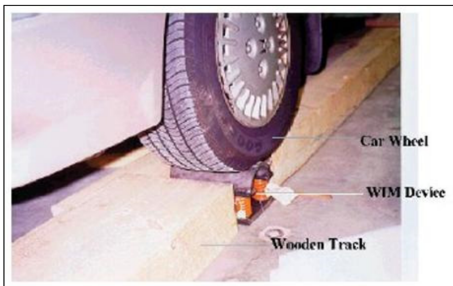
Figure 3.23 WIM avec fibre optique (Malla, 2000)
