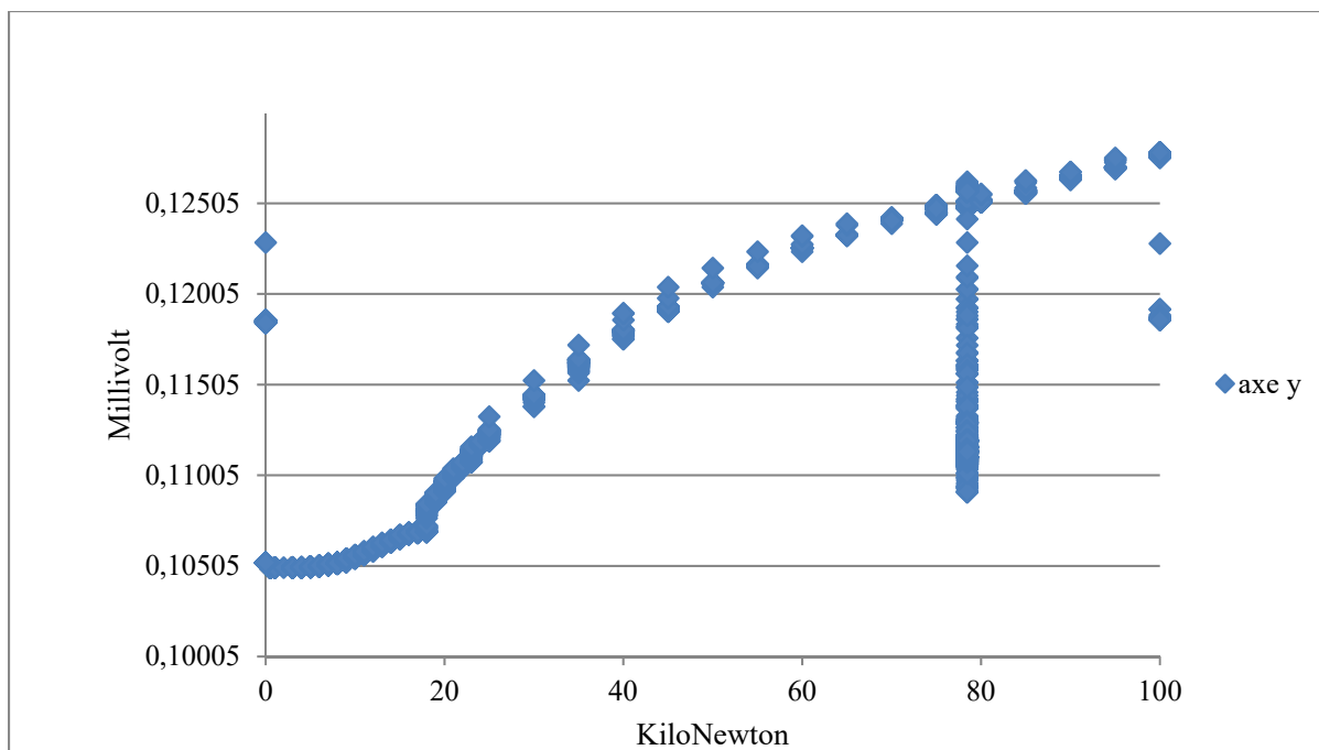
Figure 5.28 Acquisition statique des données sur le capteur nommé Y
