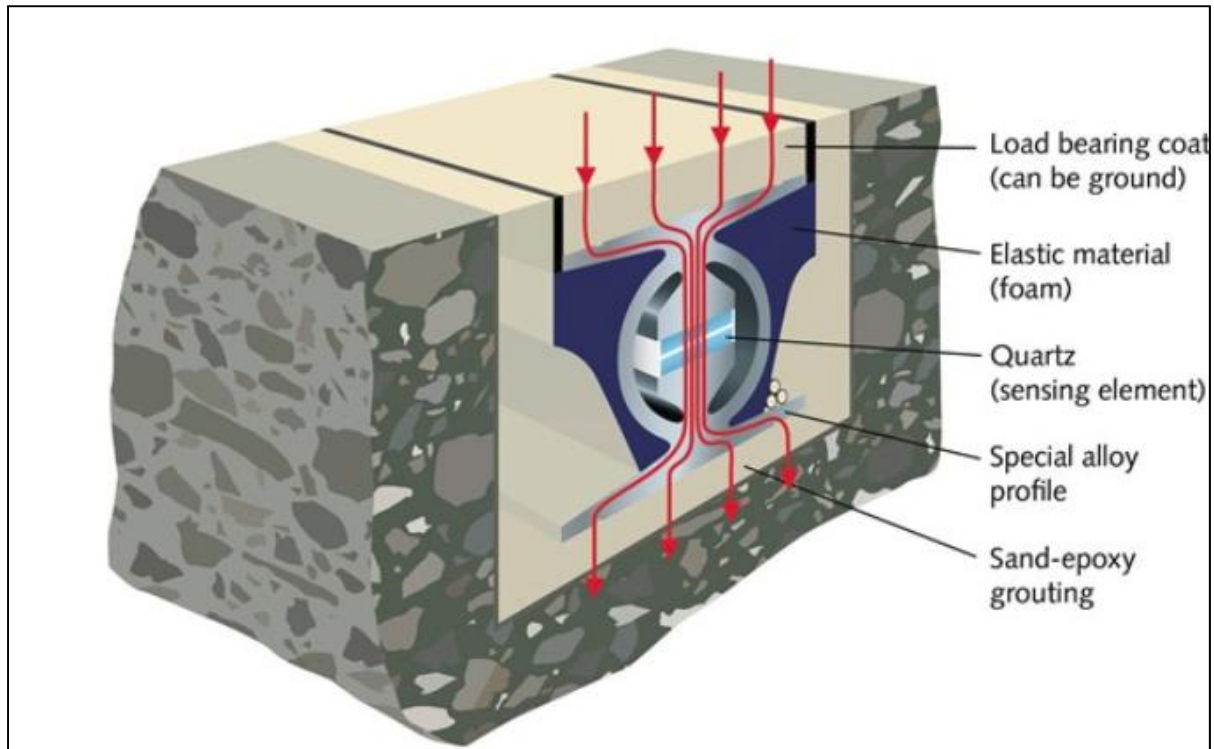
Figure 3.15 système WIM qui utilise un capteur piézoélectrique (https://www.kistler.com/en/glossary/term/wim/)
