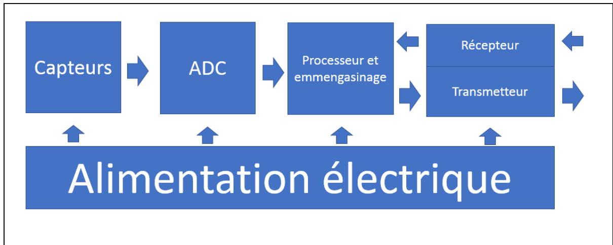
Figure 3.3 Architecture physique du système d'acquisition
