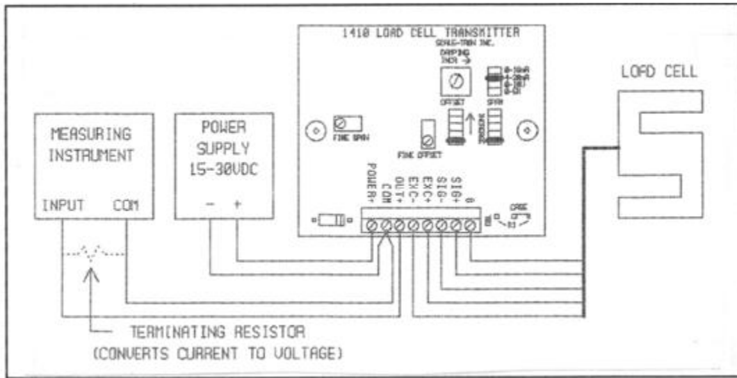
Figure 5.13 Diagramme de connexion pour un ADC et amplificateur ( http://www.vishaypg.com/load-cells/ )
