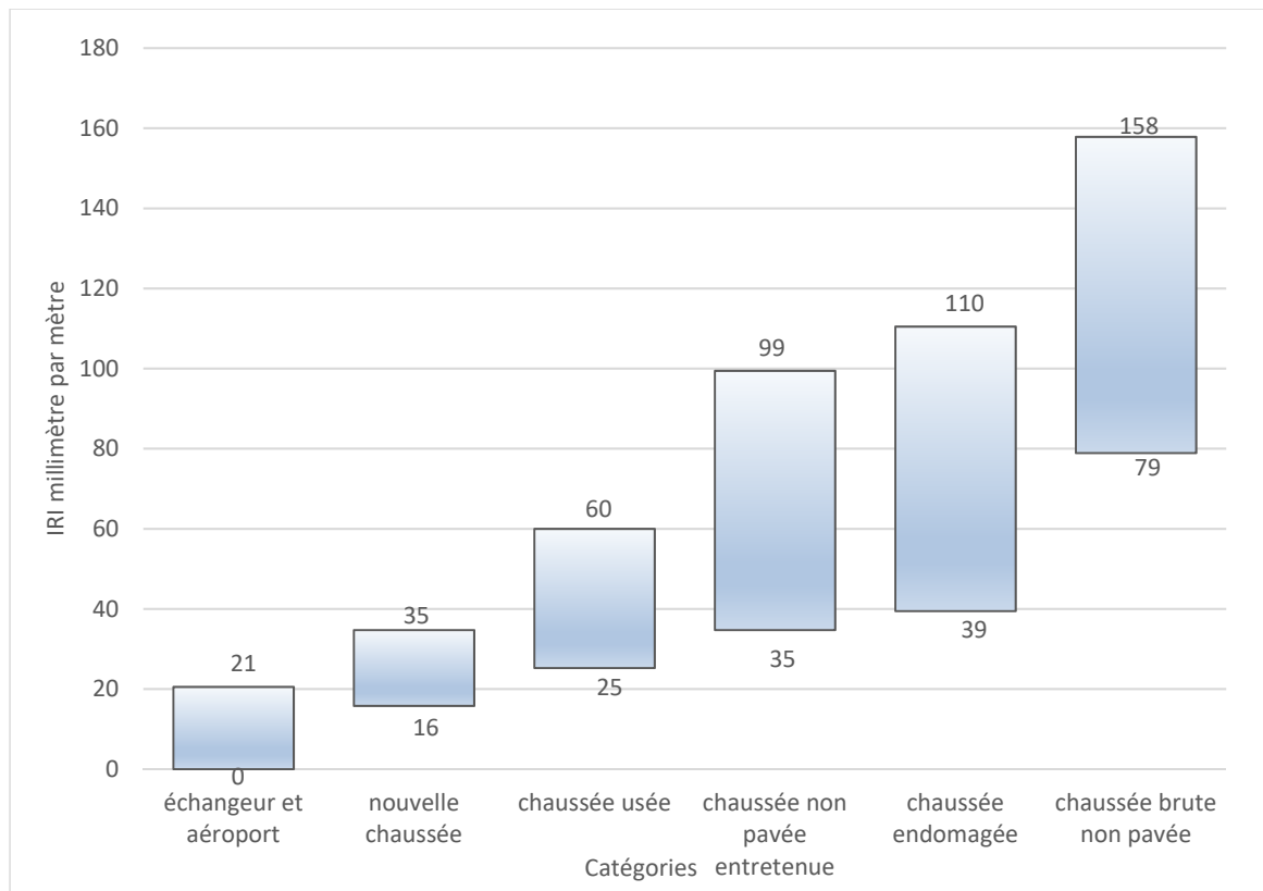
Figure 2.3 Échelle d'indice de rugosité (Sayers et al. 1986)
