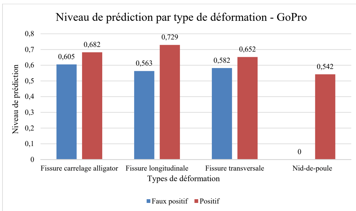
Figure 6.6 Niveau de prédiction par type de déformation - GoPro
