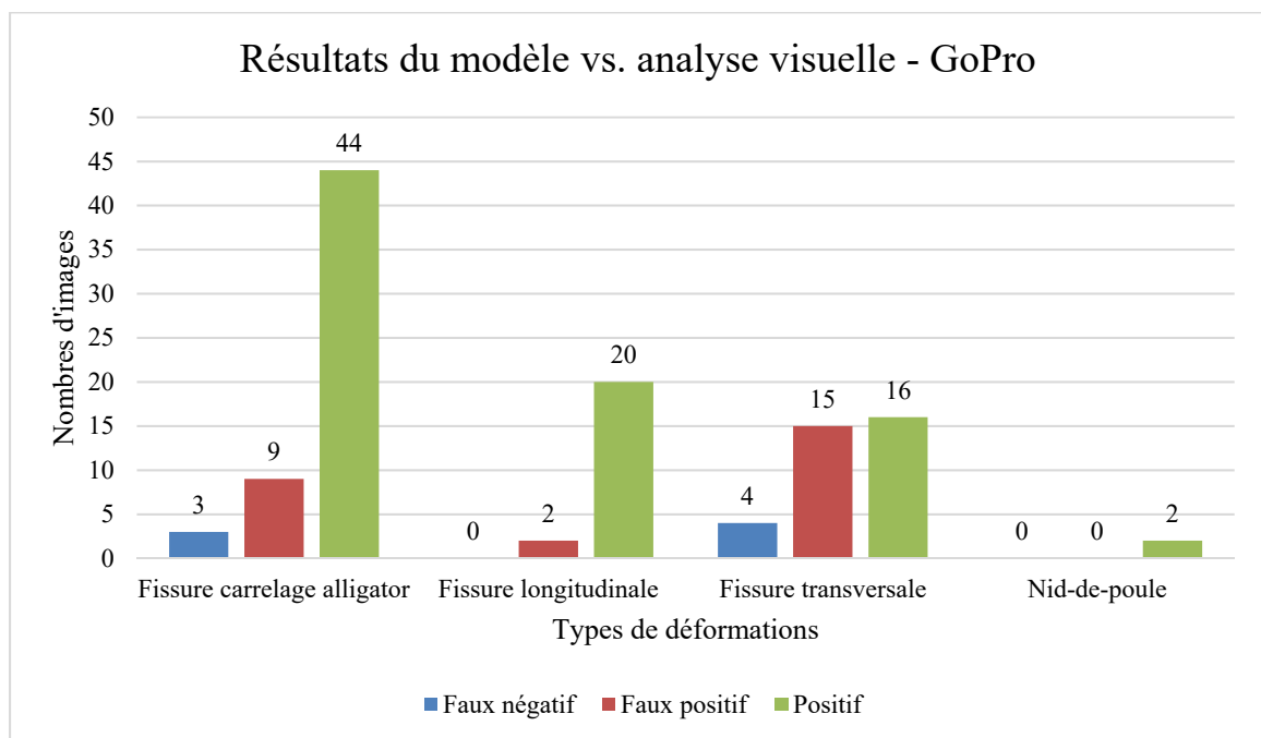
Figure 6.5 Résultats du modèle vs. analyse visuelle – GoPro
