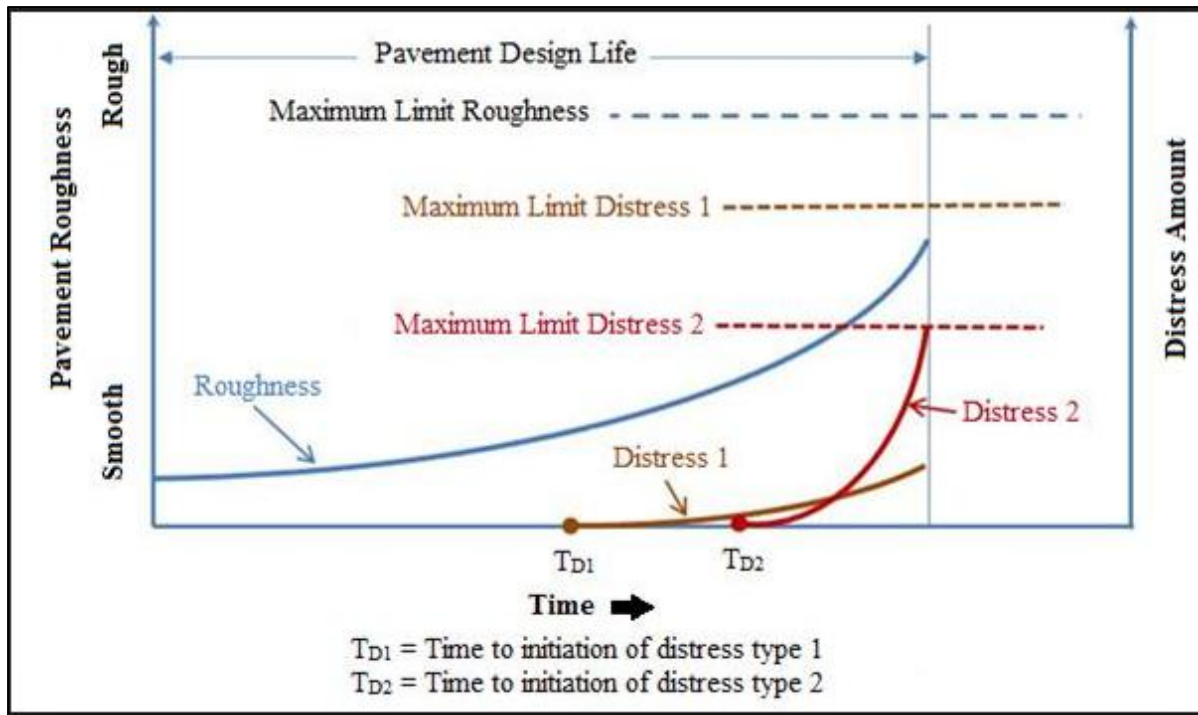
Figure 2.6 Exemple de multi dommages subis par la route (FHWA, 2001)
