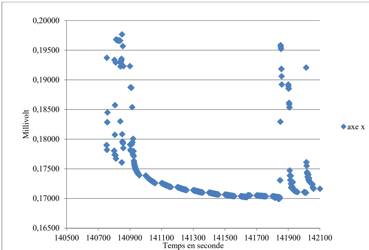
Figure 5.30 Acquisition des données dynamiques sur le capteur nommé x (Les résultats de la charge de 78.45 kN sont mV sur l'axe des y et le temps en seconde sur l'axe des x)
