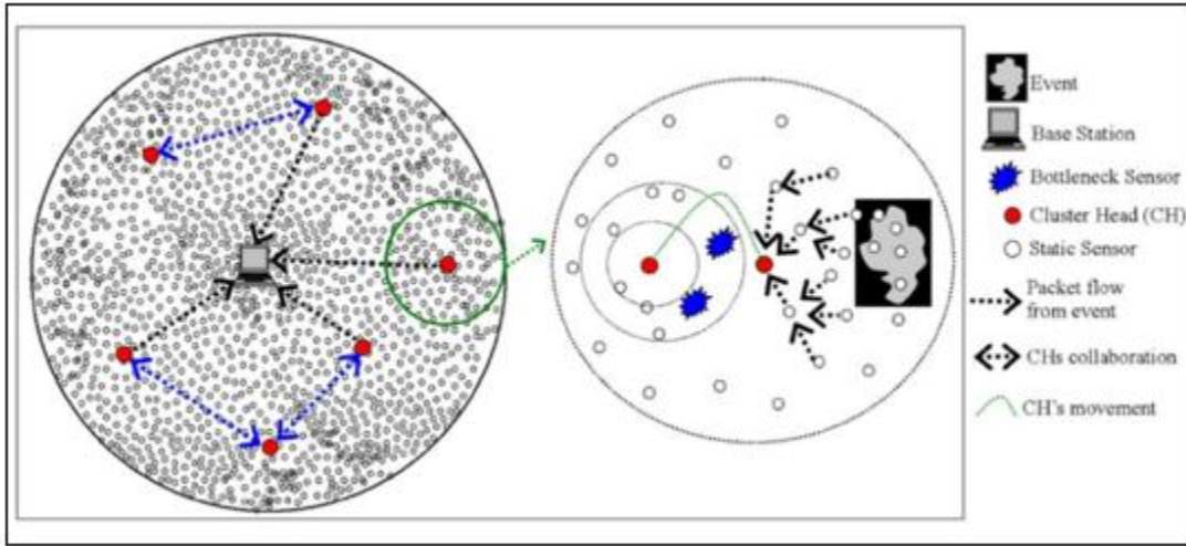
Figure 3.4 Mode de mobilité à plusieurs têtes de grappes (Khan, 2014)
