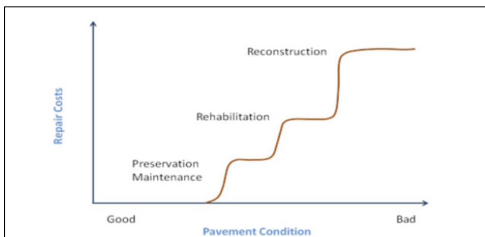
Figure 2.5 PCI, relation entre les coûts et les conditions de la route (FHWA, 2013)
