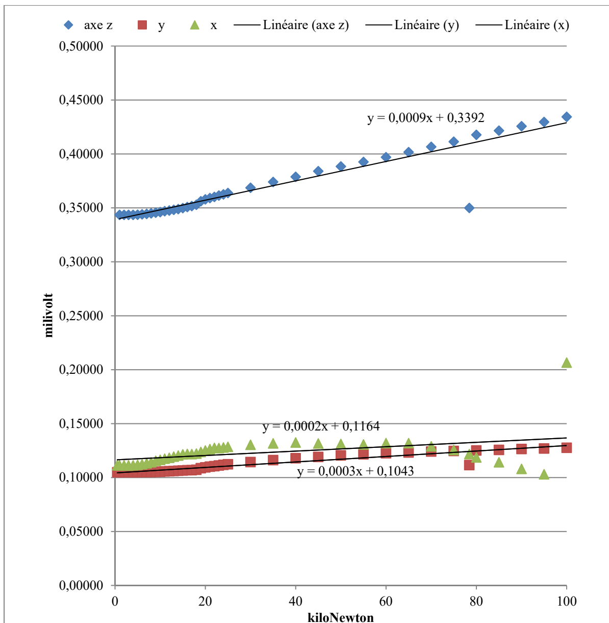
Figure 5.31 Régression linéaire avec données originales
