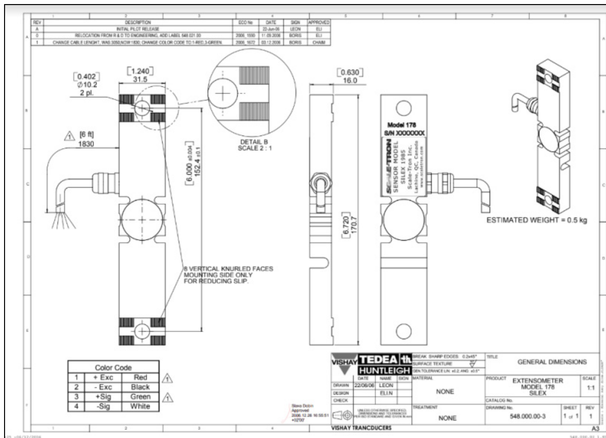
Figure 5.12 Extensomètre de Vishay ( http://www.vishay.com/search?query=extensometer&searchChoice=part )
