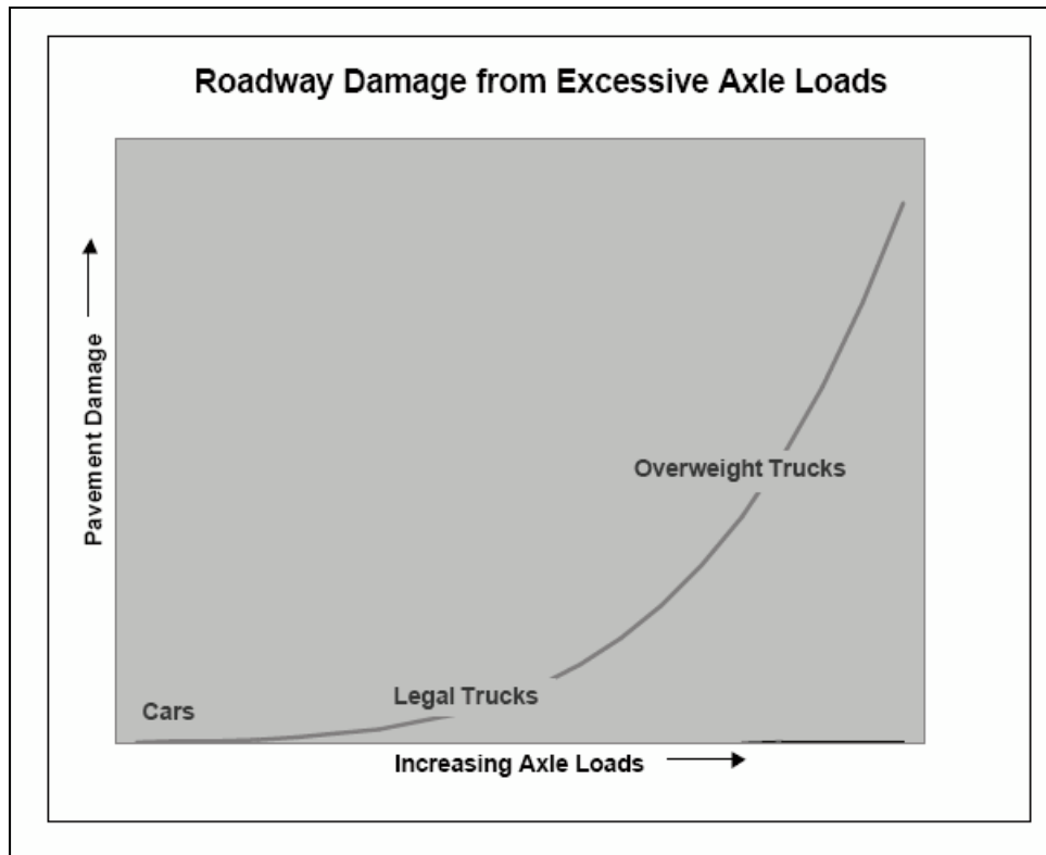
Figure 3.29 Augmentation des dommages de la chaussée via la charge de l'essieu, puissance n (4-5) (Santero, 2005)
