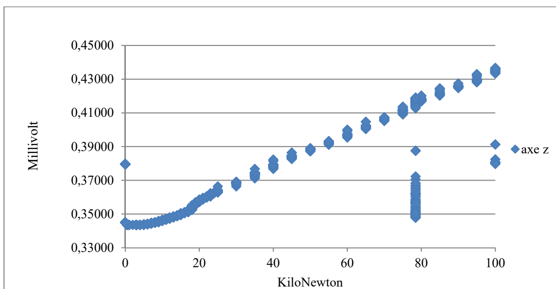
Figure 5.29 Acquisition statique des données sur le capteur nommé Z (Les résultats sont mV sur l'axe des y et kN sur l'axe des x)
