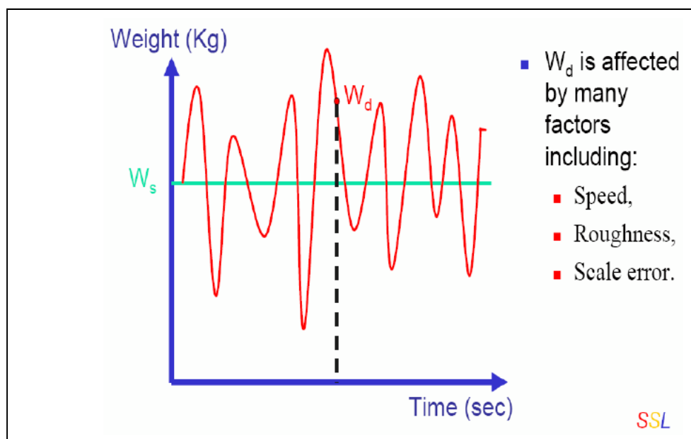
Figure 3.27 Évaluation du poids statique et dynamique (IRD, 2001)
