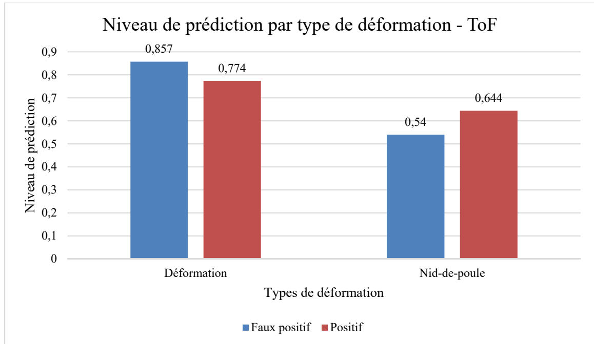
Figure 6.3 Niveau de prédiction par type de déformation - ToF
