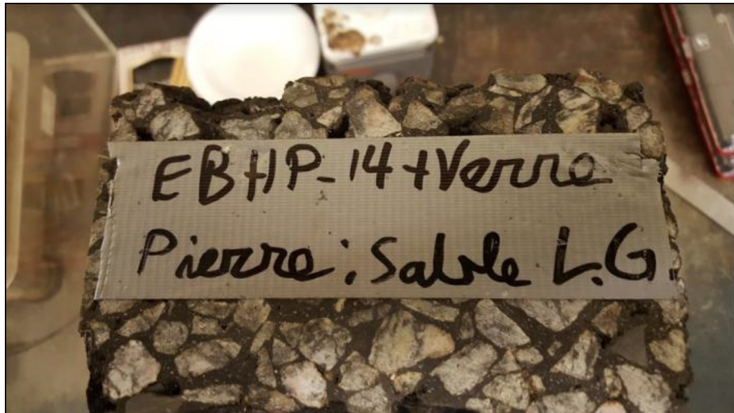
Figure 5.10 Enrobé bitumineux haute performance de l'expérimentation
