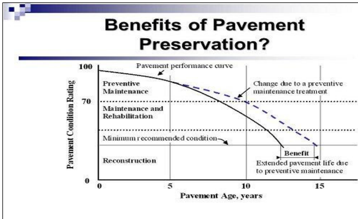
Figure 2.1 Bénéfice de la préservation (AASHTO, 2009)
