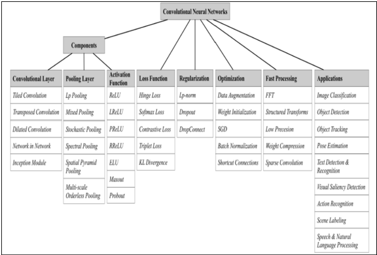
Figure 3.14 Réseau de neurones convolutif (Gu, 2018)
