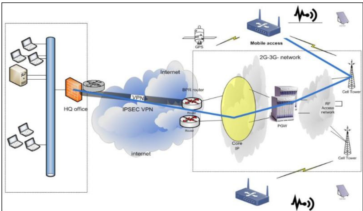
Figure 5.15 Architecture réseau cellulaire
