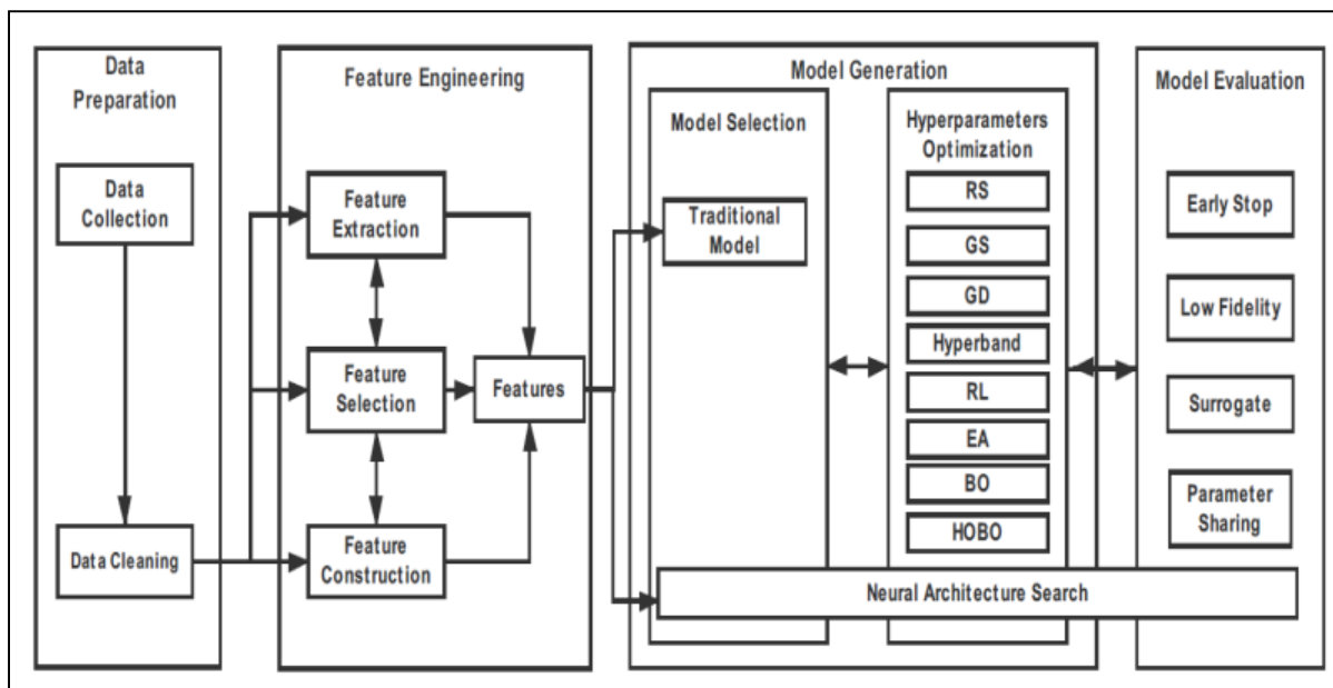
Figure 4.1 Vision globale pour l'AutoML pour la génération des données (He, 2019)
