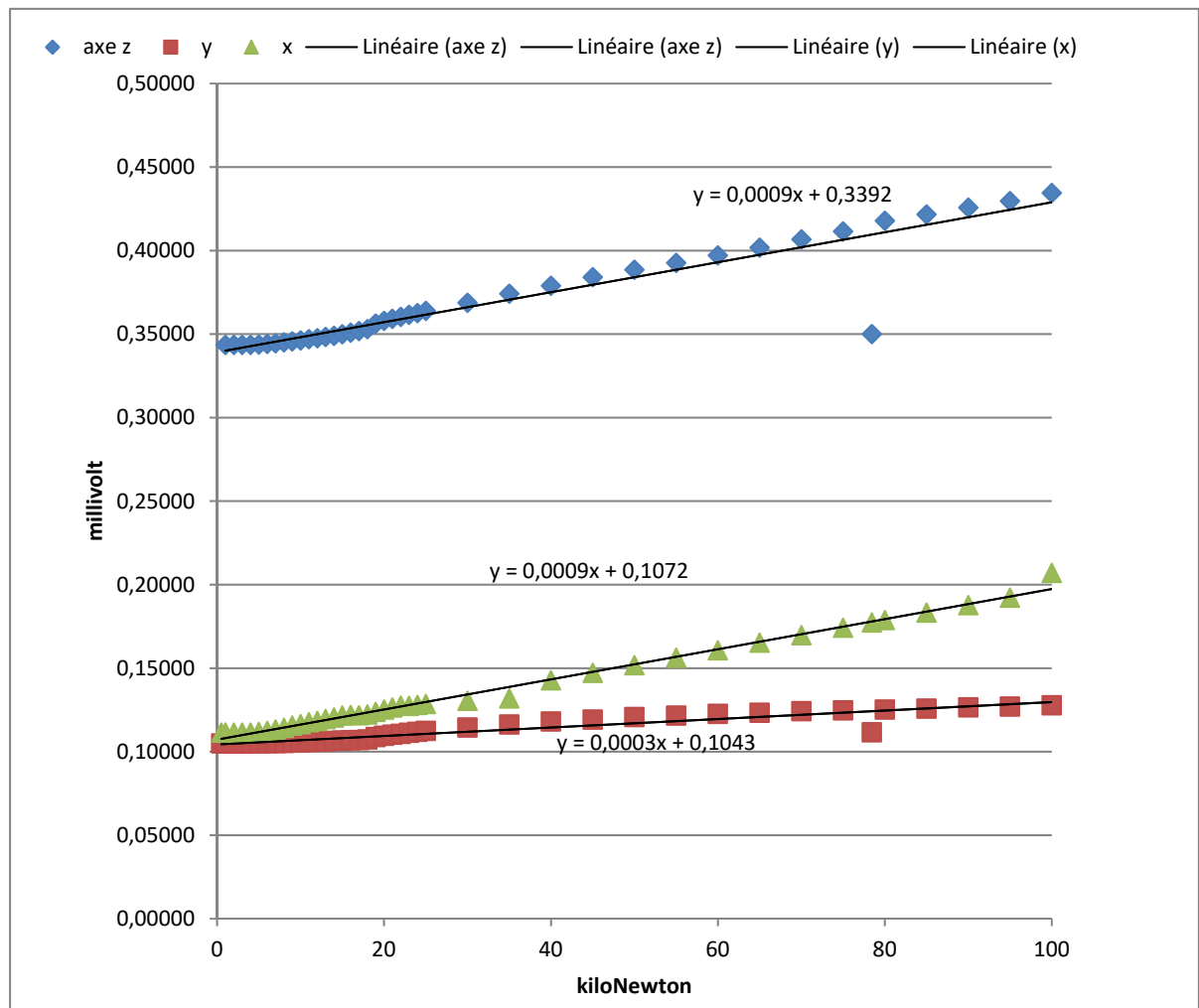
Figure 5.32 Régression linéaire avec valeur des x corrigée qui donne l'équation y = 0.0009x + 0.1072
