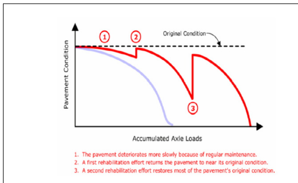
Figure 3.28 Cycle de vie de la chaussée avec maintenance (WAPA, 2002)
