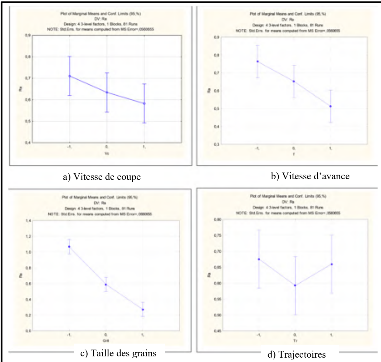
Figure 4-10: Influence des facteurs principaux sur Ra
