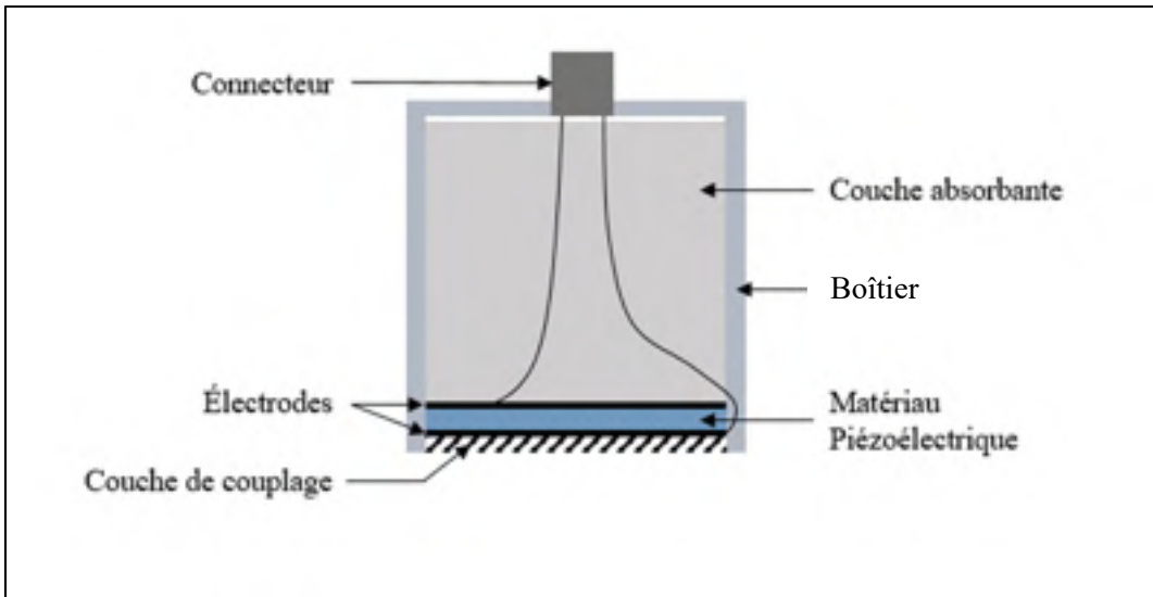
Figure 1.9 Schéma d'un transducteur piézoélectrique
