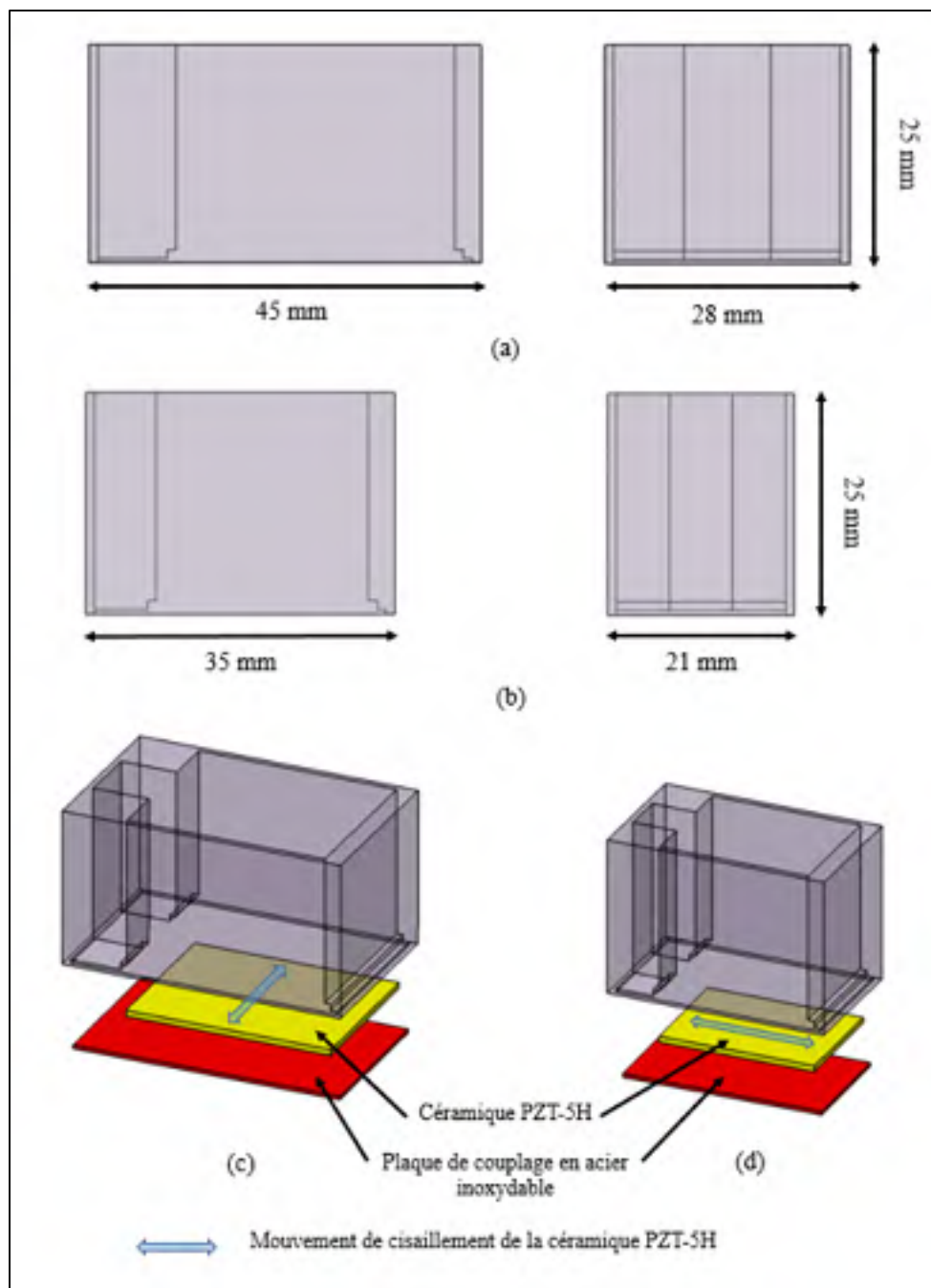
Figure 3.3 Dimensions des boîtiers ABS et composants des transducteurs piézoélectriques. (a) Dimensions du boîtier S_0 centré à 100 kHz, (b) Dimensions du boîtier SH_0 centré à 90 kHz, (c) Vue éclatée du transducteur S_0 , (d) Vue éclatée du transducteur SH_0
