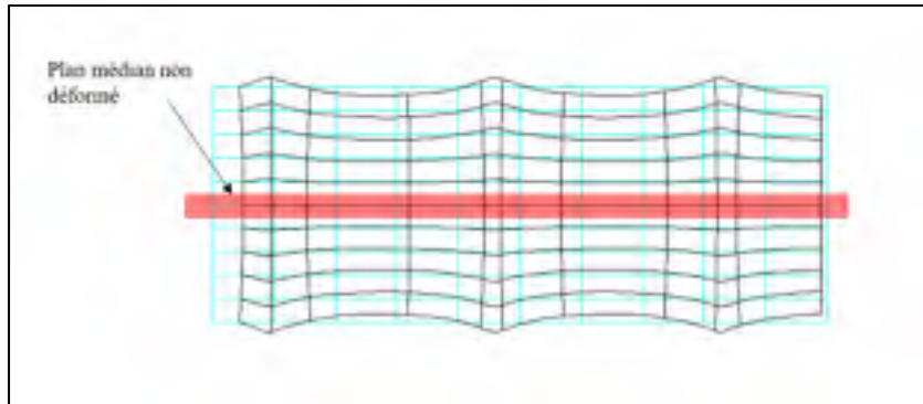
Figure 2.10 Forme du mode d'onde S_0 pour une plaque d'acier de 12.7 mm d'épaisseur. Obtenu avec DISPERSSE (Pavlakovic et al., 1997)
