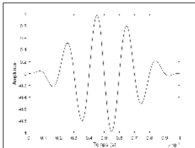
Figure 2.3 Signal d'excitation de 5 cycles centré à 50 kHz avec fenêtré de Hann
